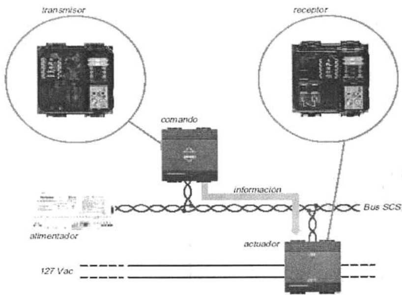
Figura. Configuración de los dispositivos, comandos y actuadores.
