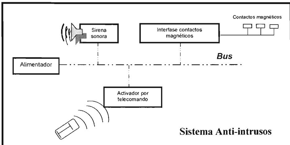
Fig. 4.1. Esquema del sistema anti-intrusos
