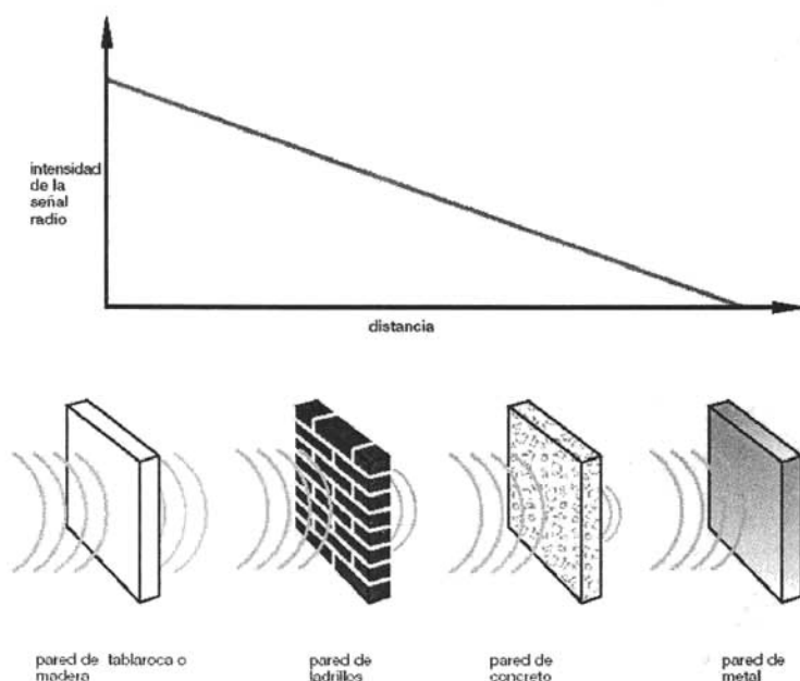
Fig. 2.1.3 Atenuación de la señal
