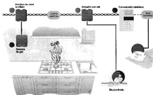
Figura 3.3.1.- Detección de fuga de gas con sistema antirrobo y detector de gas.
