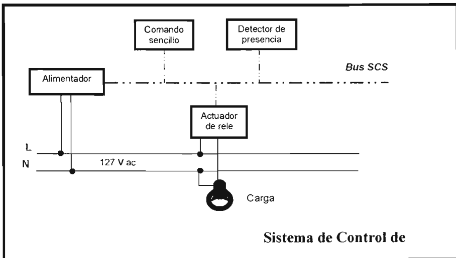
Fig. 4.2 Esquema del sistema de Control de iluminación
