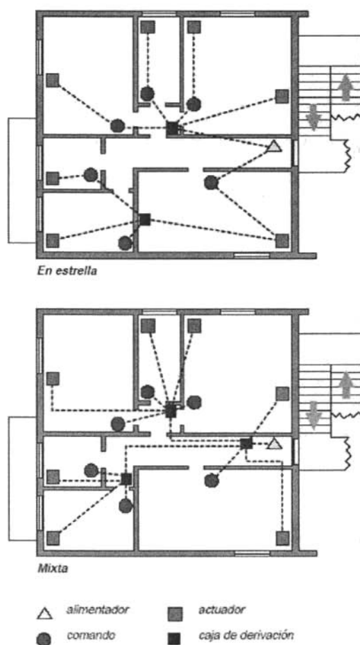
Ejemplo de distribución BUS y energía en una casa-habitación
