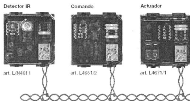
Fig. Configuración de detectores IR pasivos
