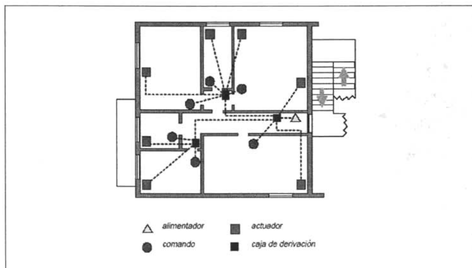
Fig. 4.1.1 Unidad habitacional
