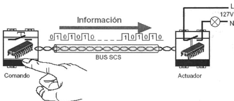
Fig.2.1.1 Sistema SCS
