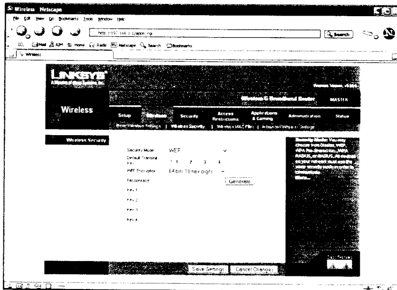
Configuración de la Seguridad de la Red Inalámbrica
