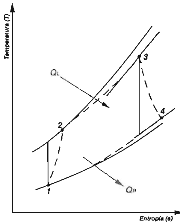
Figura 3.2.2. Diagrama T-s del ciclo termodinámico básico real de las turbinas de gas.
