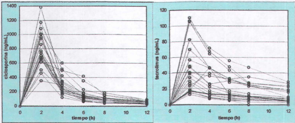
Figura 3 Perfiles farmacocinéticos
