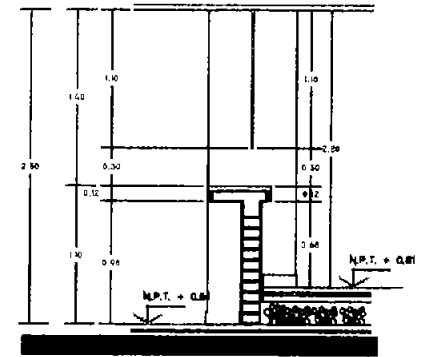
Corte F - F'
