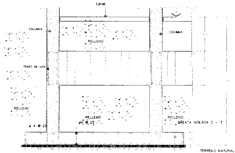
Corte J-J'
