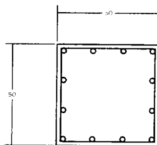
Columna C-2
