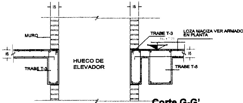
Corte G-G'
