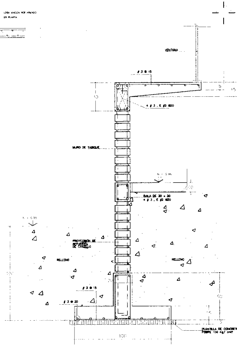
Detalle 1
