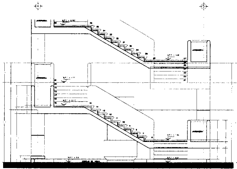
Corte longitudinal
