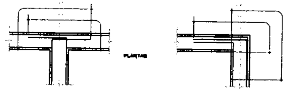
Anclajes extremos (para varillas corridas y bastones)
