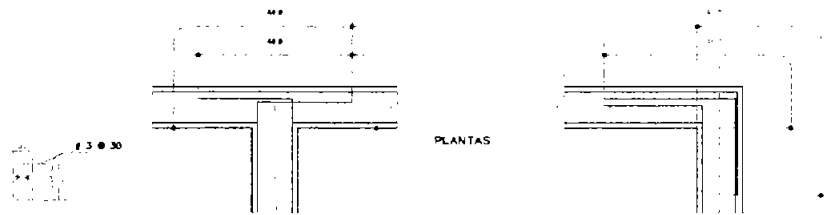
Anclajes extremos (para varillas corridas y bastones)
