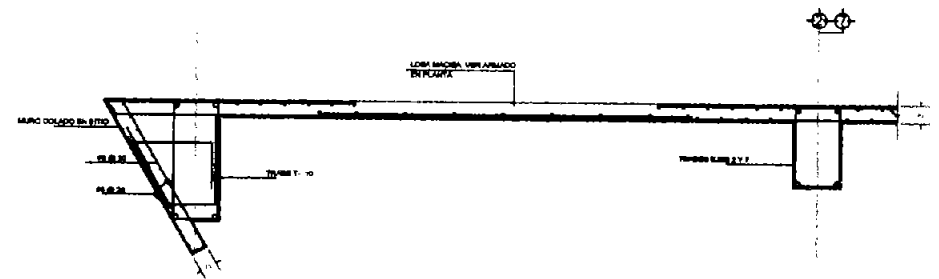
Corte B-B'
