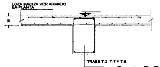
Corte D-D'
