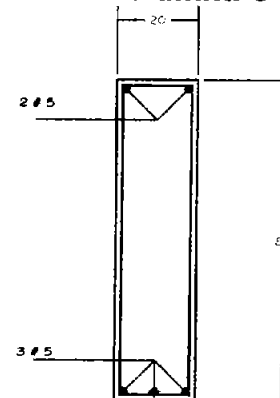
Trabe de liga E # 3 @ 15
