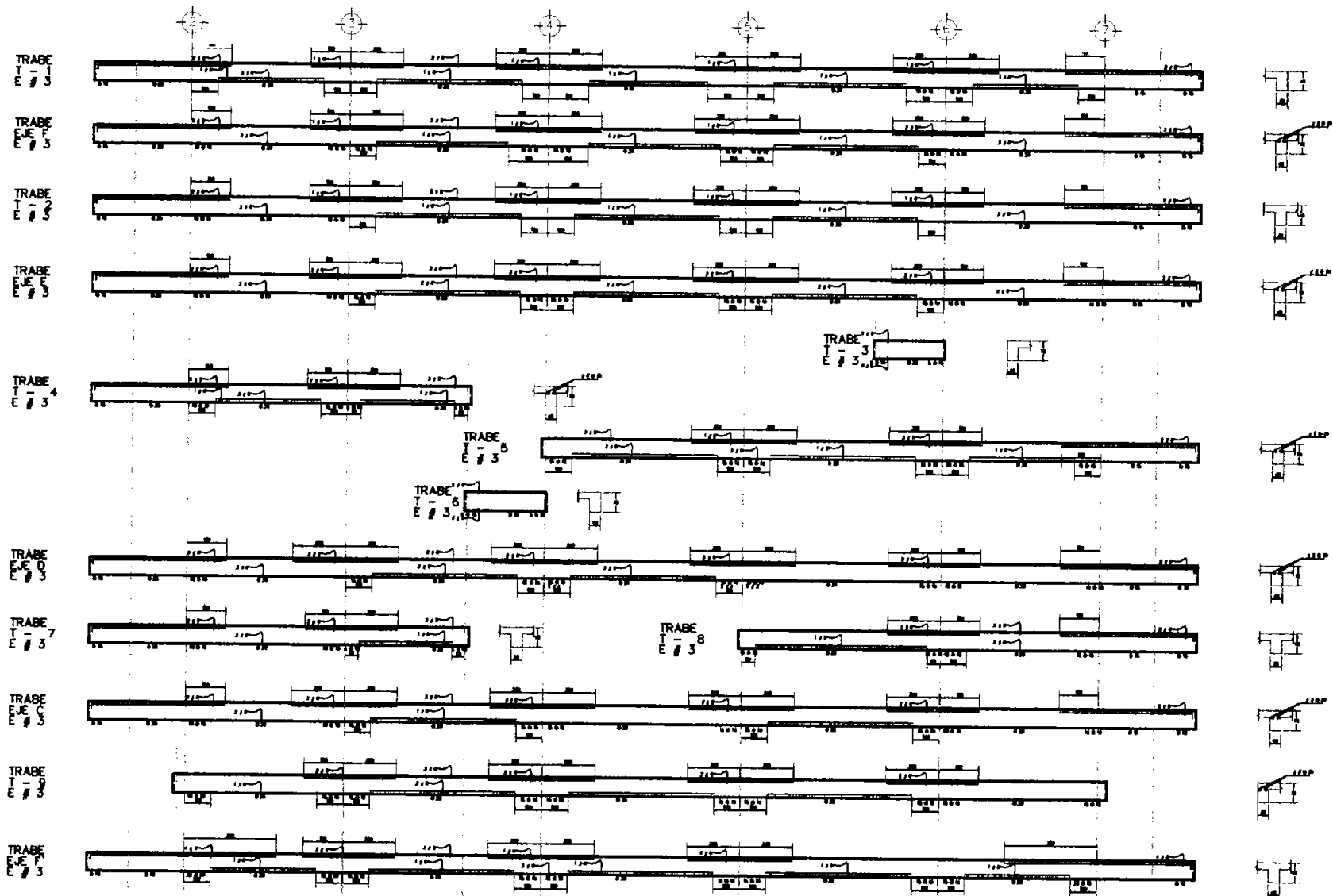
Detalle de traves corte y planta
