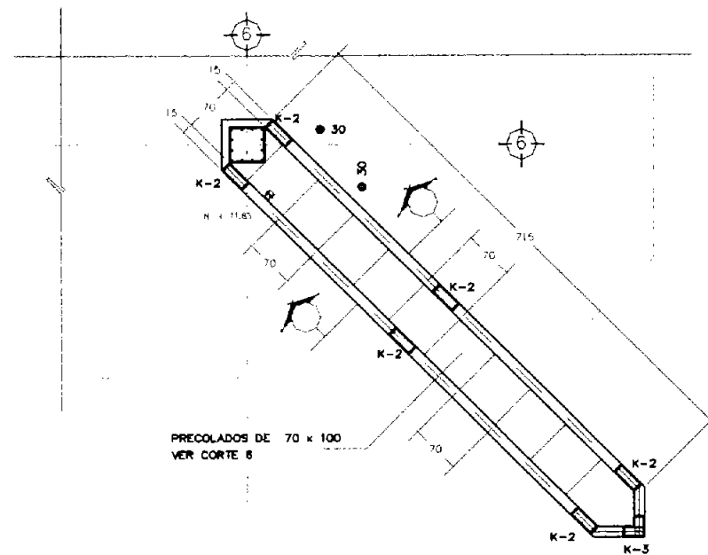
Planta parcial de azotea
