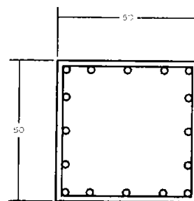
Columna C-3
