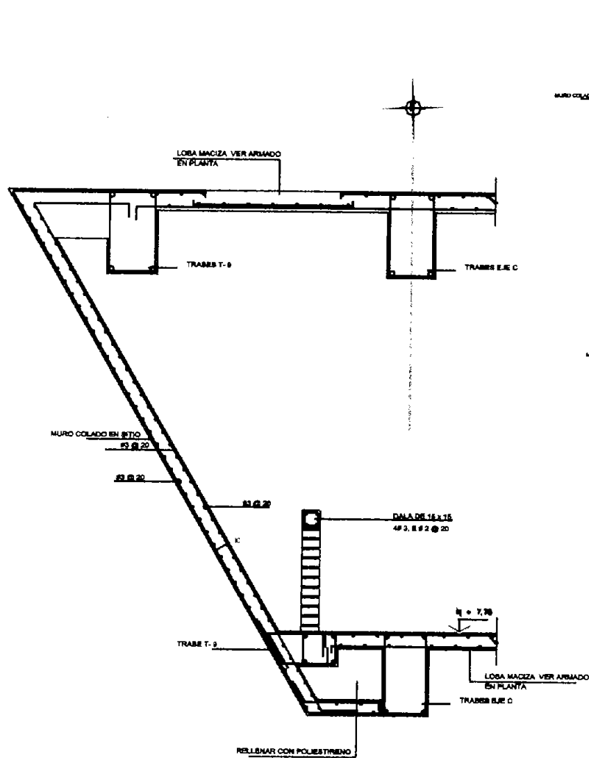
Corte A-A'
