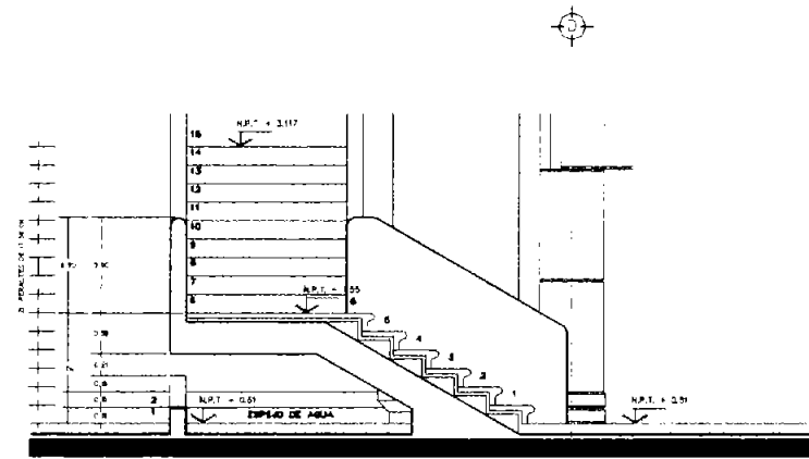
Corte transversal
