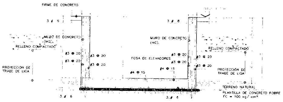
Corte H-H'
