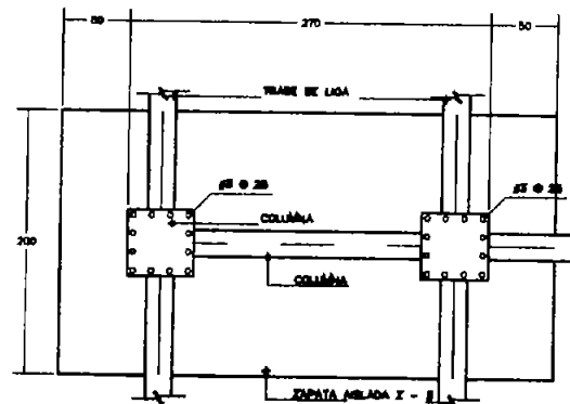
Zapata aislada Z-1
