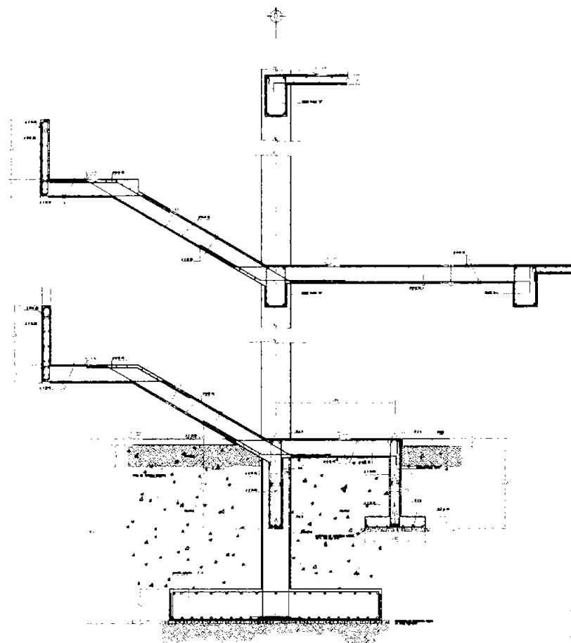
Corte C-C'
