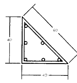
Columna C-5
