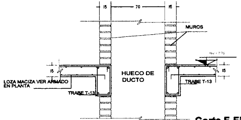
Corte F-F'
