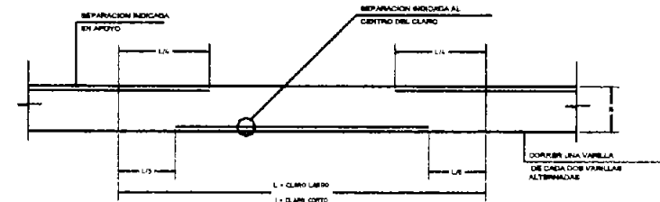
Corte tipo de losa maciza
