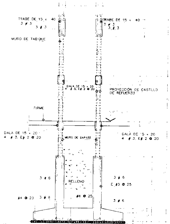
Corte F-F'
