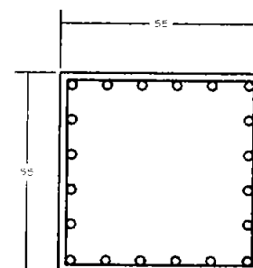
Columna C-4
