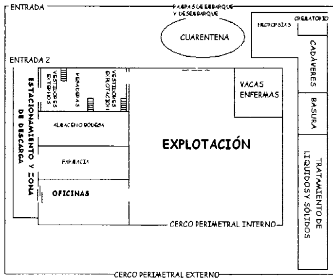
Figura 8. Croquis de la explotación.
