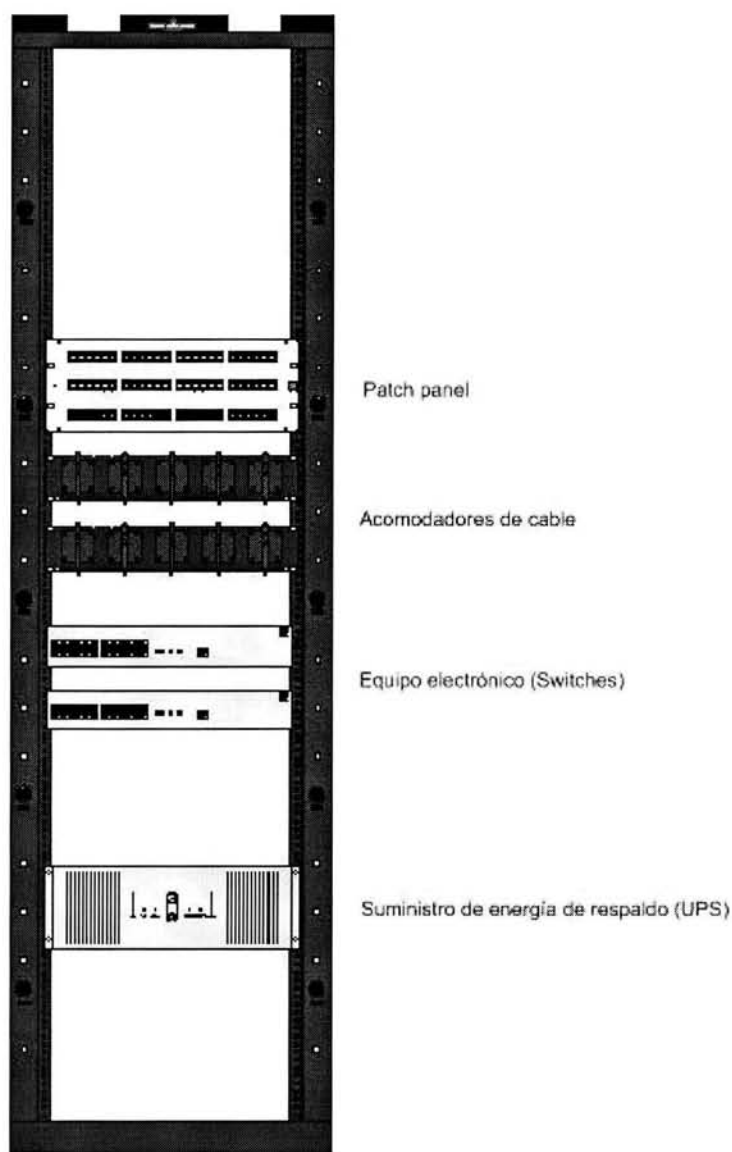
Figura 3-4. Disposición de equipo dentro del rack.
