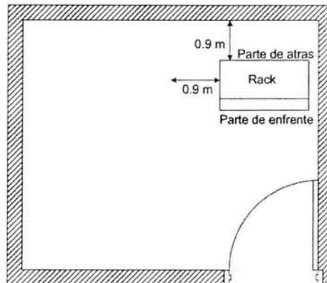
Figura 3-3. Vista superior del rack en el Closet de Telecomunicaciones.
