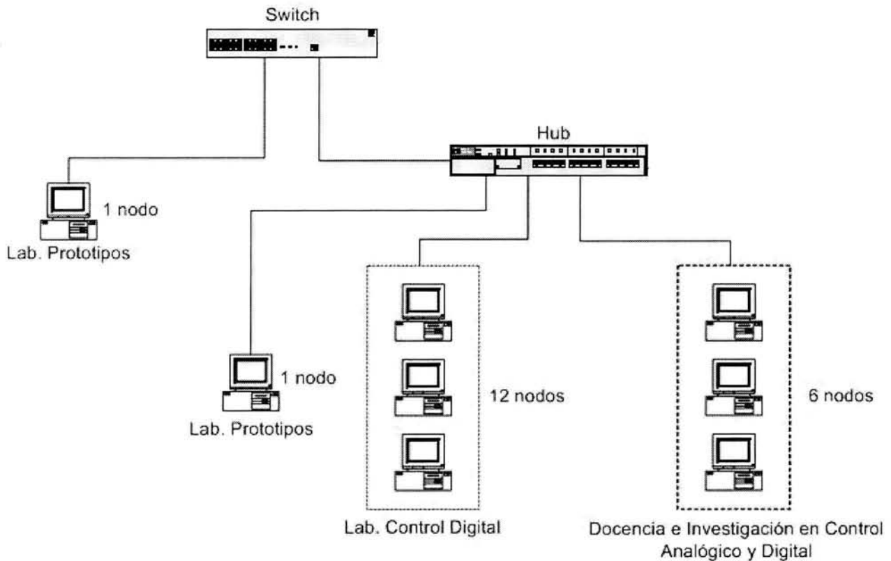
Figura 3-1. Diagrama de red del primer piso.
