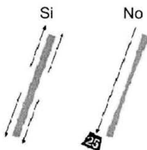
Figura 3-9. No estirar excesivamente el cable.
