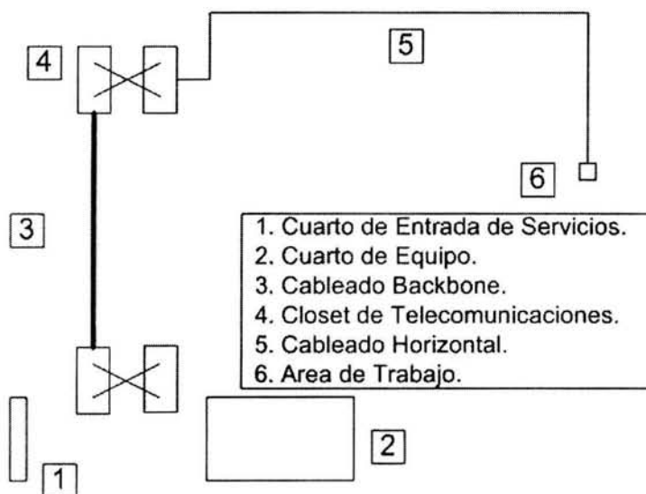
Figura 2-9. Subsistemas de Cableado Estructurado.
