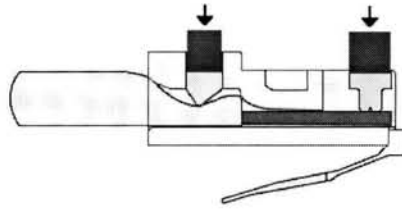
Figura 3-15. Fijación de cable UTP a plug RJ-45.
