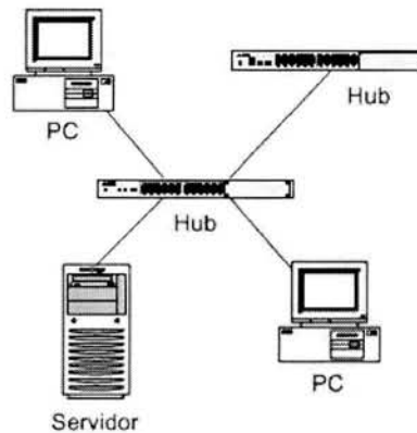
Figura 2-11. Configuración en estrella utilizando un concentrador.
