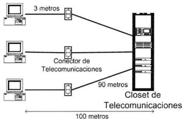
Figura 2-6. Distancias máximas para cableado horizontal.
