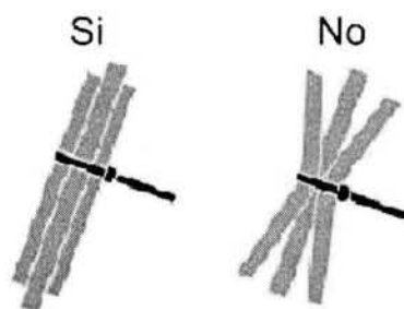
Figura 3-10. No apretar excesivamente los cables.
