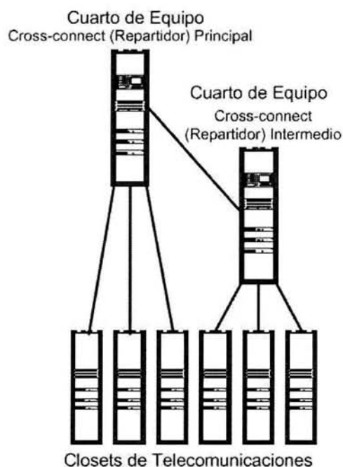
Figura 2-5. Nivel jerárquico del cableado backbone.
