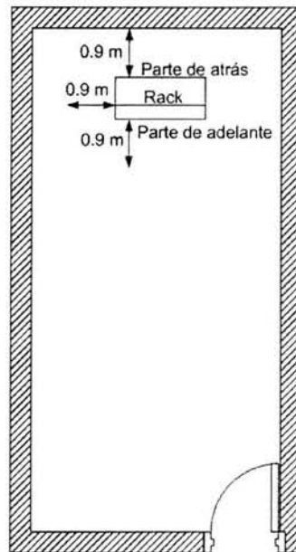
Figura 3-5. Vista superior del rack en el Closet de Telecomunicaciones.
