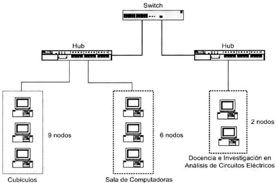
Figura 3-2. Diagrama de red del segundo piso.
