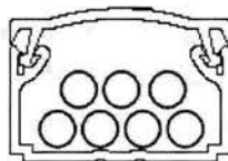
Figura 3-6. Sección transversal de canaleta llenada al 40% de su capacidad.
