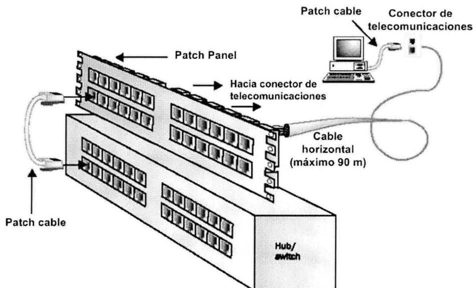
Figura 2-10. Componentes típicos de un esquema de cableado estructurado.
