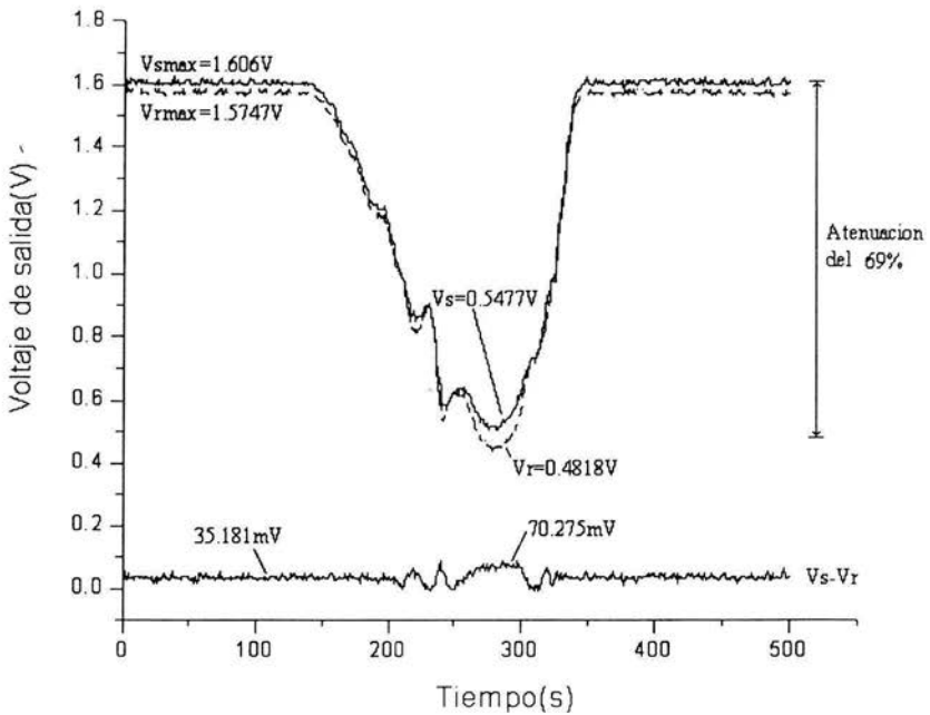
Figura 4.3.9 Monitoreo de la señal de salida cuando se aplica una curvatura de aproximadamente 5mm de diámetro.
