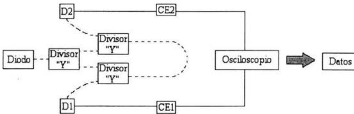
Figura 4.2.2 Primera configuración para monitorear las señales. Donde la línea punteada representa fibra óptica y la línea continua cable eléctrico
