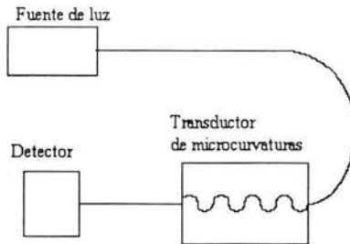
Figura 2.3.7 Los sensores de microcurvaturas en fibra óptica
