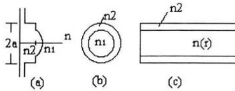
Figura 1.3.2 Fibra de índice gradual. (a) Perfil del índice de refracción. (b) Vista del extremo. (c) Vista transversal.
