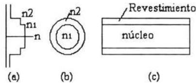
Figura 1.3.1 Fibra de índice escalonado. (a) Perfil del índice de refracción. (b) Vista del extremo. (c) Vista transversal.
