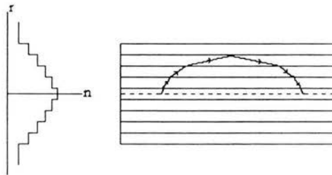
Figura 1.3.4 Modelo escalonado de una fibra óptica de índice gradual
