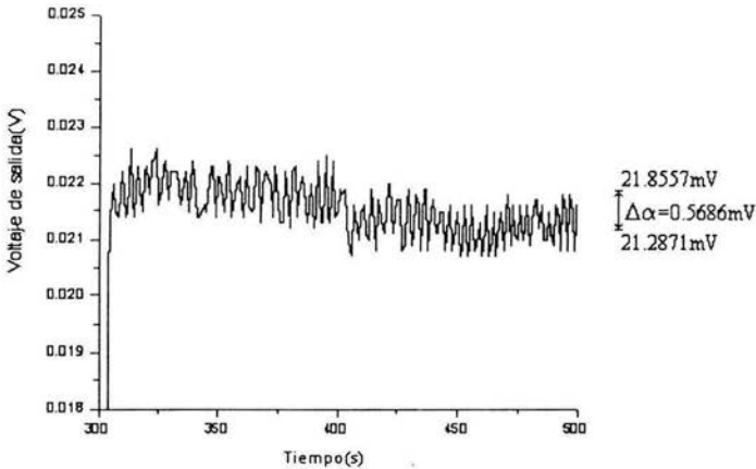
Figura 4.3.4 Ampliación de la zona donde se realiza el decremento de potencia
