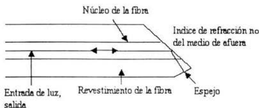
Figura 2.3.5 Sensor usando las propiedades del ángulo crítico de una fibra óptica o índice de refracción.
