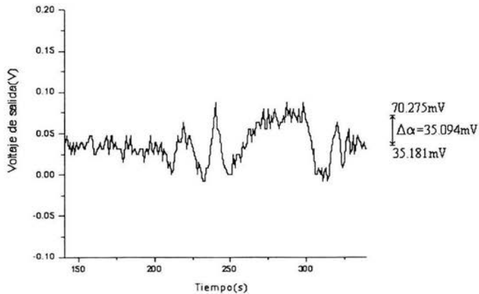
Figura 4.3.10 Ampliación de la gráfica (3.3.9) en intervalo donde se aplica la microcurvatura
