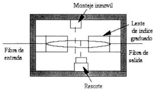
Figura 2.3.8 Sensor de vibración o aceleración utilizando rejillas.
