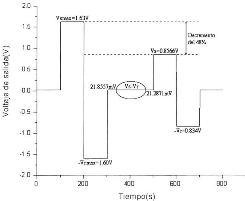
Figura 4.3.3 Monitoreo de la señal de salida cuando se realiza un decremento de potencia.
