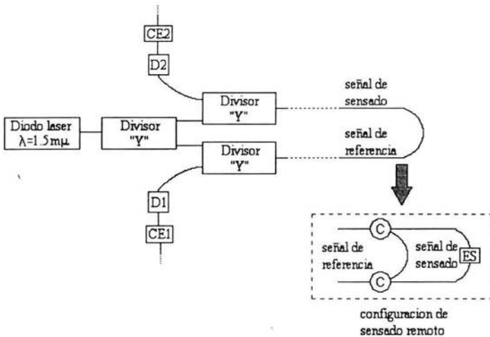
Figura 4.2.1 Esquema del arreglo experimental del sistema de referencia.
