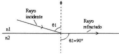
Figura 1.1.3 Refracción en el ángulo crítico, n_1 > n_2 y \theta_1 < \theta_c , porque \theta_2 = 90^\circ y \theta_1 = \theta_c .
