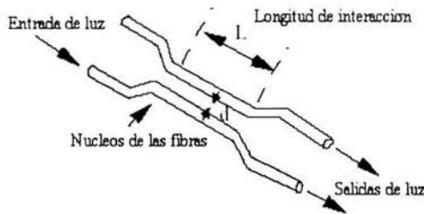
Figura 2.3.6 Sensor basado en el inter-acoplamiento de luz entre dos núcleos ubicados a proximidad.
