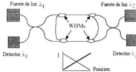
Figura 2.2.2 Sensor acústico distribuido basado en anillos de Sagnac entrelazados
