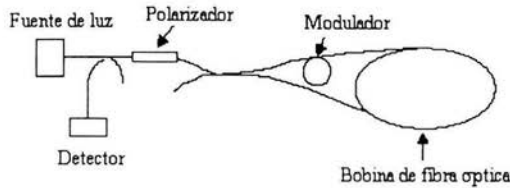
Figura 2.2.1 Los girocompases de fibra óptica de anillo abierto son sensores de rotación más simples y de más bajo costo
