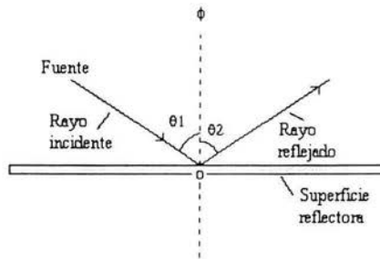
Figura 1.1.1 Ley de la reflexión: \theta_1 -ángulo de incidencia, \theta_2 -ángulo de reflexión, \phi -perpendicular a la superficie
