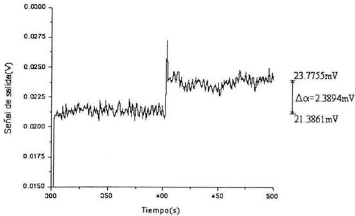
Figura 4.3.2 Ampliación de la figura (3.3.1) en la zona donde se realiza el incremento de potencia de la señal de entrada
