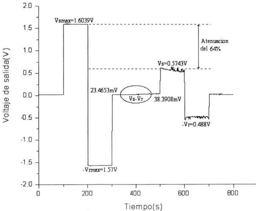
Figura 4.3.7 Monitoreo de la señal de salida ( S out ) cuando se aplica una curvatura de diámetro aproximado de 3cm
