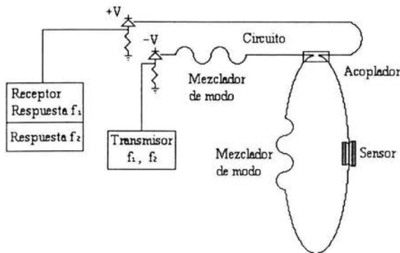
Figura (3.2) Concepto de un sistema sensor con modulación Q, usando un anillo resonador.
