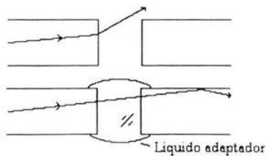
Figura 1.2.3 Un fluido adaptador de índice disminuye las pérdidas por separación de fibras reduciendo la divergencia del haz.
