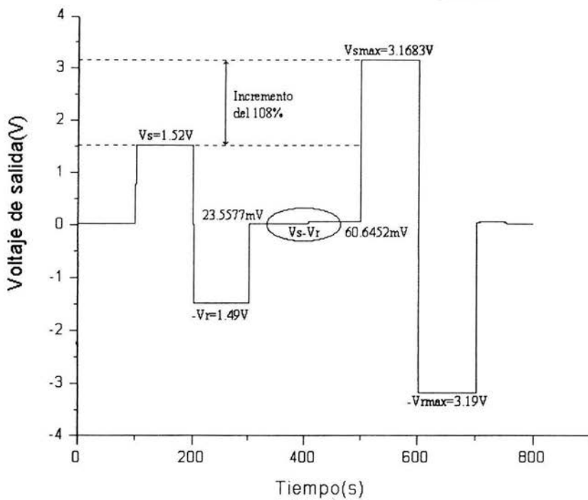
Figura 4.3.5 Monitoreo de la señal de salida cuando se incrementa la potencia y los detectores han sido invertidos en el lazo común.
