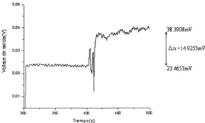
Figura 3.3.8: Ampliación de la gráfica (3.3.7) cuando se aplica una curvatura de 3cm de diámetro
