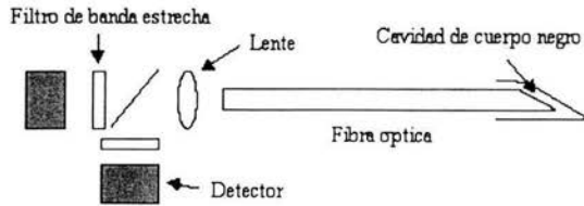
Figura 2.1.1. Sensor que permite la medida de temperatura y es más efectivo en temperaturas de más de 300°
