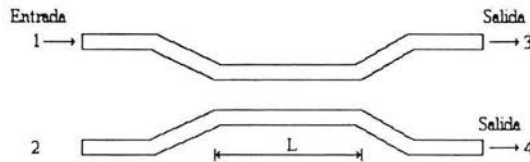
Figura 1.4.1 Acoplador direccional.
