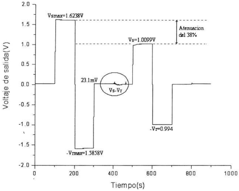
Figura 4.3.11 Monitoreo de la señal de salida cuando se aplica una curvatura de diámetro de 3cm y la fibra se mueve del plano original.
