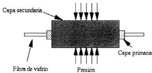
Figura 2.2.3 Las capas pueden ser usadas para optimizar la sensibilidad del sensor
