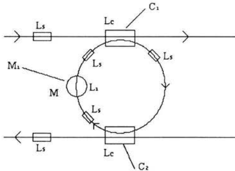
Figura 3.1 Esquema del anillo sensor autoreferenciado
