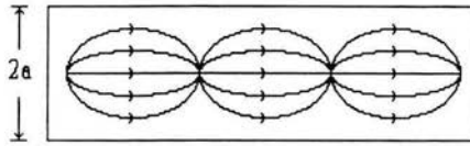
Figura 1.3.3 Trayectorias de los rayos de luz a lo largo de una fibra óptica de índice gradual
