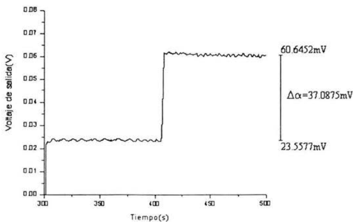
Figura 4.3.6 Ampliación de la zona a analizar cuando la potencia se incremento en un 108%
