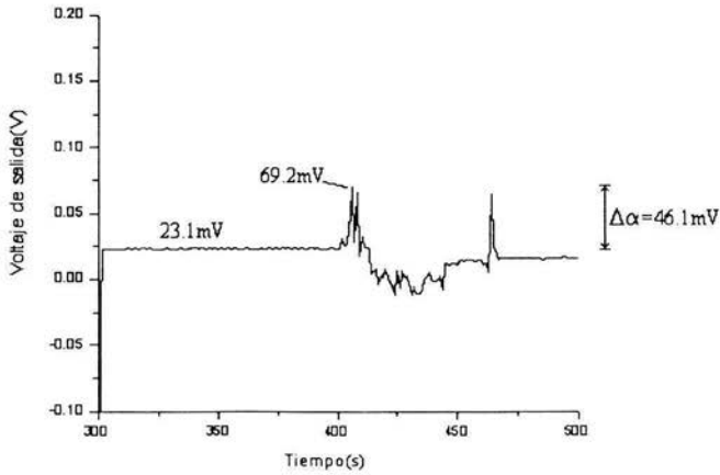
Figura 4.3.12 Ampliación del intervalo donde se realiza la curvatura
