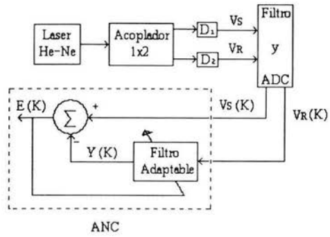
Figura (3.3) Diagrama esquemático de un sistema sensor experimental
