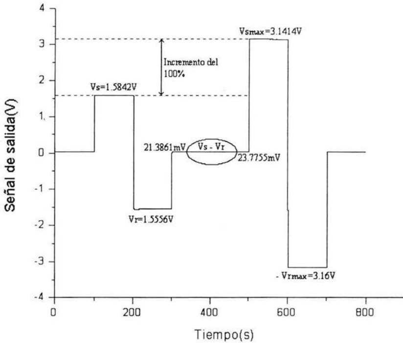
Figura 4.3.1 Monitoreo de la señal de salida ( S_{out} ) cuando se realiza un incremento de potencia de la señal de entrada del 100%
