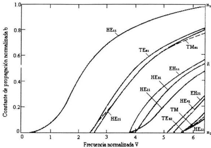
Figura 1.1.5 Constante de propagación b como función de la frecuencia normalizada V para modos de bajo orden. La escala de la derecha muestra el índice de modo n .
