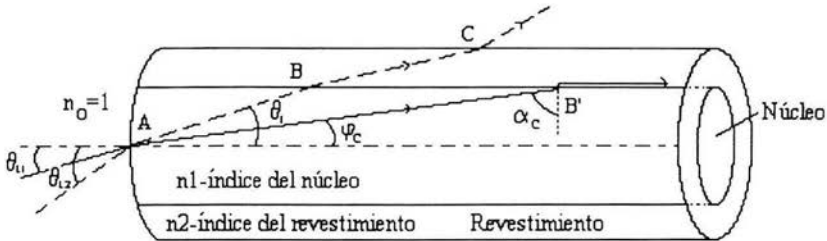
Figura 1.1.4 Propagación de luz en una fibra de índice escalonado.
