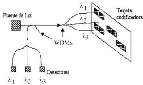
Figura 2.3.3 Sensor de posición usando la técnica de multiplexado en longitud de onda.
