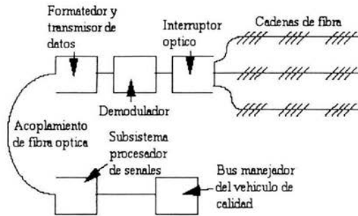
Figura 2.4.3 Arquitectura modular para un gran sistema de estructura inteligente que consistiría de cadenas de sensores accesible vía un interruptor óptico y un sistema demodulador.
