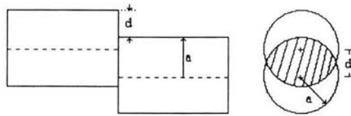
Figura 1.2.1 Corrimiento de los núcleos de las fibras transmisora y receptora. Los núcleos están desalineados por la distancia d .
