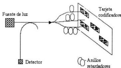
Figura 2.3.4 Sensor de posición lineal usando multiplexado por división de tiempo.
