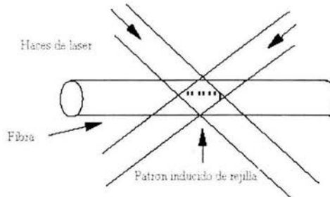
Figura 2.1.2 Sensor de fibra óptica de rejilla
