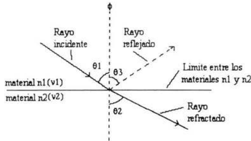
Figura 1.1.2 Reflexión y refracción: \theta_1 -ángulo de incidencia, \theta_2 -ángulo de refracción, \theta_3 -ángulo de reflexión y n_1 > n_2
