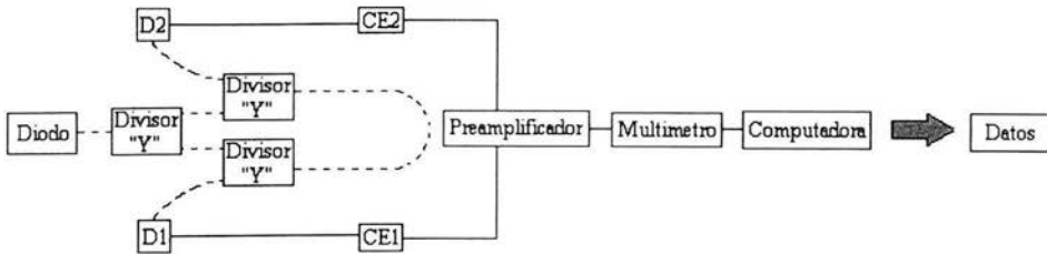
Figura 4.2.3 Segunda configuración para monitorear. Donde la línea punteada representa fibra óptica y la línea continua cable eléctrico
