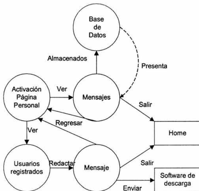
Figura 3.4. Nivel 2 del Diagrama de Flujo de Datos
