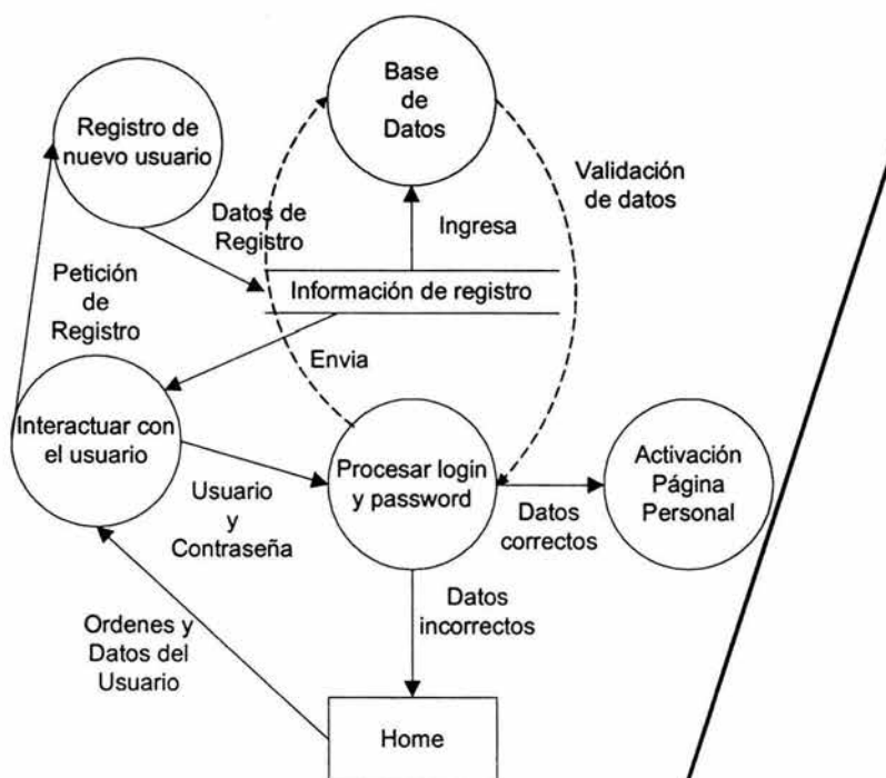
Figura 3.3. Nivel 2 del Diagrama de Flujo de Datos
