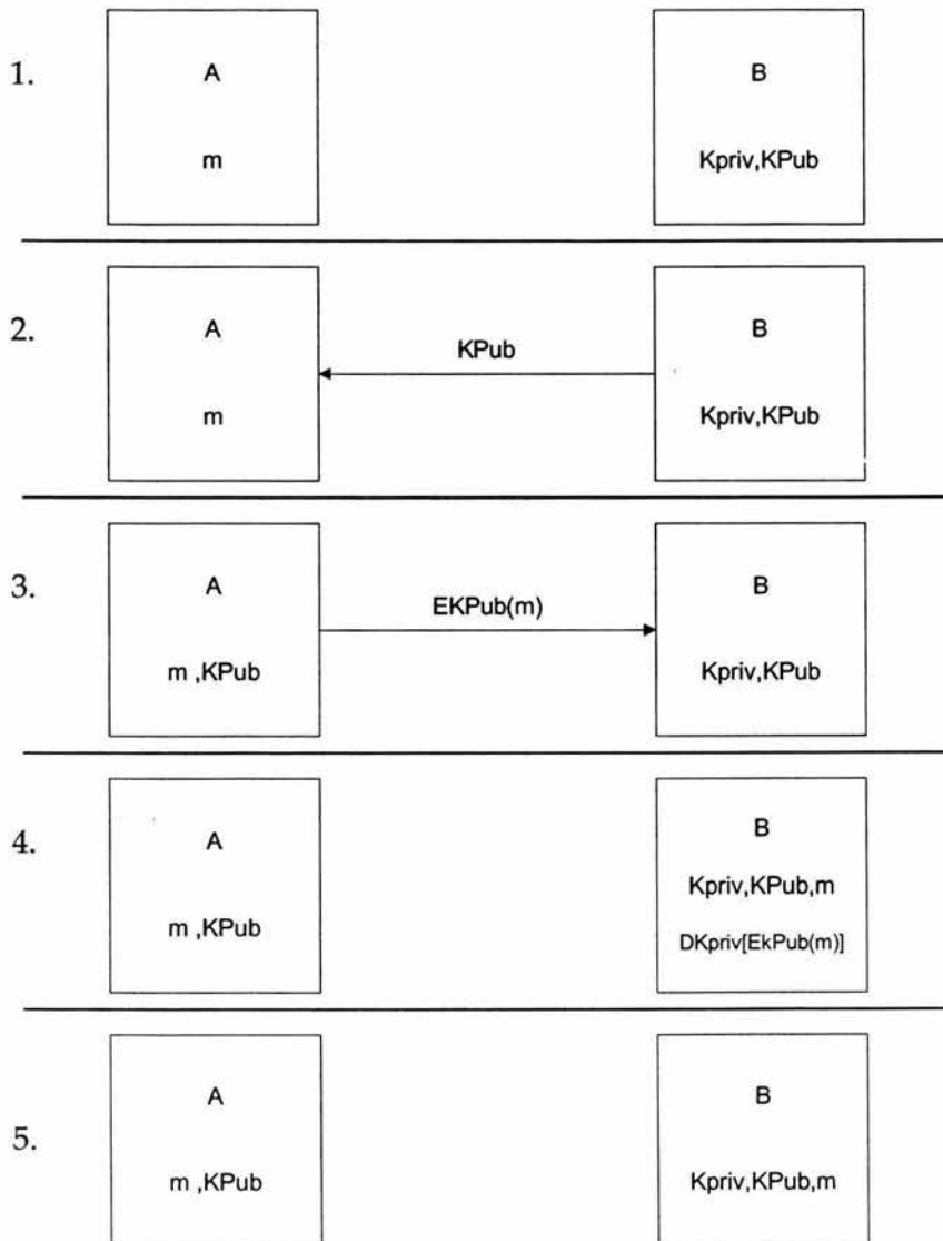
Figura 2.4. Transmisión de información empleando algoritmos asimétricos.
