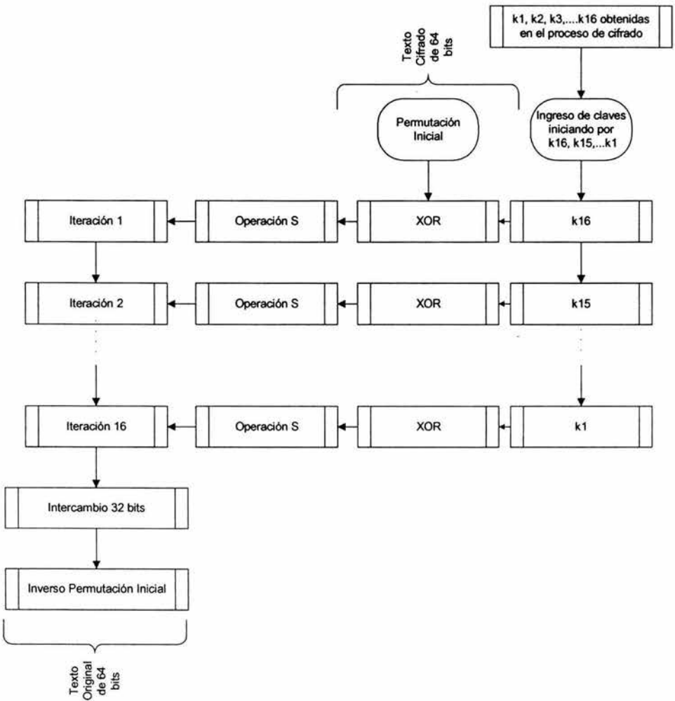
Figura 2.3. Proceso de descifrado con DES
