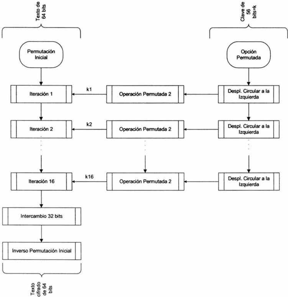
Figura 2.2. Representación del algoritmo DES
