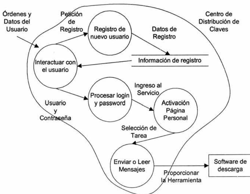
Figura 3.2. Nivel 1 del Diagrama de Flujo de Datos
