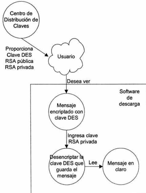
Figura 3.6. Nivel 2 del Diagrama de Flujo de Datos
