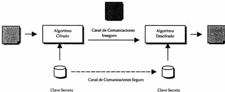
Figura 2.1. Criptosistema para Algoritmo Simétrico de Cifrado
