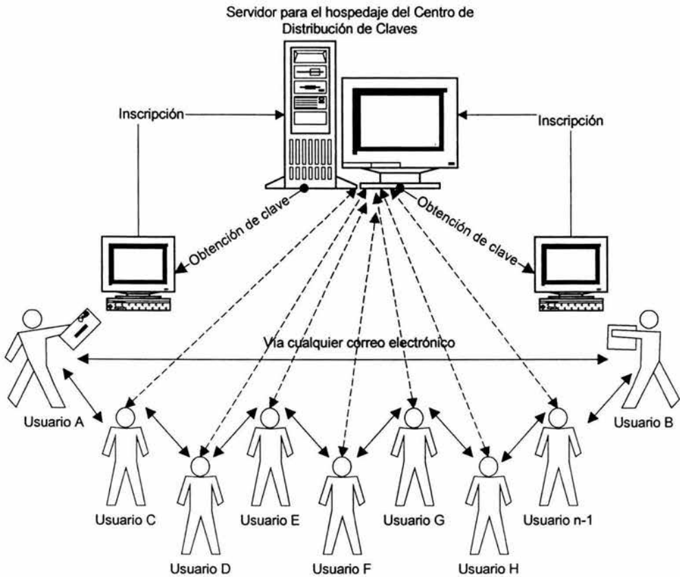
Figura 1.1. Diagrama del Centro de Distribución de Claves
