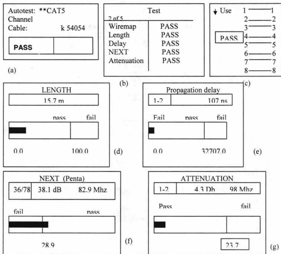
Figura II.43 Equipos de medición
