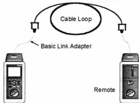
Figura II.41 Auto prueba
