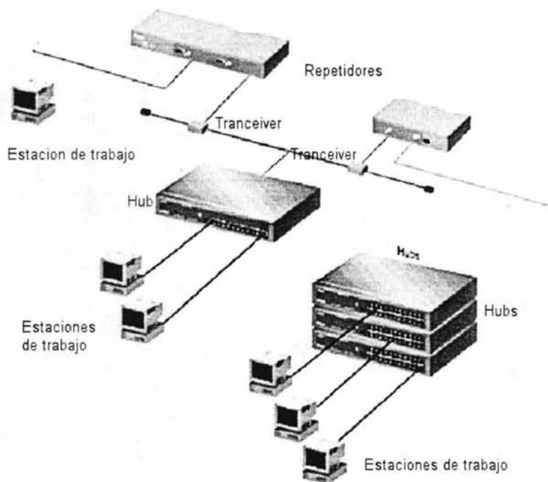
Figura 1.17. Uso de repetidores.
