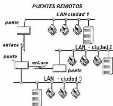
Figura I.20. Puente remoto
