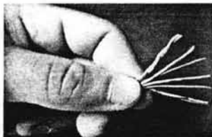
Figura VI.18 Terminado de corte del cable UTP
