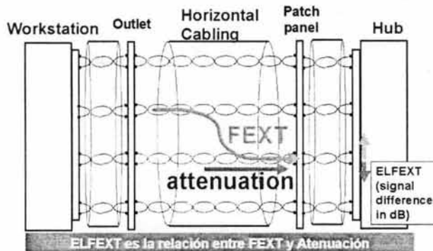
Figura II.36. ELFEXT
