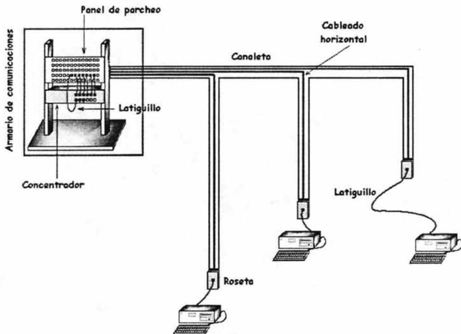
Figura II.2. Cableado Horizontal
