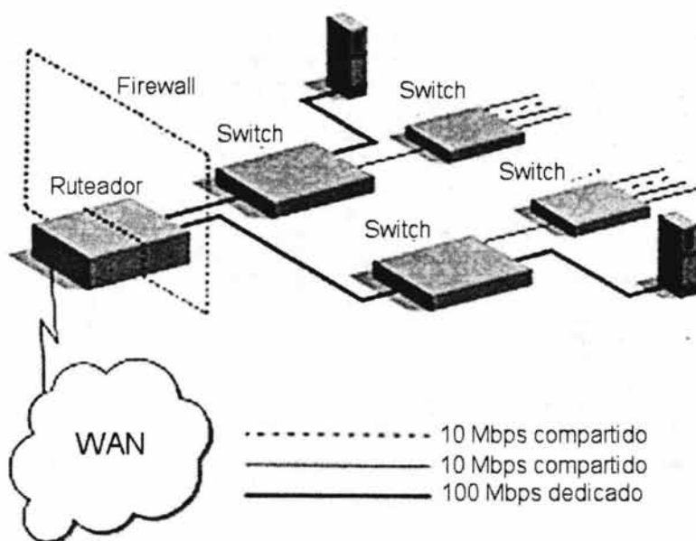
Figura I.21. Uso de ruteadores
