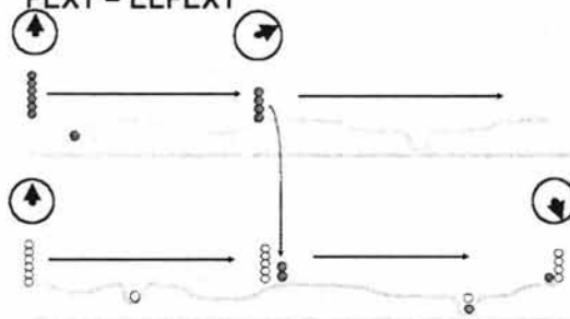
Figura II.37. ELFEXT
