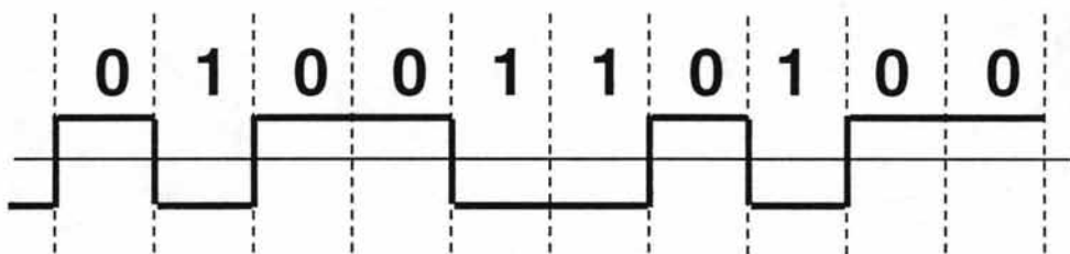
Figura II.23. Transmisión Digital
