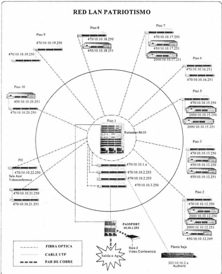
Figura V.1. Estructura de la red LAN en el INEGI.
