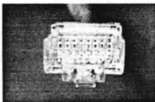
Figura VI.22 Ver de frente que todos los hilos lleguen.
