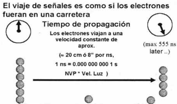
Figura II.29. Velocidad nominal de propagación NVP
