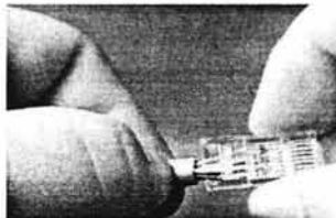
Figura VI.21 Empujar los cables hasta el fondo con la cubierta dentro.
