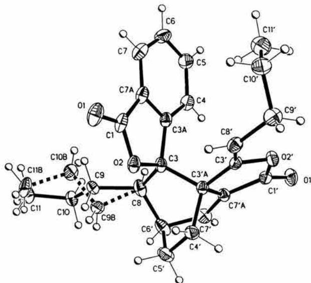
Figura 5. Estructura molecular por rayos X de 46 .
