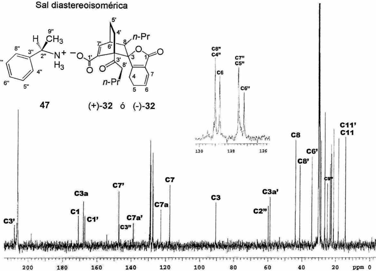
Espectro 50. RMN ^{13}\text{C} de la sal diastereoisomérica del ceto ácido 32 con la amina quiral 47
