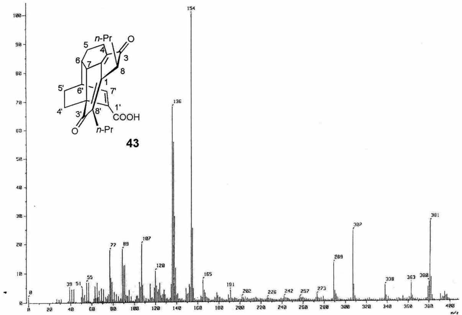
Espectro 33. Masas (FAB) del compuesto 43
