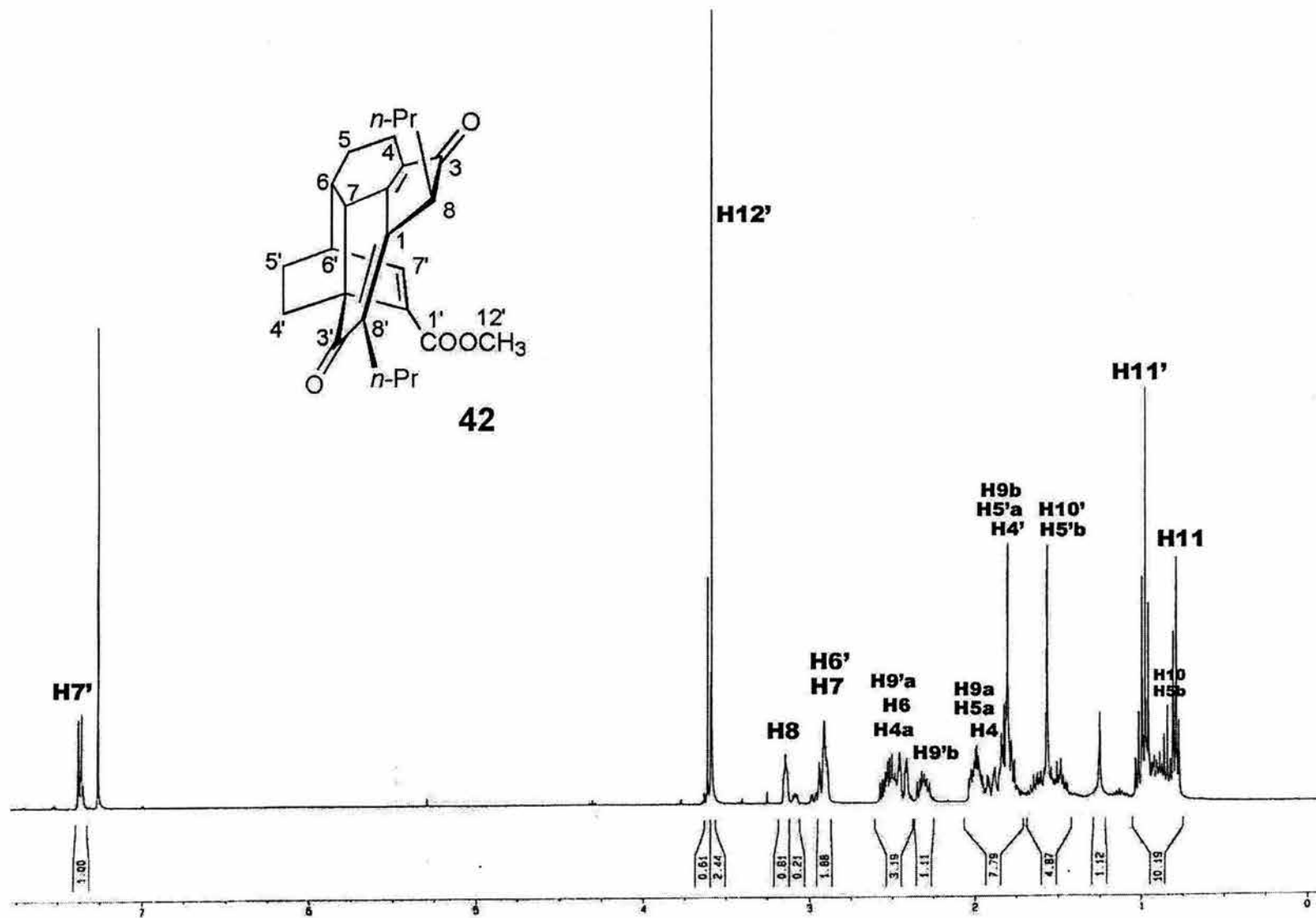
Espectro 28. RMN 1 H del compuesto 42
