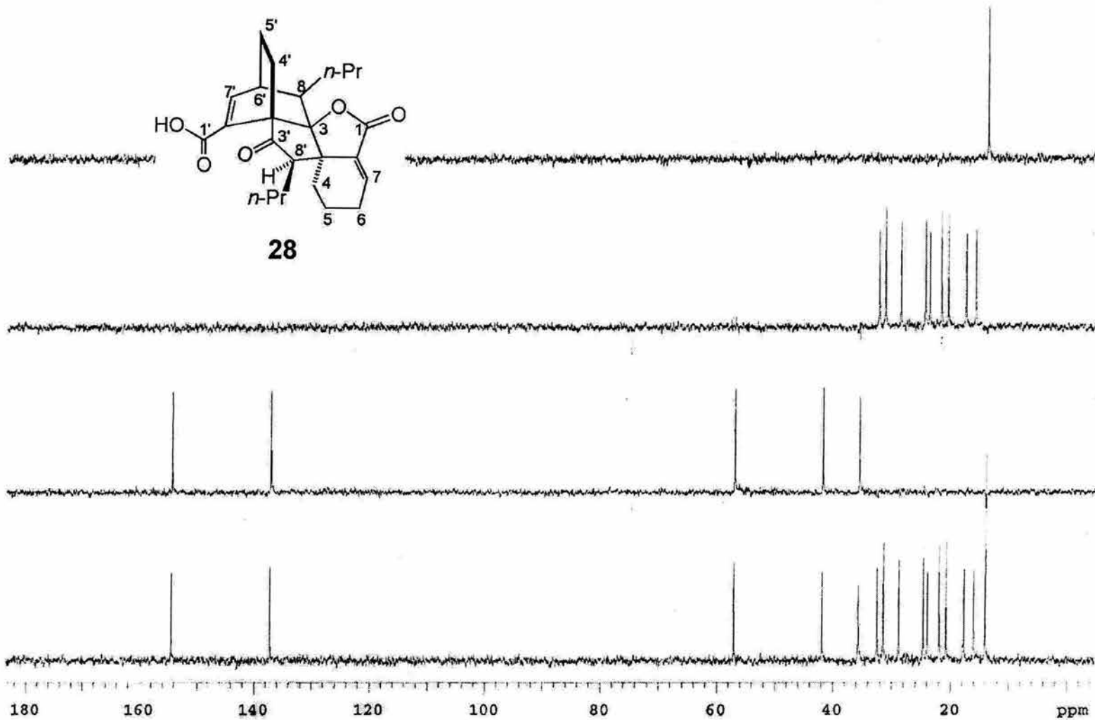
Espectro 10. RMN ^{13}\text{C} (DEPT) de ciclotoquinólida B (28)
