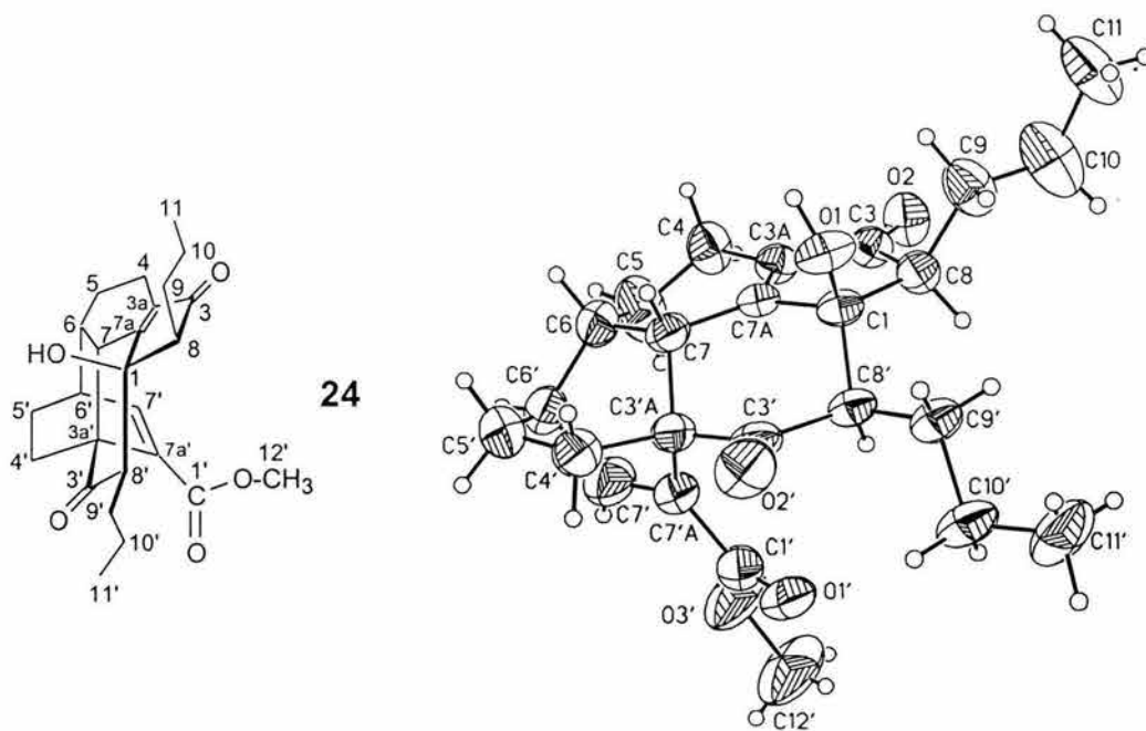
Figura 2. Estructura molecular por rayos X de 24.
