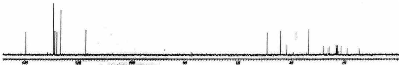
Espectro 56. RMN ^{13}\text{C} (DEPT) de la amida diastereoisomérica del ceto ácido 32 y la amina quiral 47
