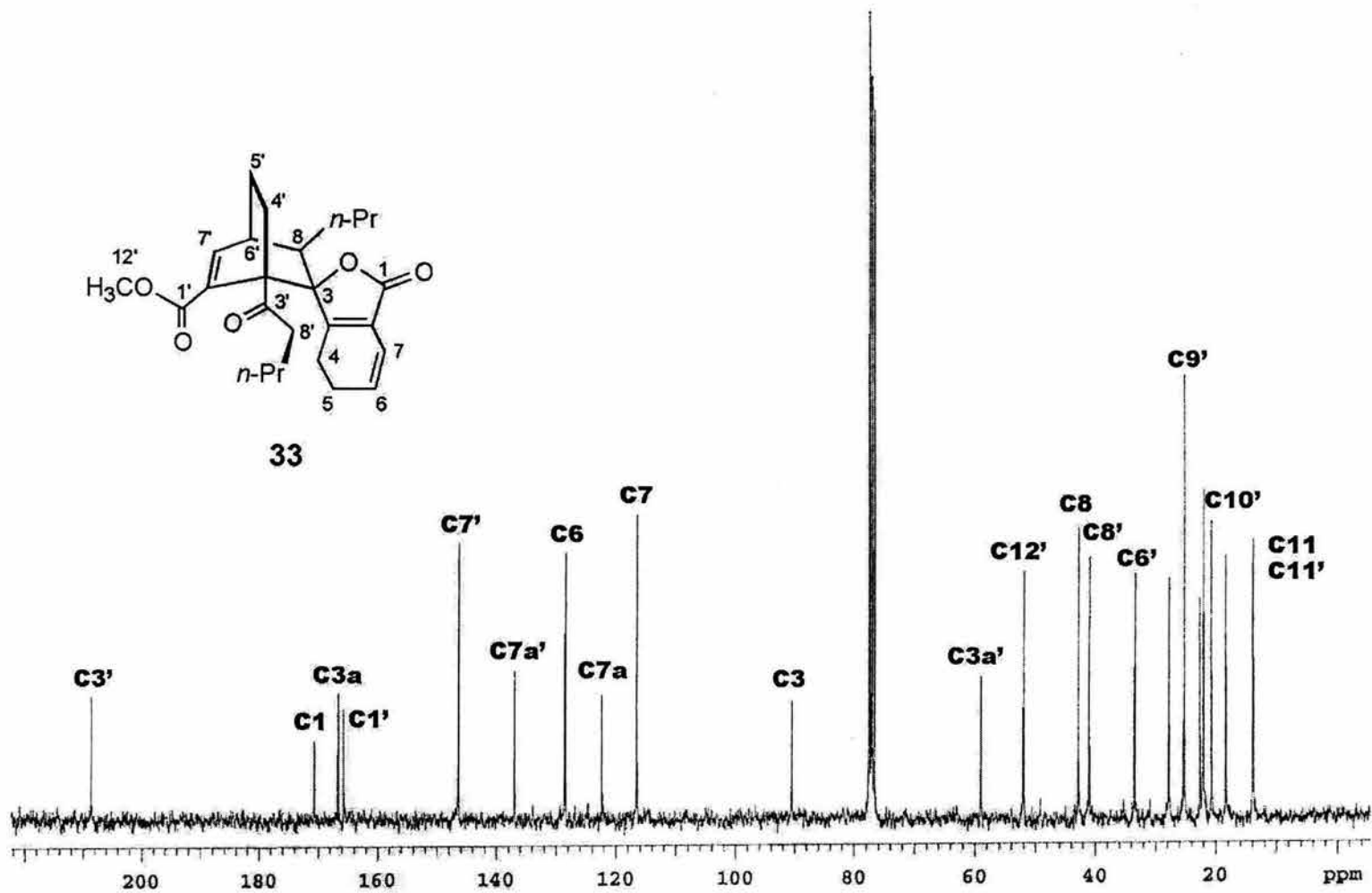
Espectro 13. RMN ^{13}\text{C} del ceto éster 33
