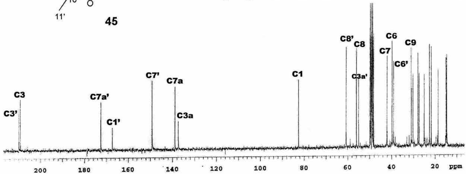
Espectro 39. RMN ^{13}\text{C} del compuesto 45
