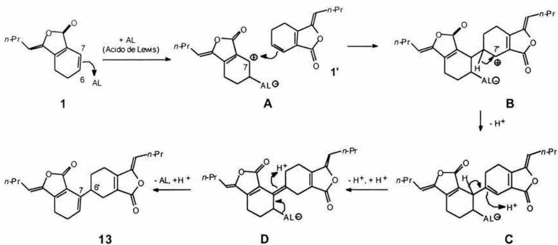
Esquema 7. Mecanismo de formación de 13 .
