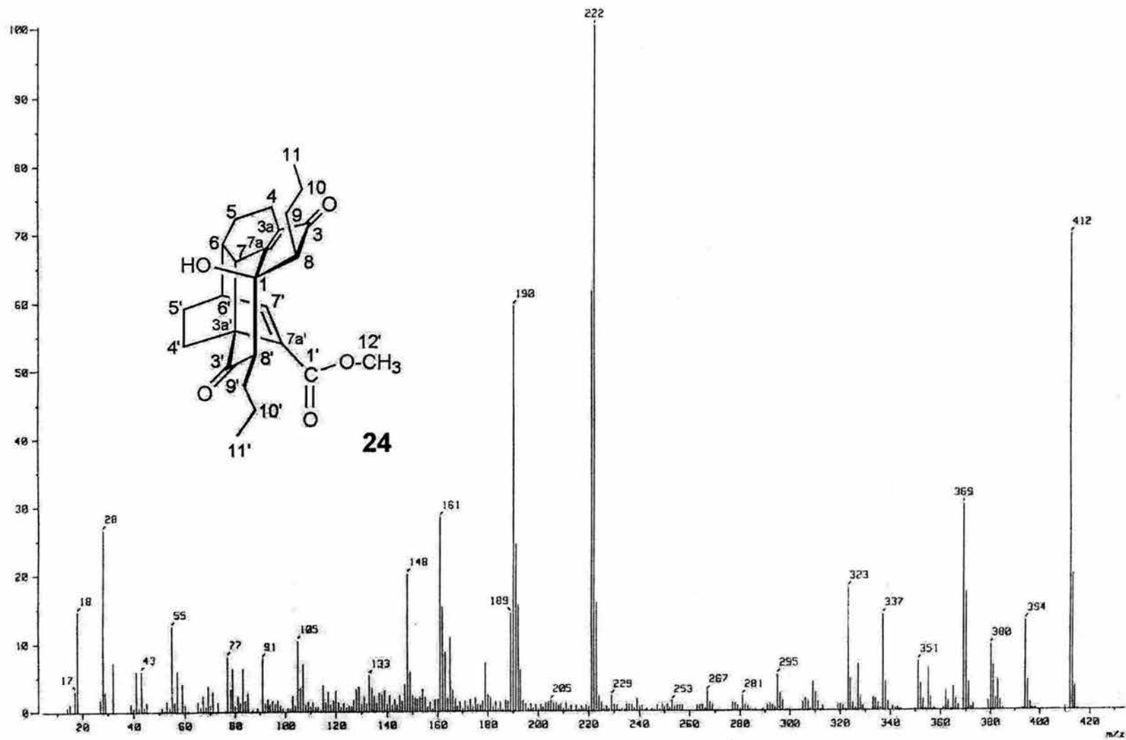
Spectro 18. Masas (IE) del compuesto 24
