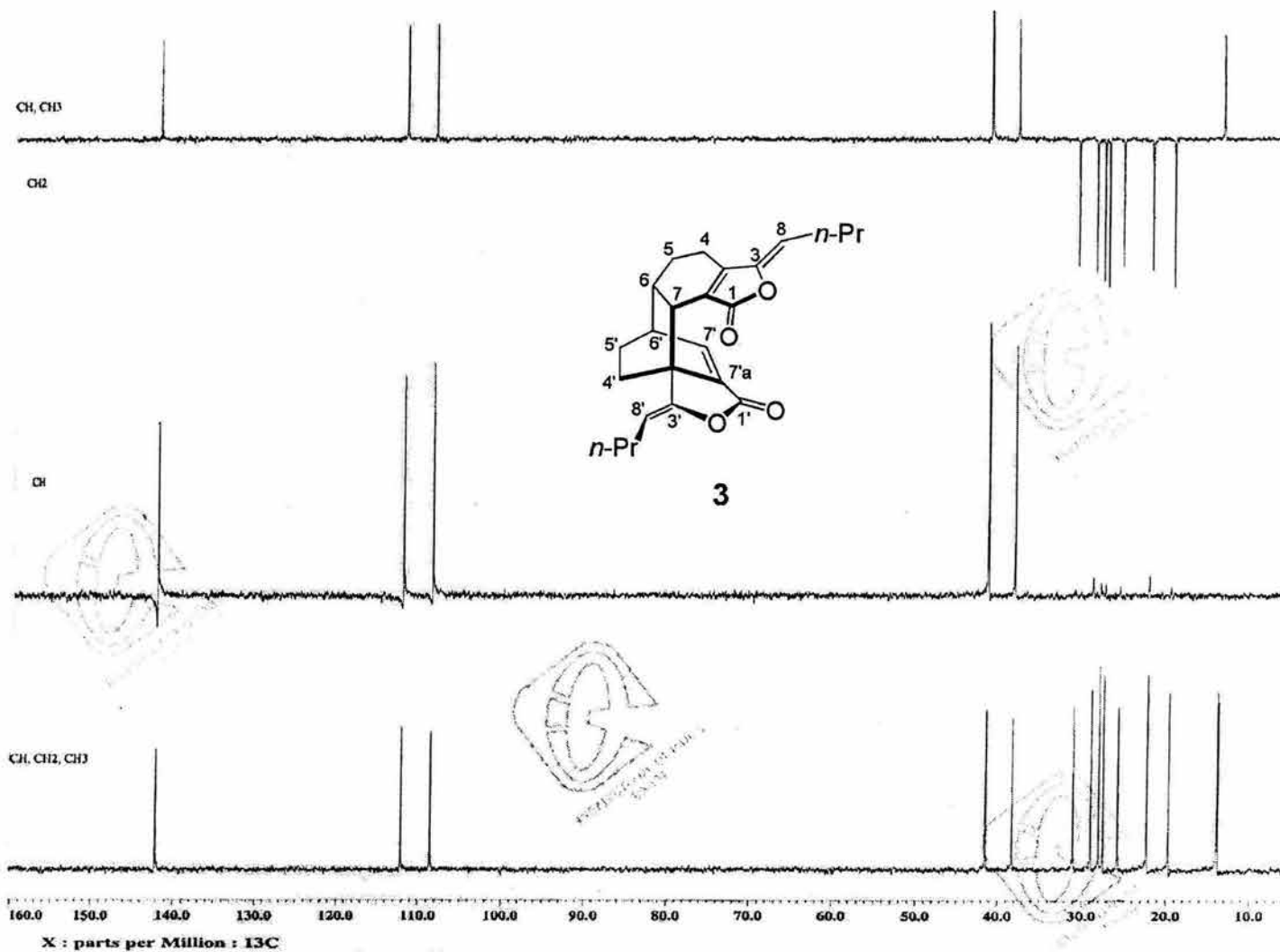
Espectro 4. RMN 13 C (DEPT) de diligustilida (3)
