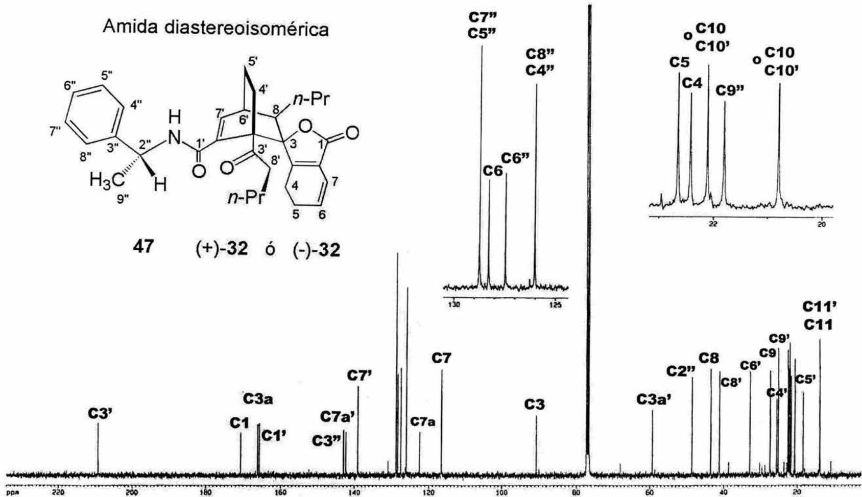
Espectro 55. RMN 13 C de la amida diastereoisomérica del ceto ácido 32 y la amina quiral 47
