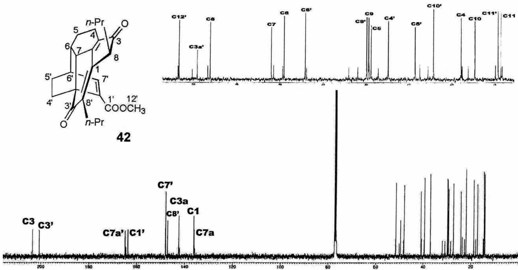
Espectro 29. RMN 13 C del compuesto 42
