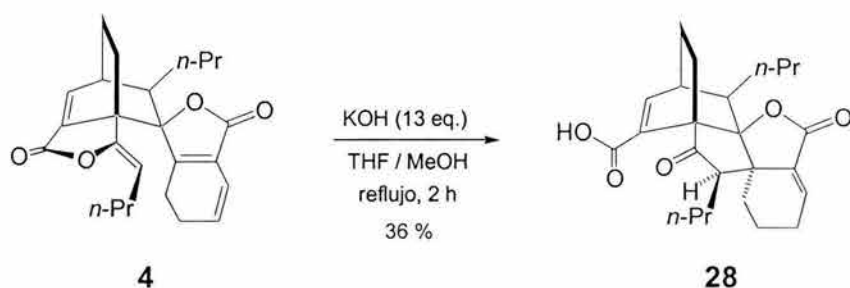
Esquema 25. Obtención de 28 por tratamiento de toquinólida B ( 4 ) con KOH.
