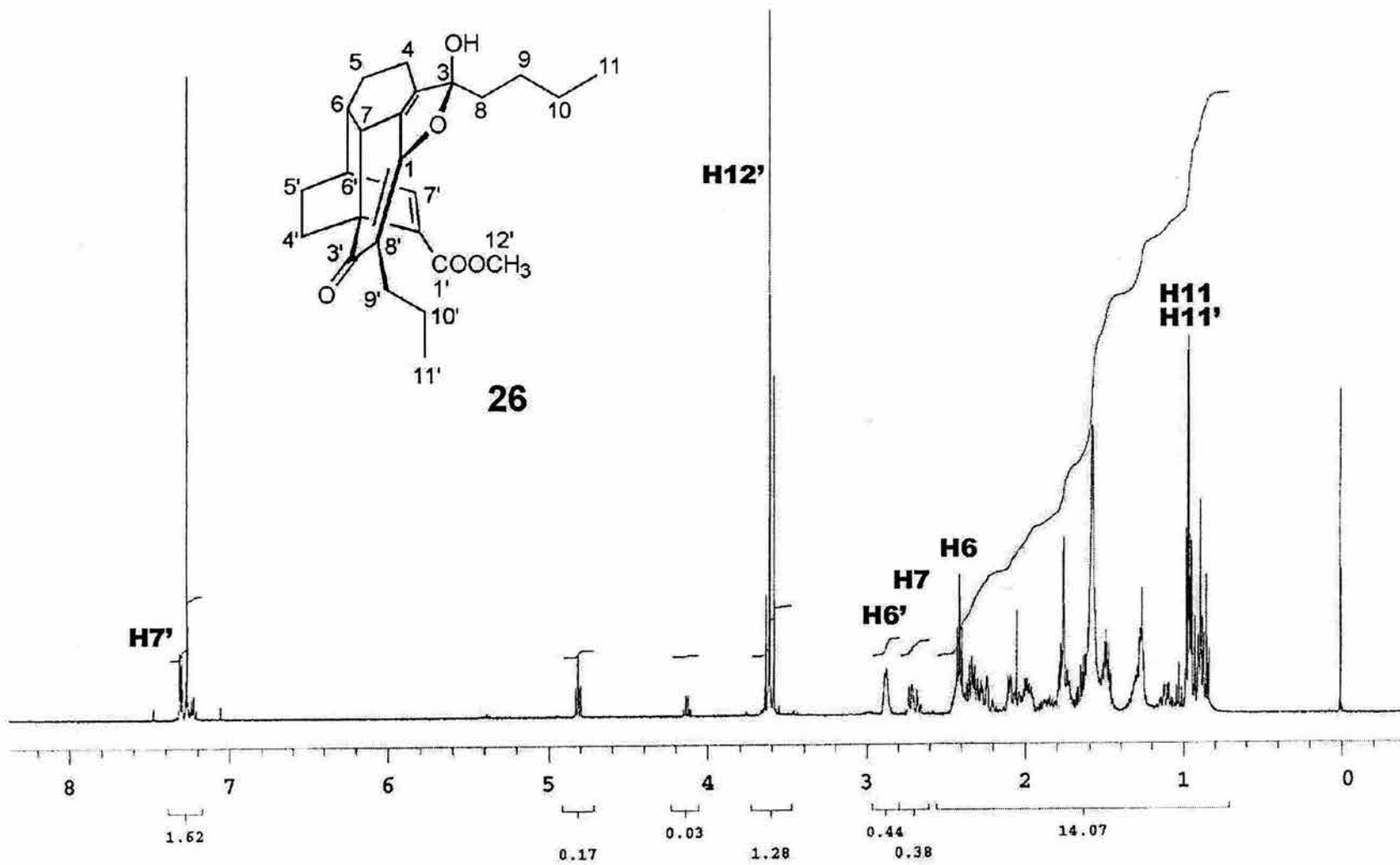
Espectro 24. RMN 1 H del compuesto 26
