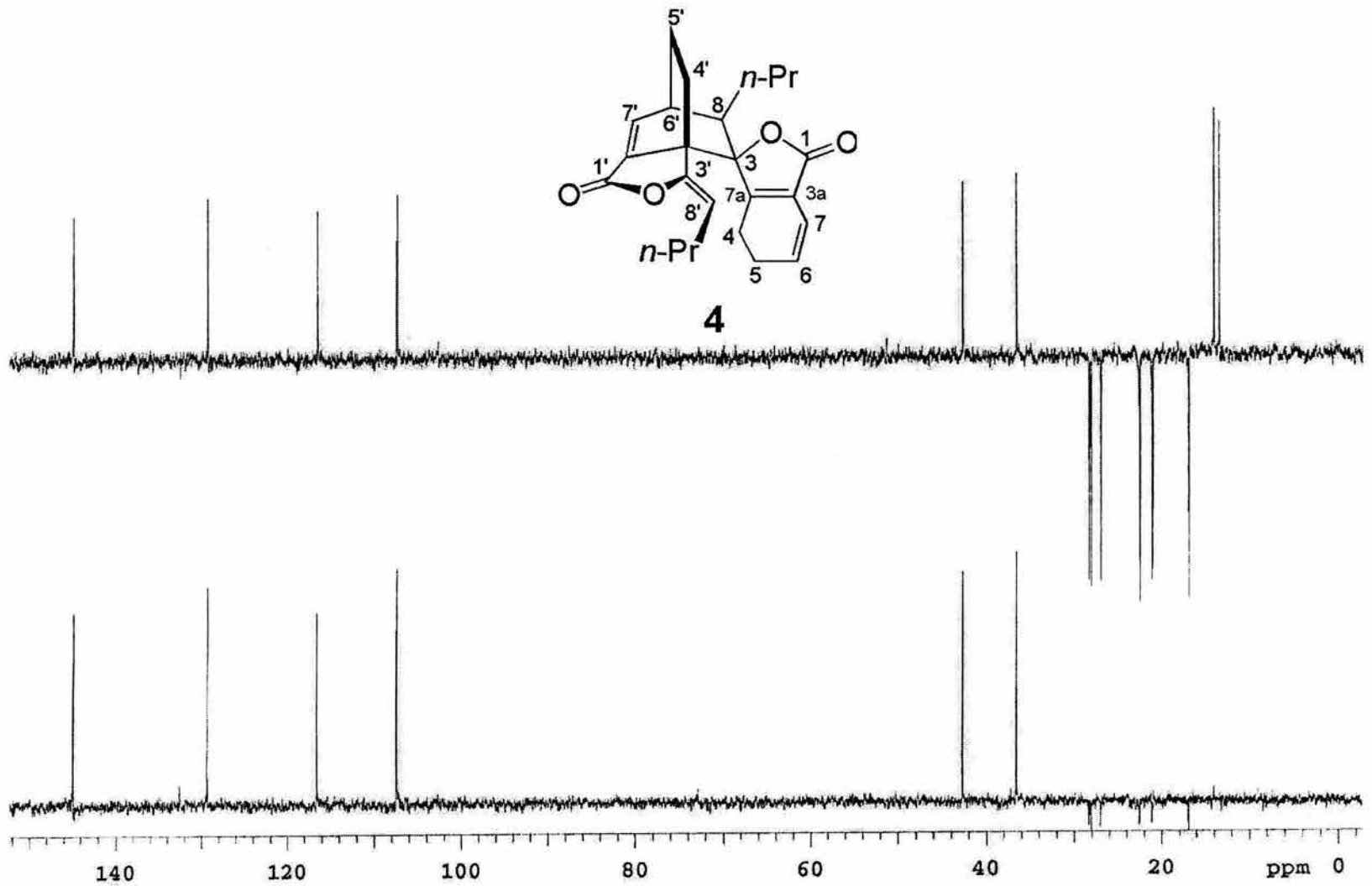
Espectro 7. RMN ^{13}\text{C} (DEPT) de toquinólida B (4)
