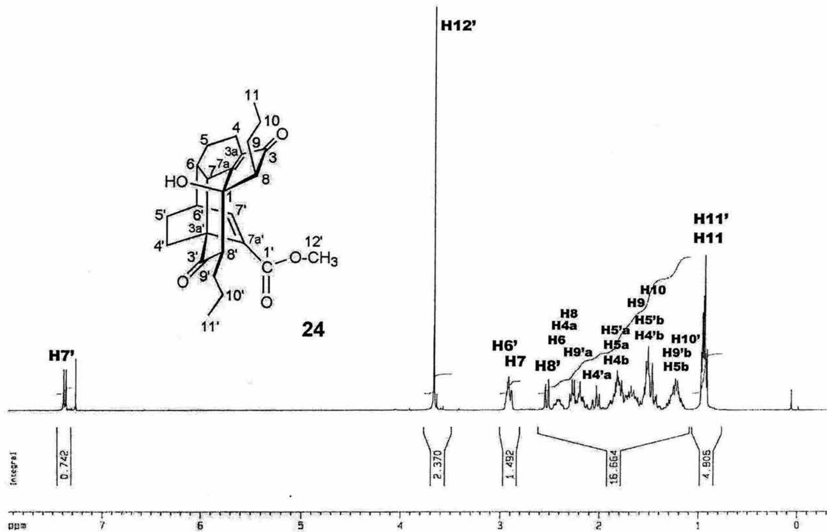
Espectro 15. RMN 1 H del compuesto 24
