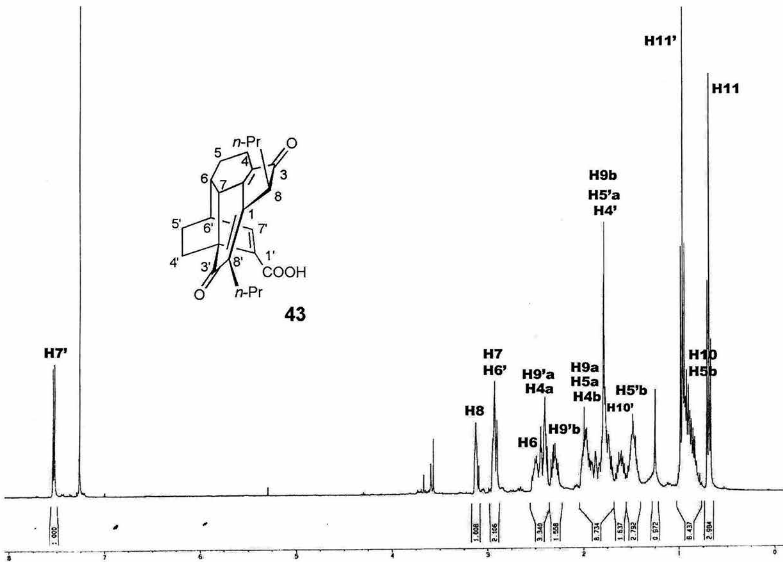
Espectro 31. RMN 1 H del compuesto 43
