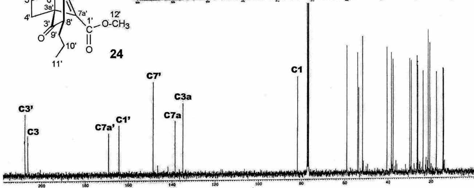
Espectro 16. RMN 13 C del compuesto 24
