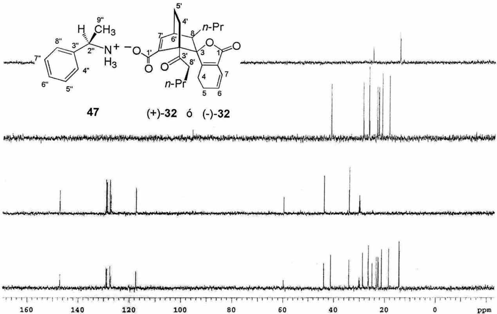
Espectro 51. RMN 13 C (DEPT) de la sal diastereoisomérica del ceto ácido 32 con la amina quiral 47
