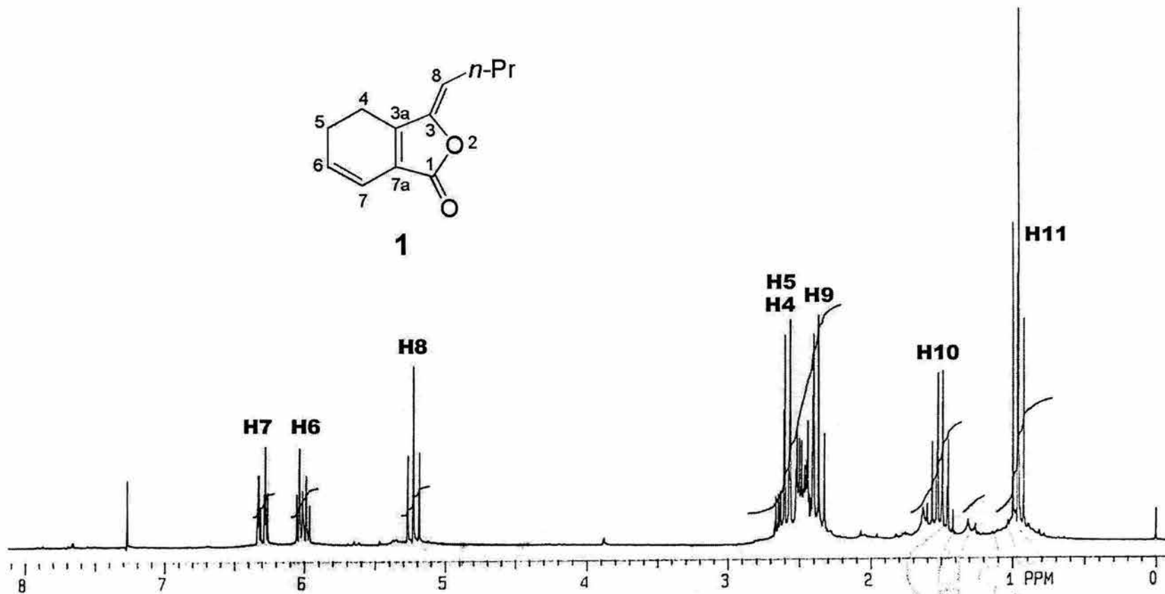
Espectro 1. RMN ^1\text{H} de Z-ligustilida (1)
