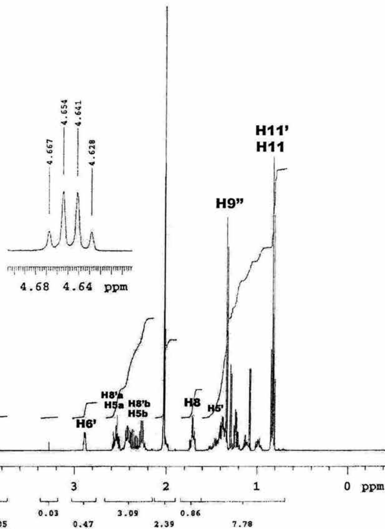
Espectro 49. RMN ^1\text{H} de la sal diastereoisomérica del ceto ácido 32 con la amina quiral 47
