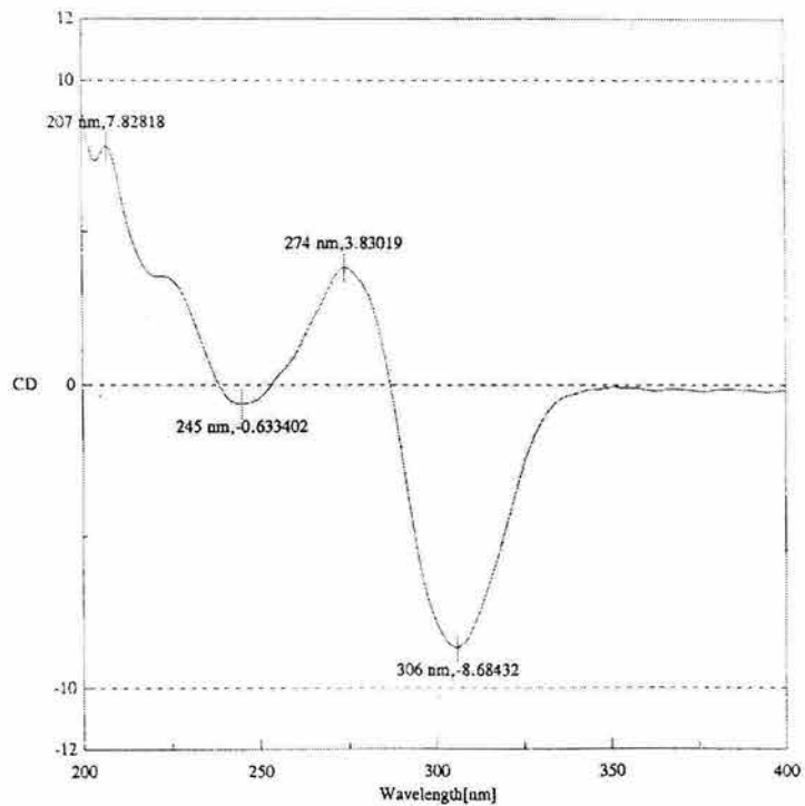
Figura 7. Dicroísmo Circular de la amida diastereoisomérica 55
