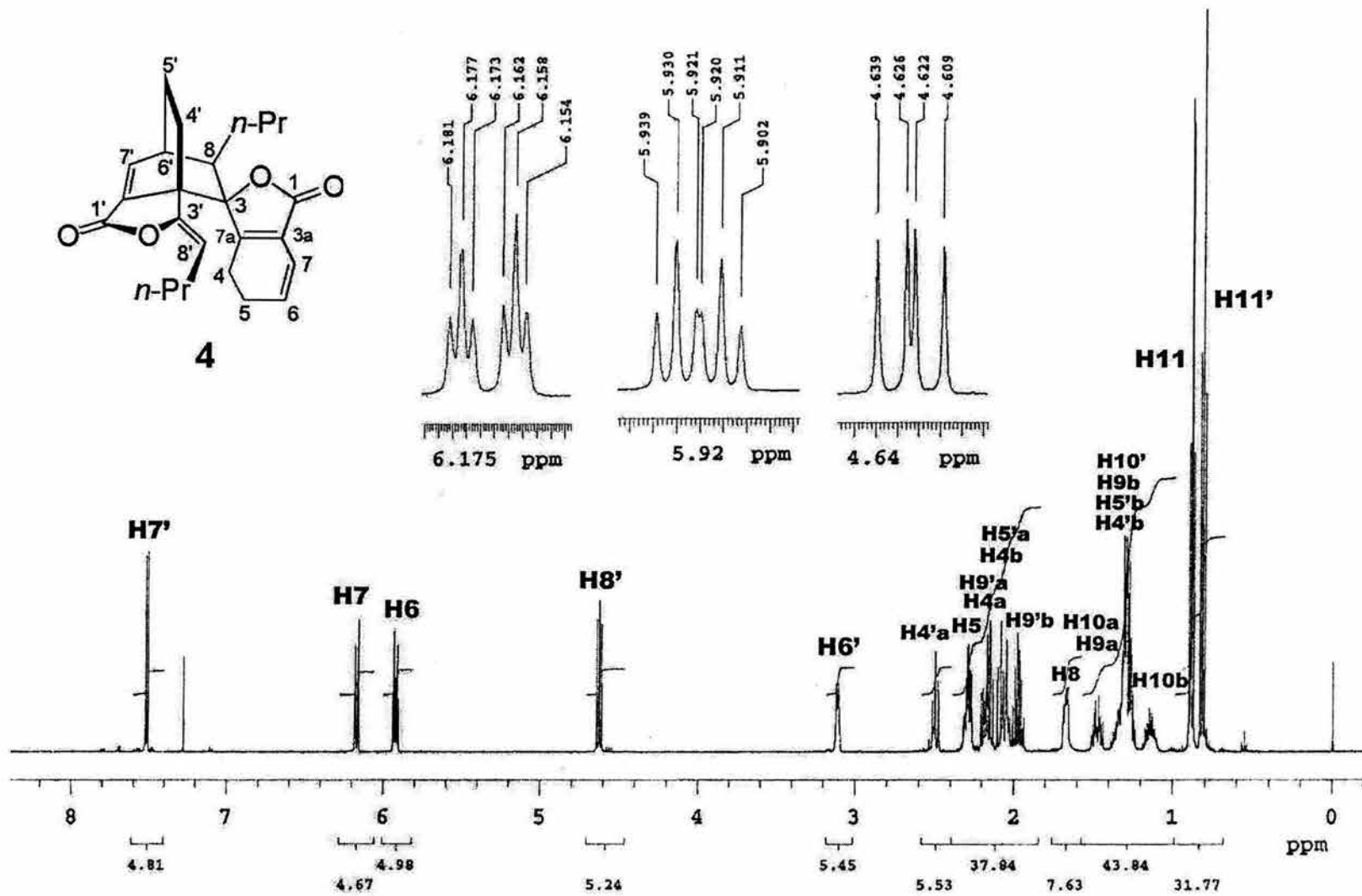
Espectro 5. RMN 1 H de toquinólida B (4)
