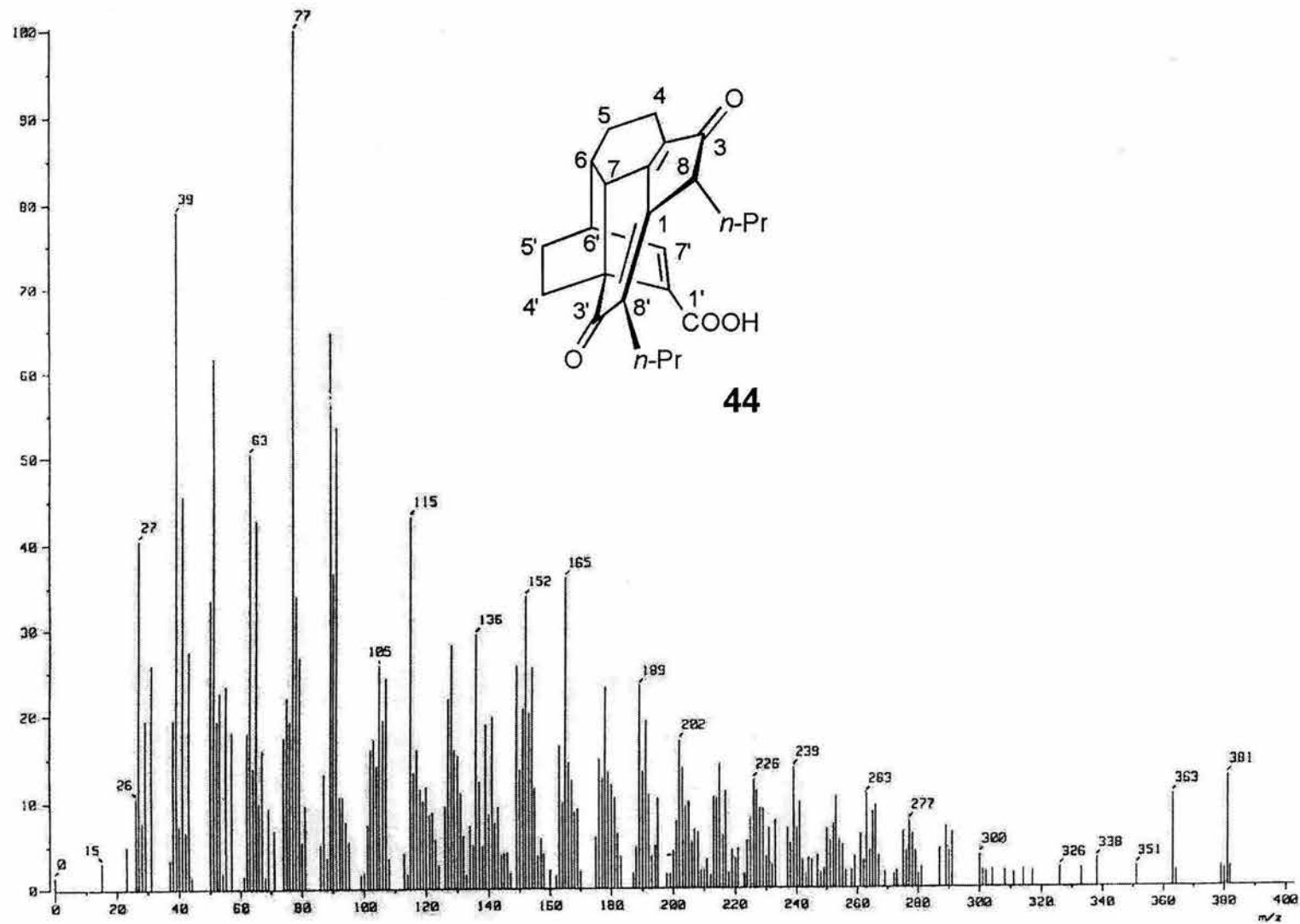
Espectro 37. Masas (FAB) del compuesto 44
