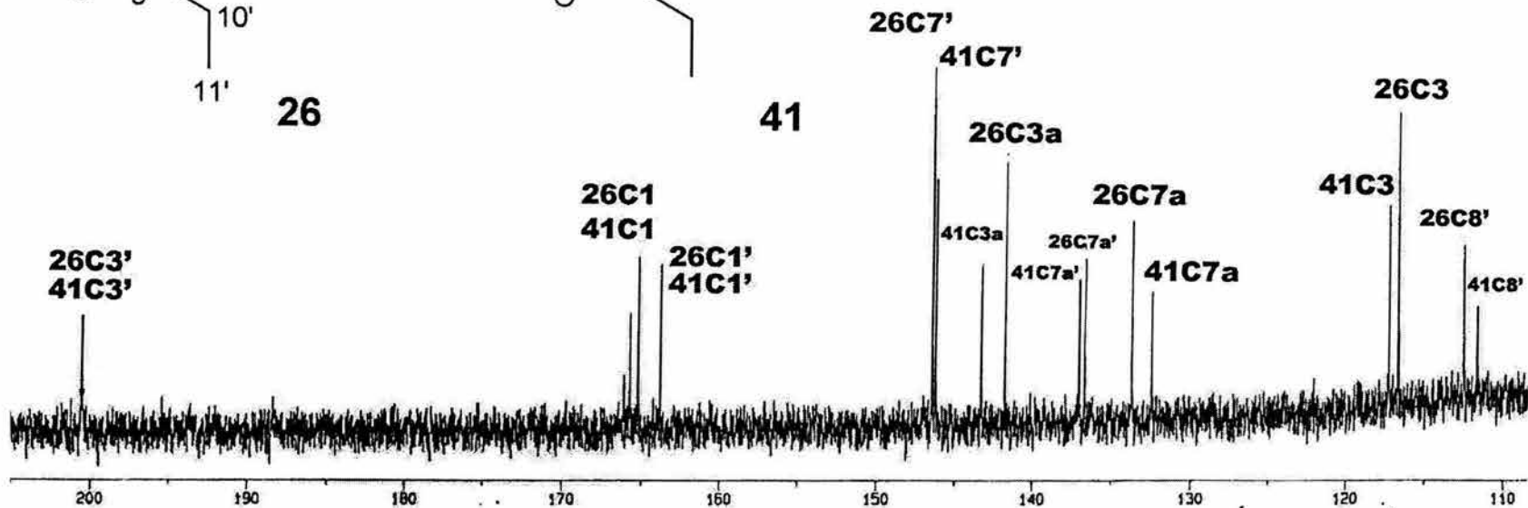
Espectro 26. RMN ^{13}\text{C} de la mezcla de los epimeros 26 y 41
