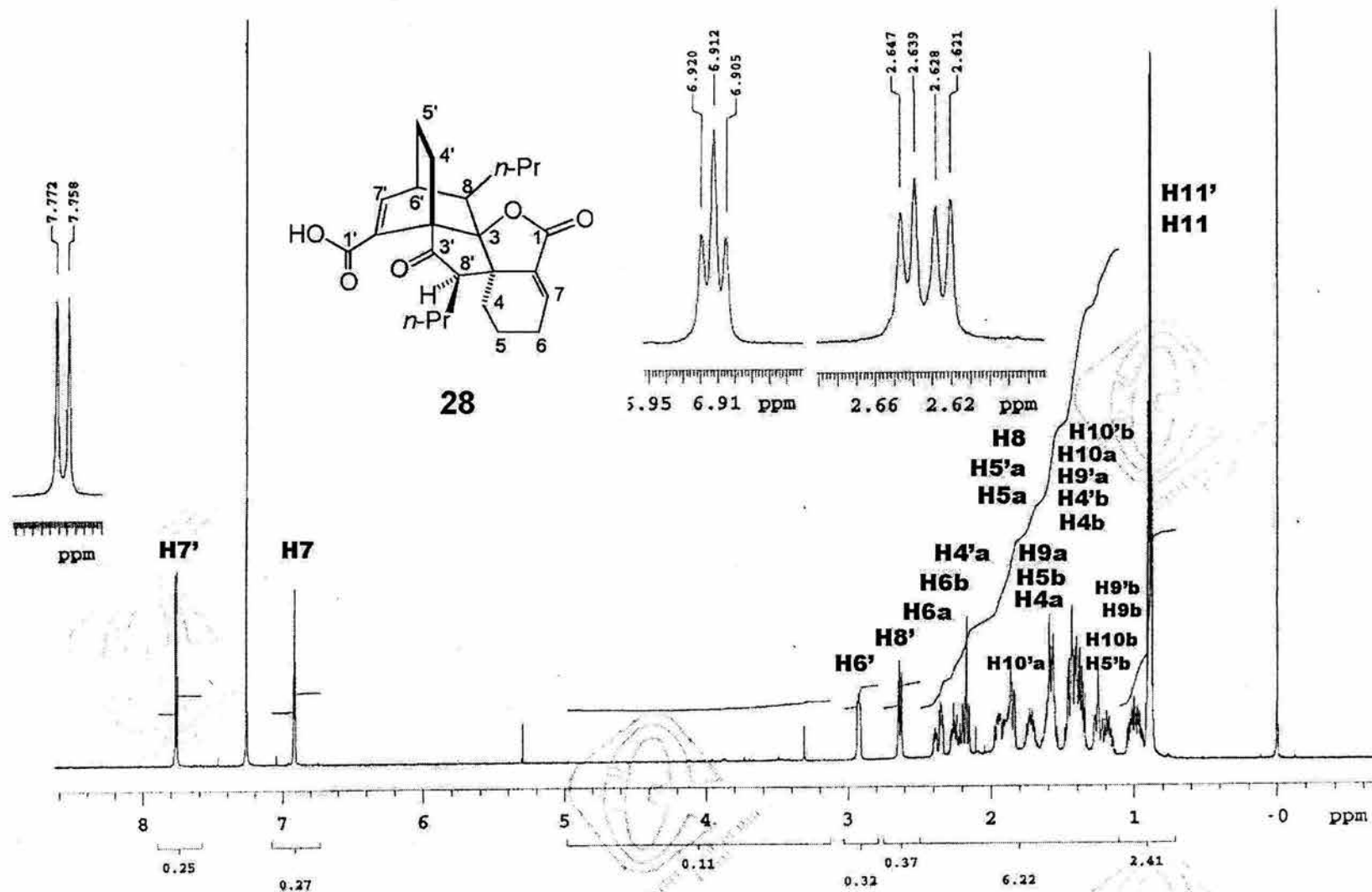
Espectro 8. RMN 1 H de ciclotoquinólida B (28)
