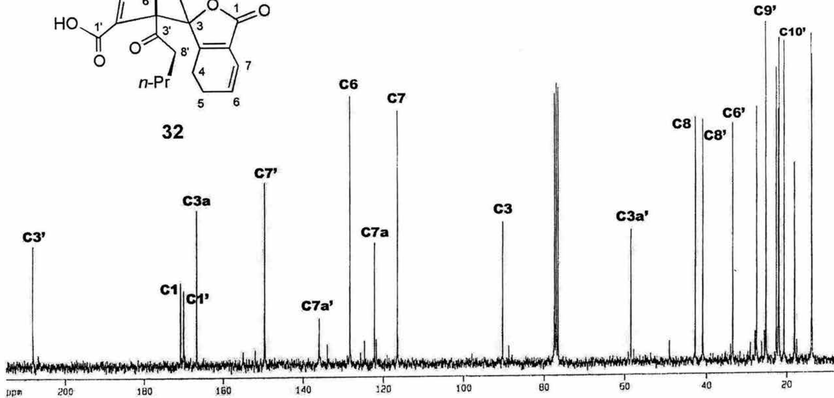
Espectro 47. RMN ^{13}\text{C} Ceto ácido 32
