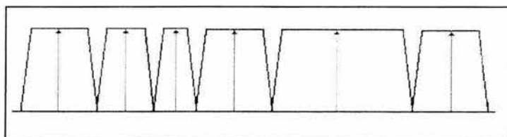
Figura 3.2 Efecto del transpondedor MCPC.
