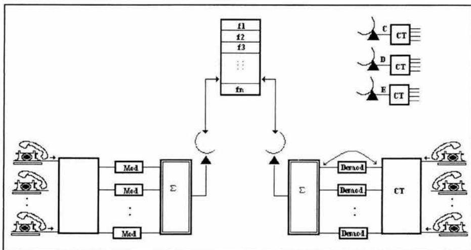
Figura 3.4 Sistema SCPC.
