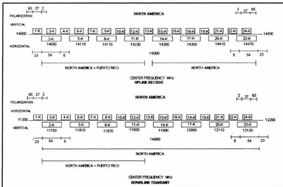
Plan de frecuencias en Banda Ku
