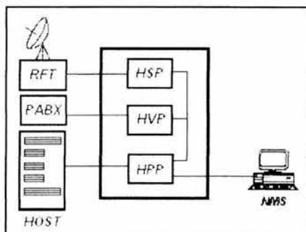
Figura 4.6 Arquitectura interna de la Estación Maestra de una VSAT.
