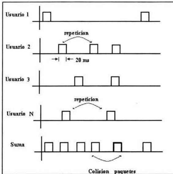
Figura 3.11 Ejemplo de una transmisión con colisión.
