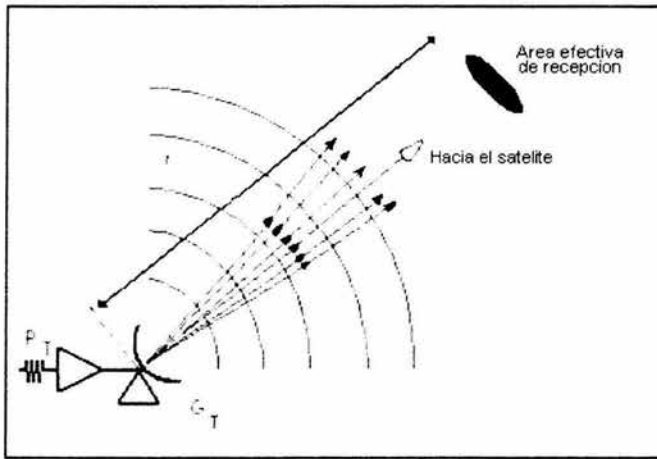
Figura 5.5 PIRE y área efectiva de recepción.
