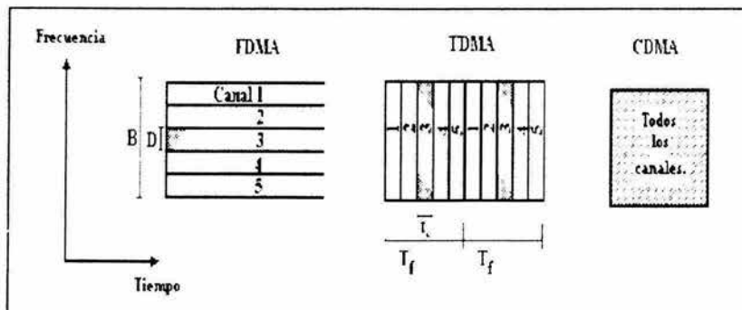
Figura 3.1 Técnicas básicas de acceso múltiple.
