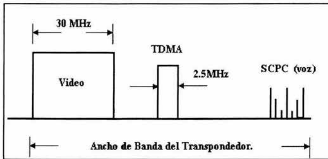
Figura 3.8 Transpondedor multiservicio de TDMA de banda angosta.
