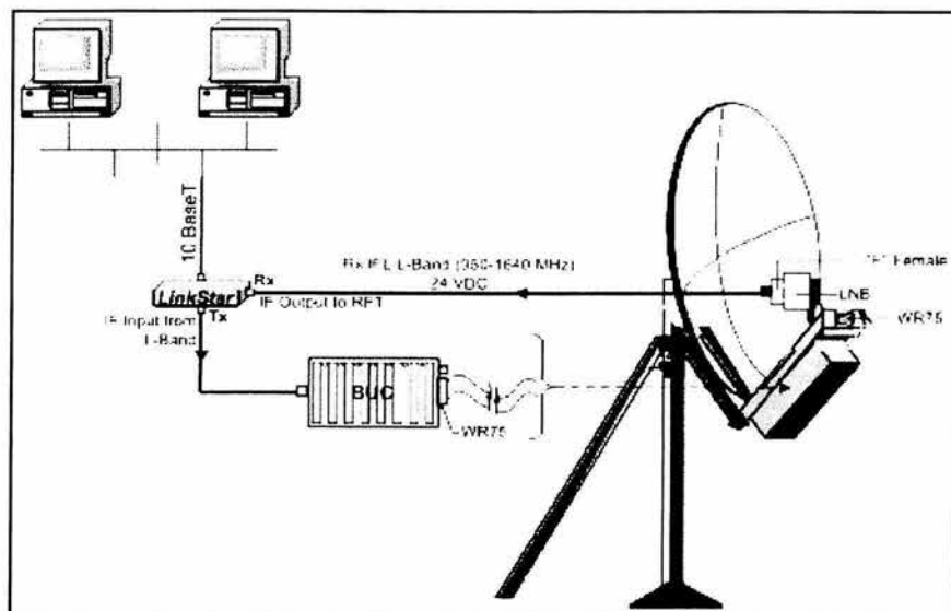
Figura 7.5 Descripción de una Estación Terrena Terminal de una red LinkStar.
