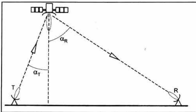
Figura 7.9 Pérdidas por desapuntamiento.
