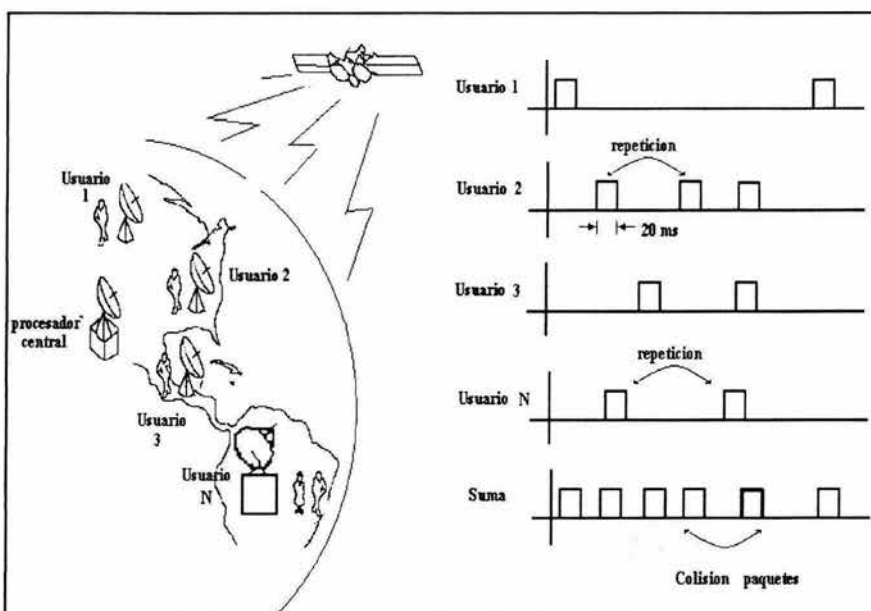
Figura 3.10. Operación del Sistema Aloha.
