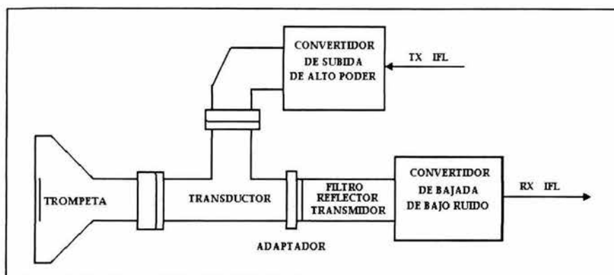
Figura 4.7 Componentes RF del ODU.
