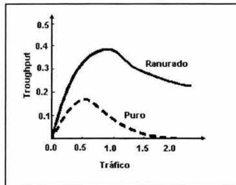
Figura 3.12 Throughput contra Tráfico en canales Aloha.
