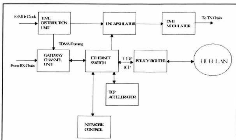
Figura 7.3 Diagrama de bloques del funcionamiento del hub de una red LinkStar.
