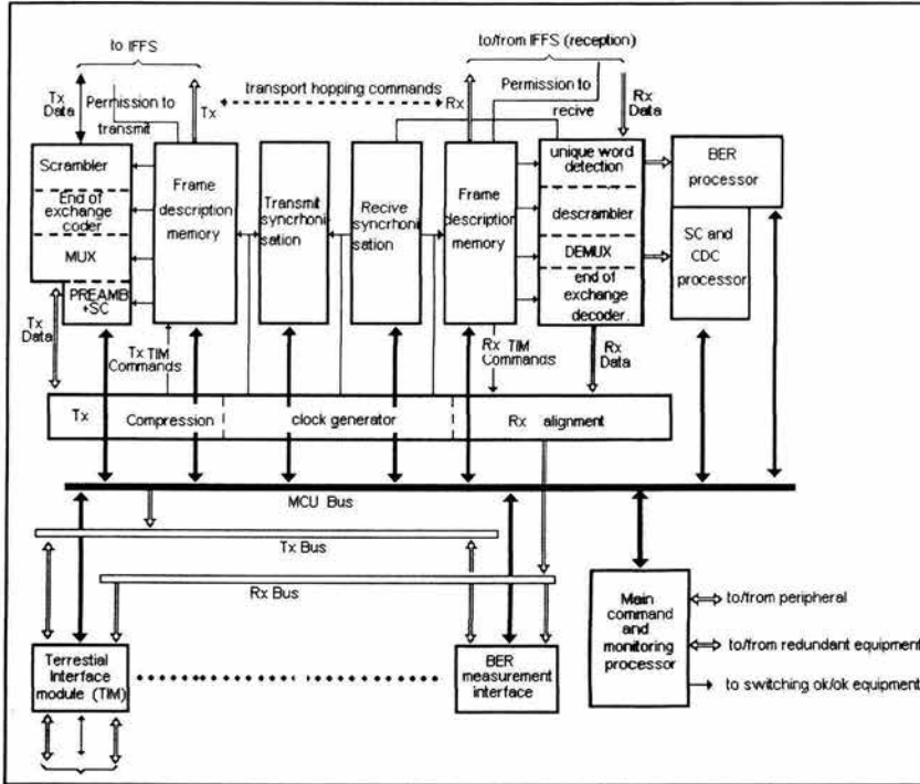
Figura 4.10 Diagrama de bloques del equipo lógico común.
