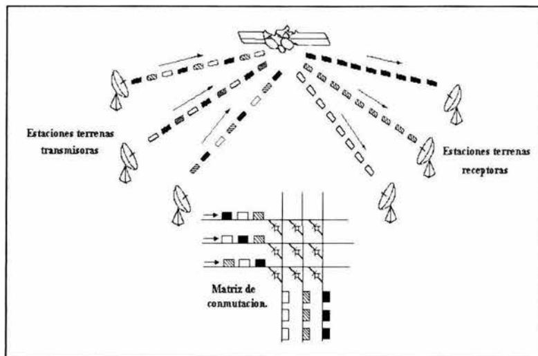
Figura 3.9 TDMA con conmutación en el satélite.
