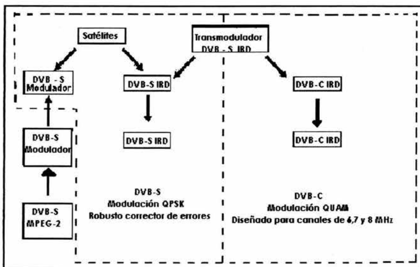
Transmodulación de una señal
