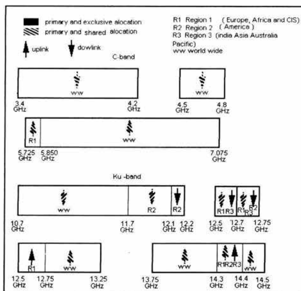
Figura 4.11 Bandas de frecuencia asignadas en una VSAT.
