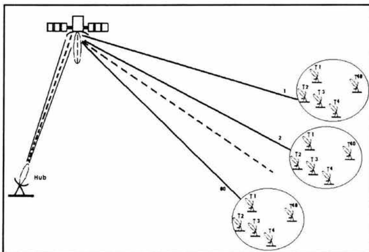
Figura 7.6 Distribución de VSATs y asignación de portadoras.
