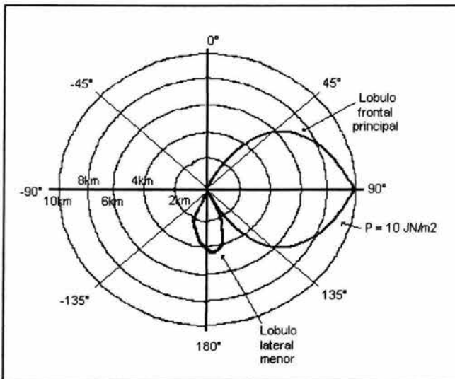
Figura 5.4 Diagrama de la muestra de un patrón de radiación.
