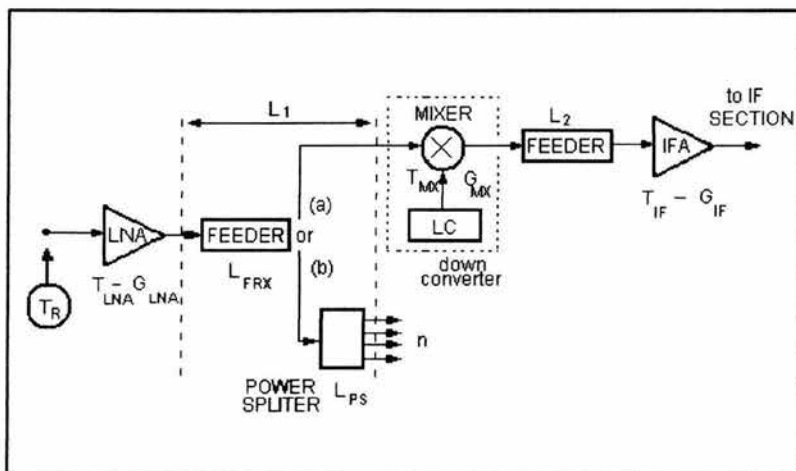
Figura 4.9 Diagrama de bloques del receptor.
