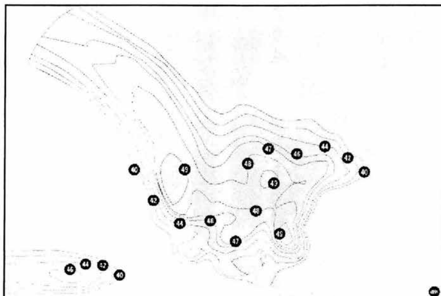
Polarización vertical en Banda Ku
