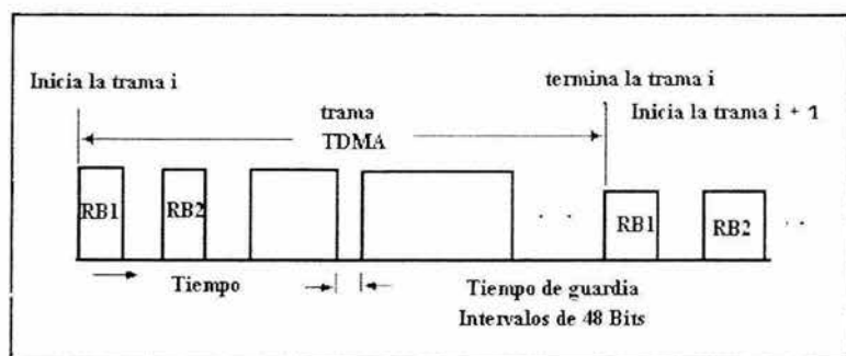
Figura 3.7 Trama de TDMA.
