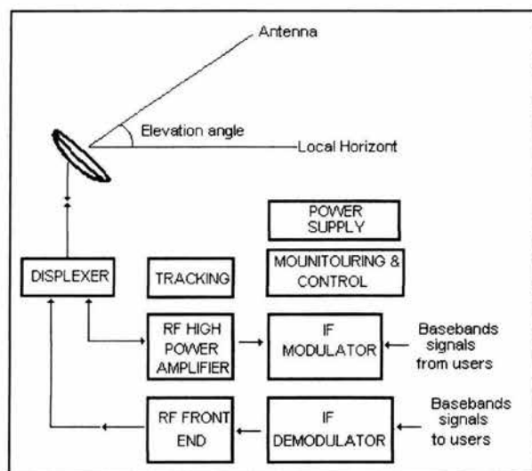
Figura 5.2 Organización de una estación terrena.
