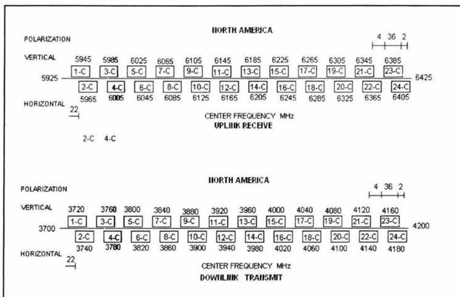
Plan de frecuencias en Banda C
