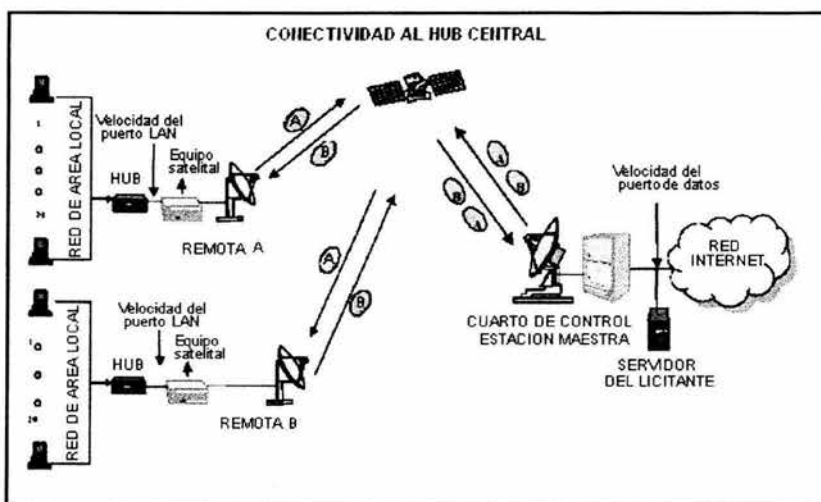
Figura 6.1 Diagrama de conectividad al hub central.
