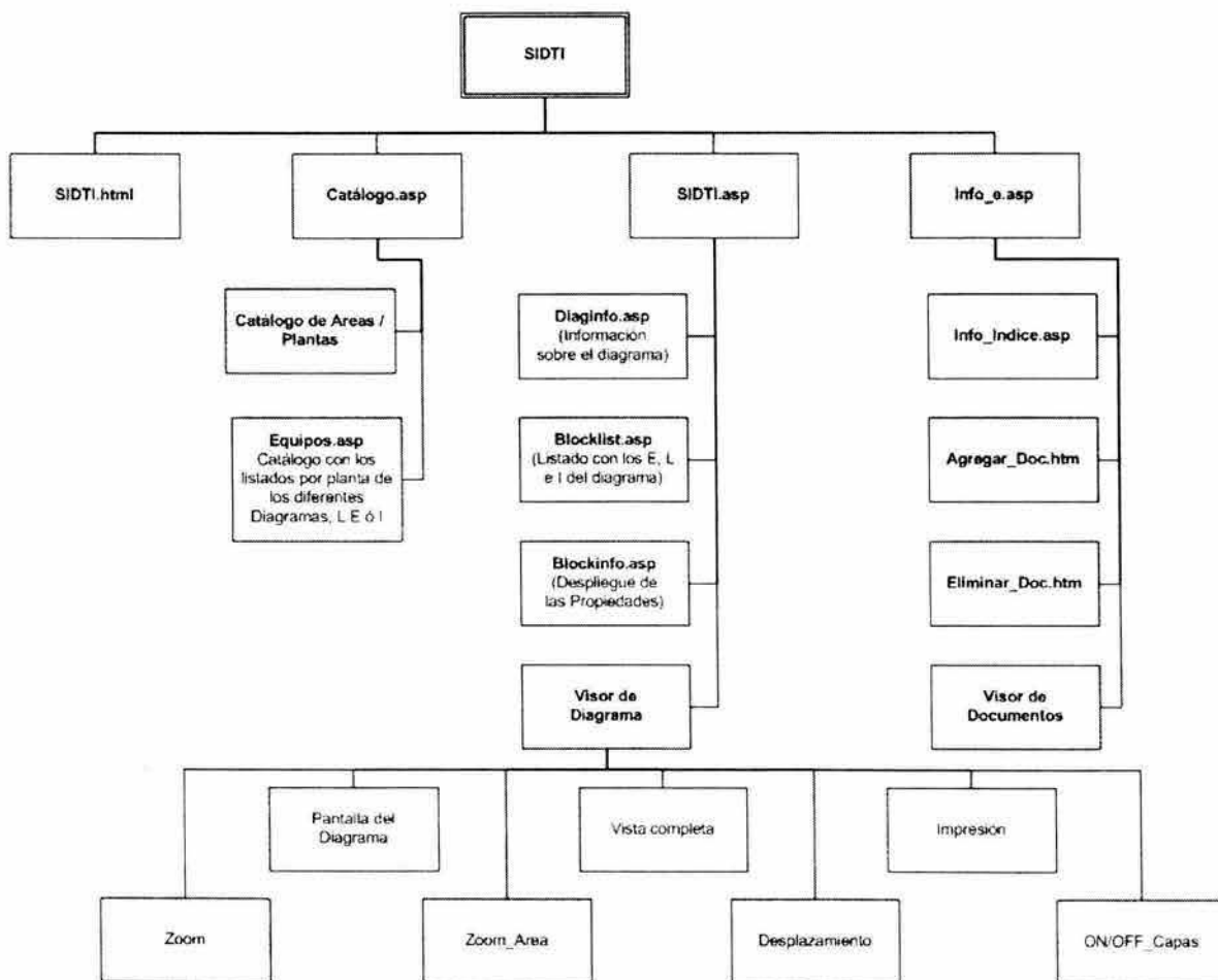
Figura 2.2. Carta estructurada.
