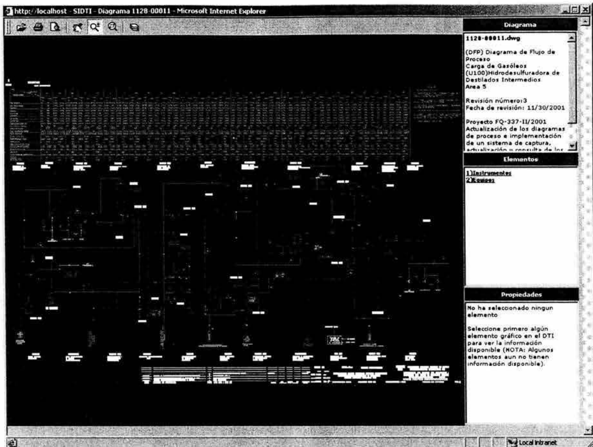
Figura 3.3 SIDTI.asp
