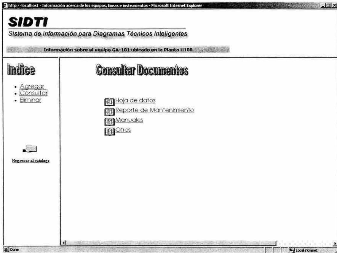
Figura 3.7 Consultas.asp
