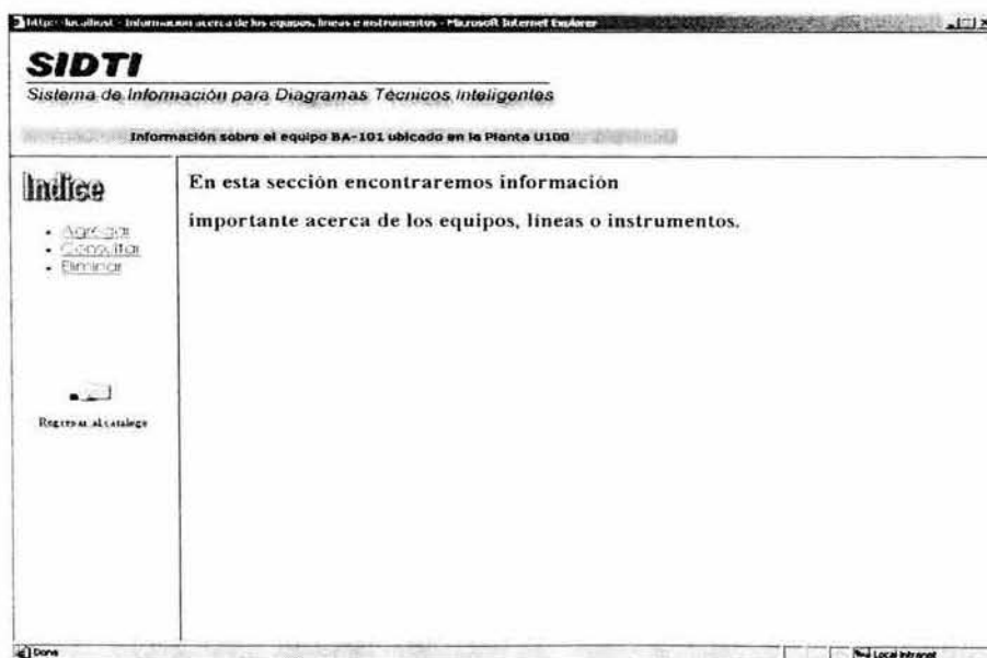
Figura 2.3. Interfaz nueva
