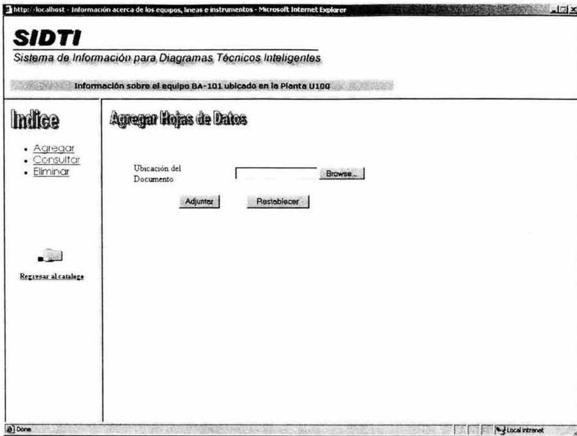
Figura 3.6 Agregar_HD.asp
