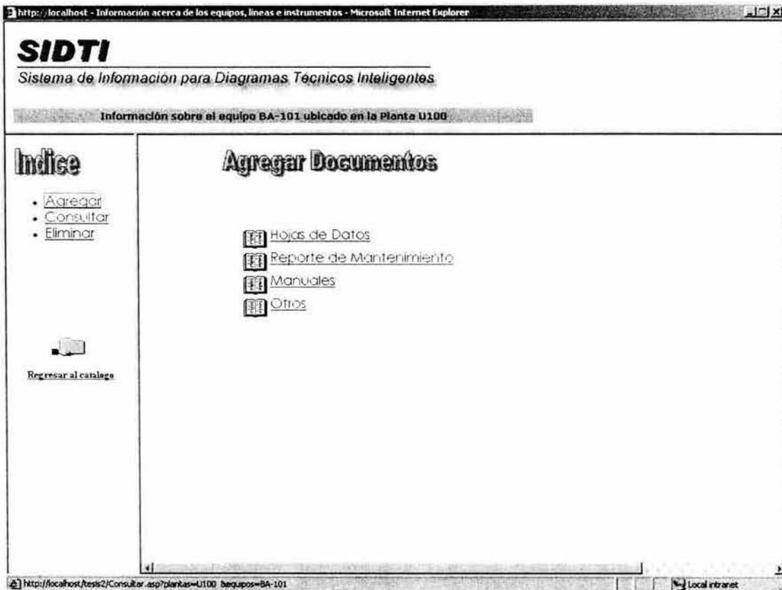
Figura 3.5 Agregar_Doc.asp
