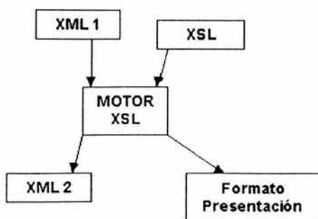
Fig. 1.4.2.1. –1 Esquema de Acoplamiento de Archivos.
