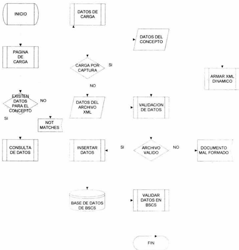
Figura. 3.2.8 –1 Diagrama de Flujo del proceso de cargas.
