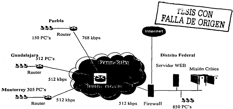
Figura 3.1. Arquitectura de Red WAN.
