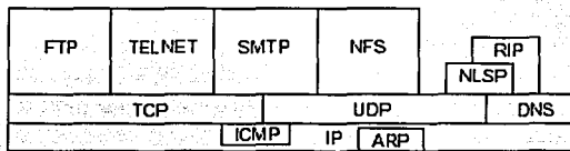
Figura 1.3. El protocolo stack de Internet o TCP/IP.
