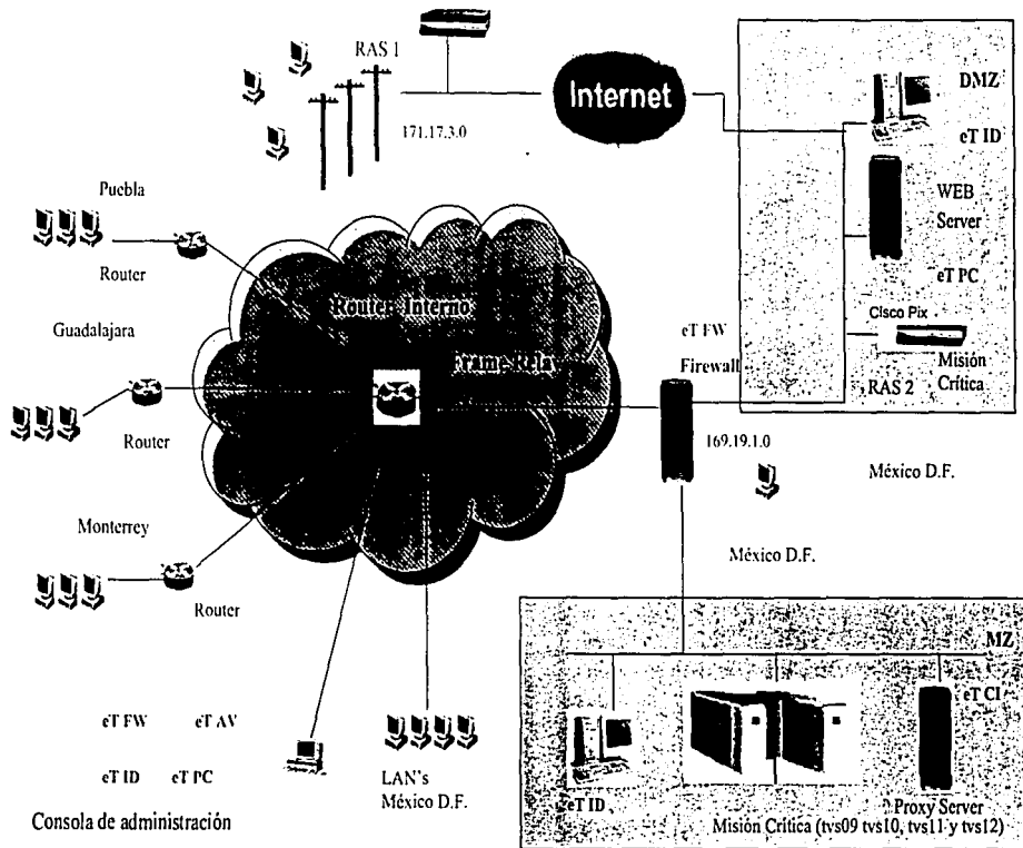
Figura 4.4. Arquitectura del Sistema de Seguridad
