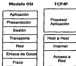
Figura 1.4. Comparación del Modelo OSI y TCP/IP.
