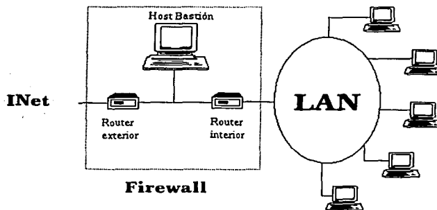
Figura 2.2. Arquitectura DMZ.
