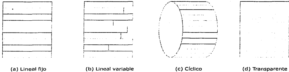
Figura 3.9 Estructuras de archivos de una TI (a,b,c,d)
