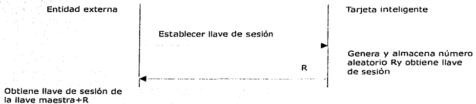
Figura 3.18 Proceso de obtención de una llave de sesión
