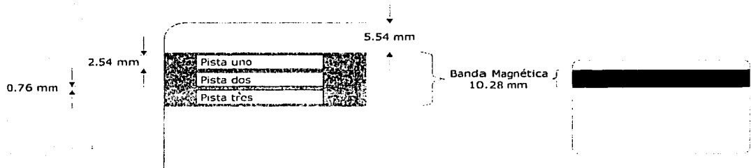
Figura 2.1 Sub-bandas de una tarjeta magnética
