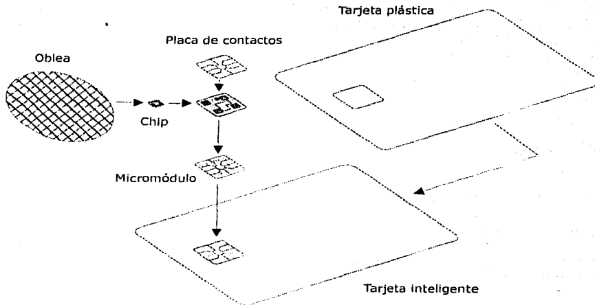
Figura 2.17 Esquema de la fabricación de la tarjeta inteligente
