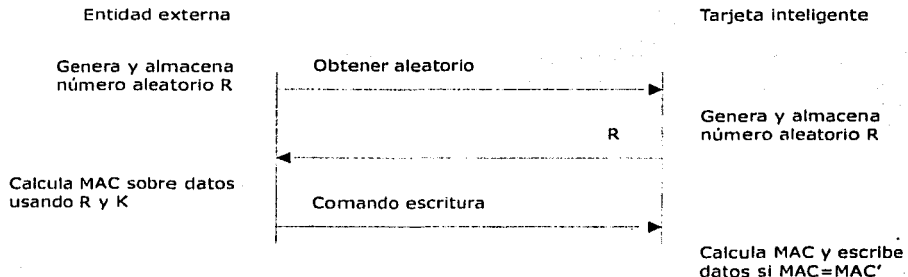
Figura 3.15 Operación de escritura en modo protegido
