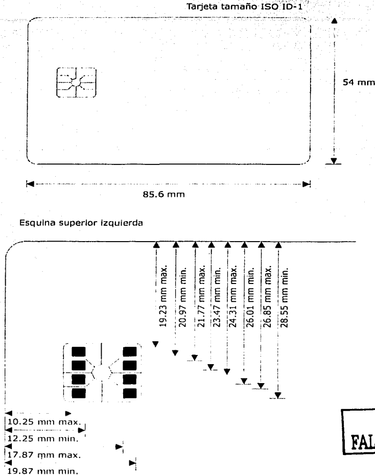
Figura 2.12 Dimensiones de la tarjeta inteligente y posición de los contactos
