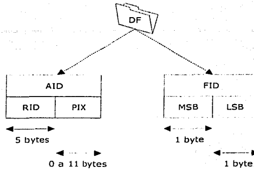
Figura 3.8 Identificadores de un archivo DF
