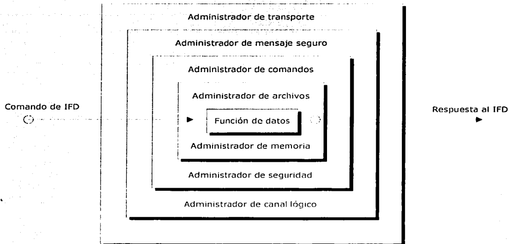
Figura 3.2 Estructura del sistema operativo de una tarjeta inteligente.
