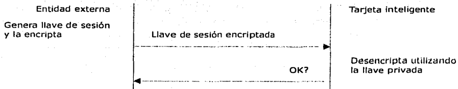
Figura 3.19 Proceso de obtención de una llave de sesión utilizando la llave pública
