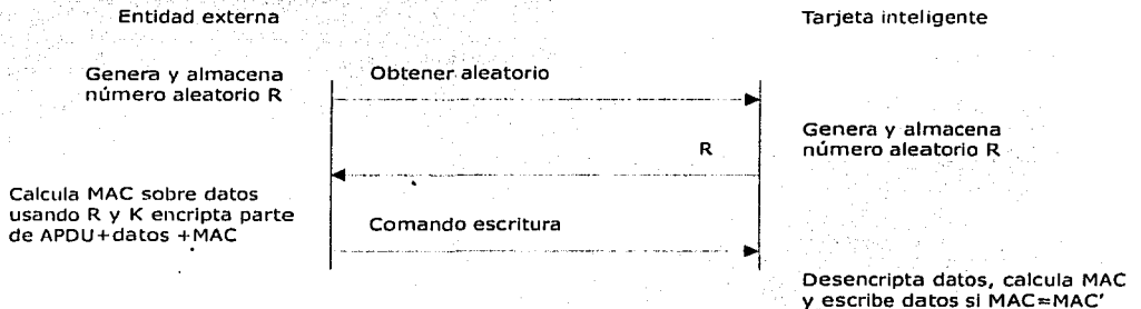
Figura 3.17 Operación de escritura en modo protegido y encriptado
