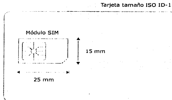
Figura 5.5 Esquema del módulo SIM
