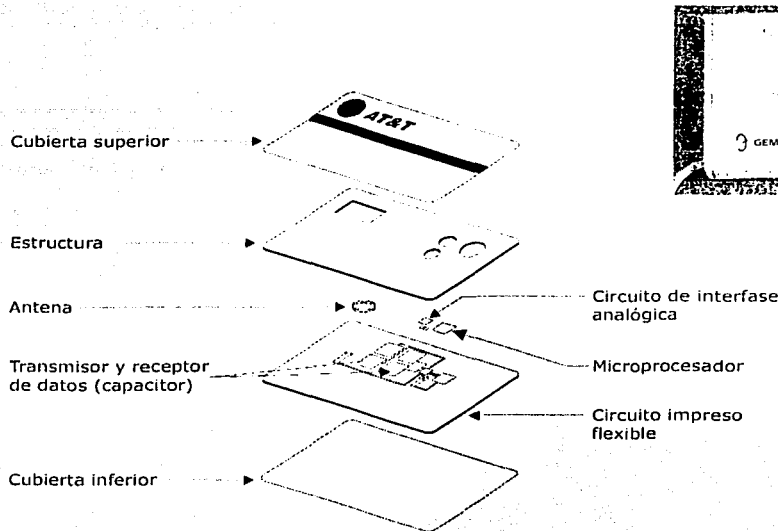
Figura 2.10 Tarjeta y lector sin contactos
