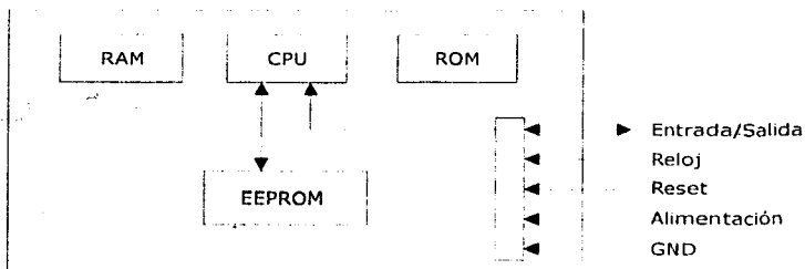
Figura 2.7 Arquitectura de una tarjeta con microprocesador
