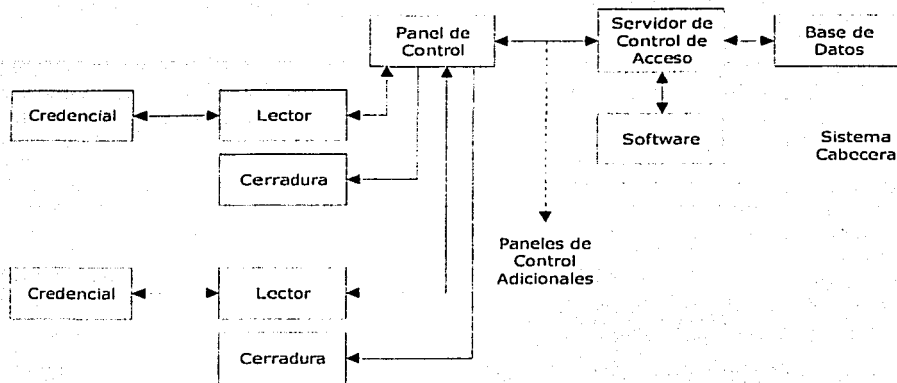
Figura 5.2 Esquema del sistema de control de acceso
