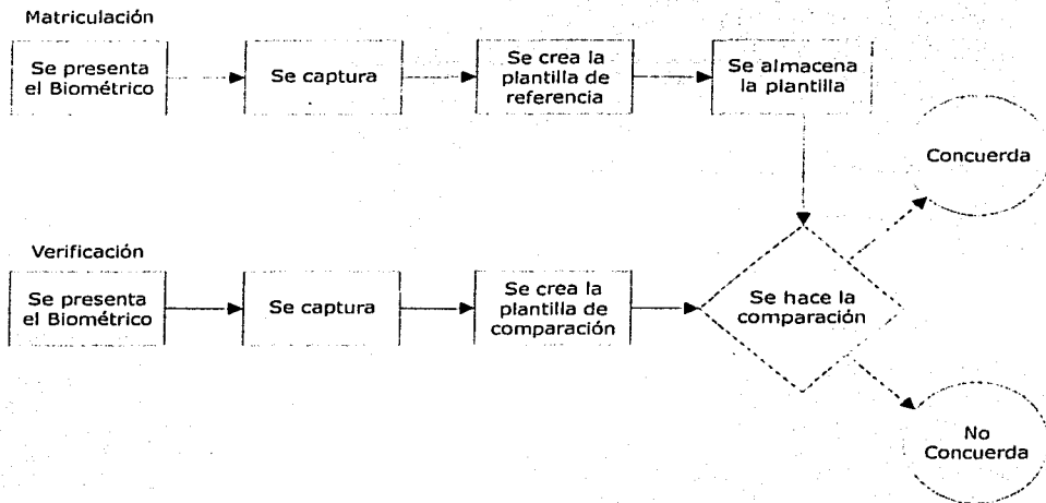
Figura 5.3 Proceso de comparación biométrica
