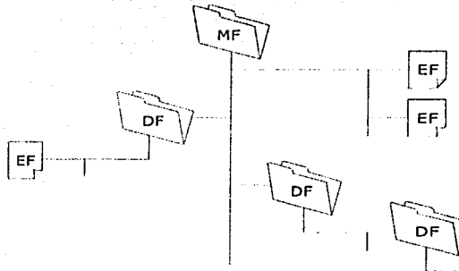
Figura 3.6 Tipos de archivos de una TI
