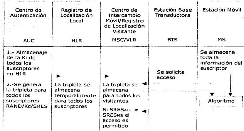
Figura 5.10 Procedimiento de autenticación
