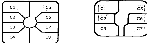
Figura 2.13 Configuración de los contactos
