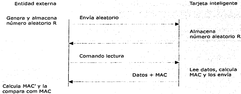
Figura 3.14 Operación de lectura en modo protegido
