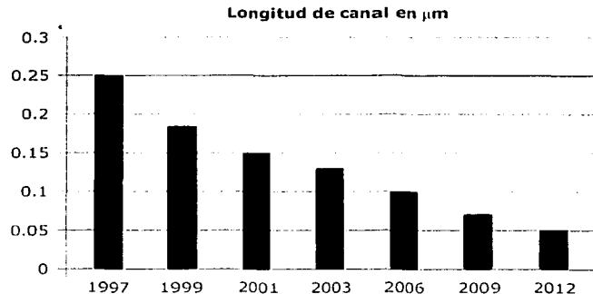
Figura 1.1 Reducción de la longitud de canal (Fuente: Intel)
