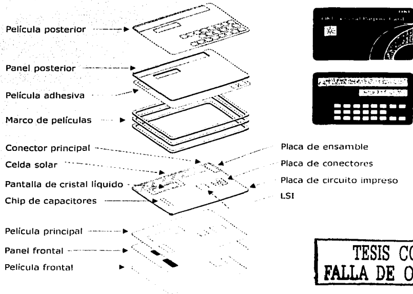
Figura 2.8 Esquema de una Super Smart Card
