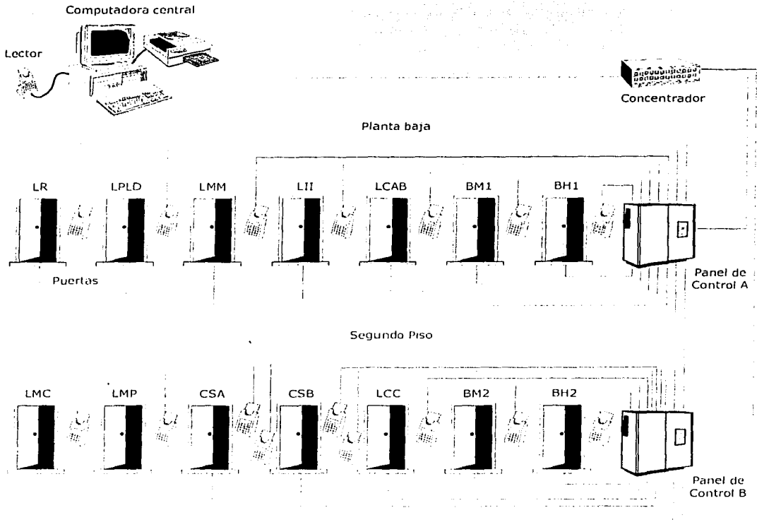
Figura 6.7 Diagrama del Sistema de Control de Acceso
