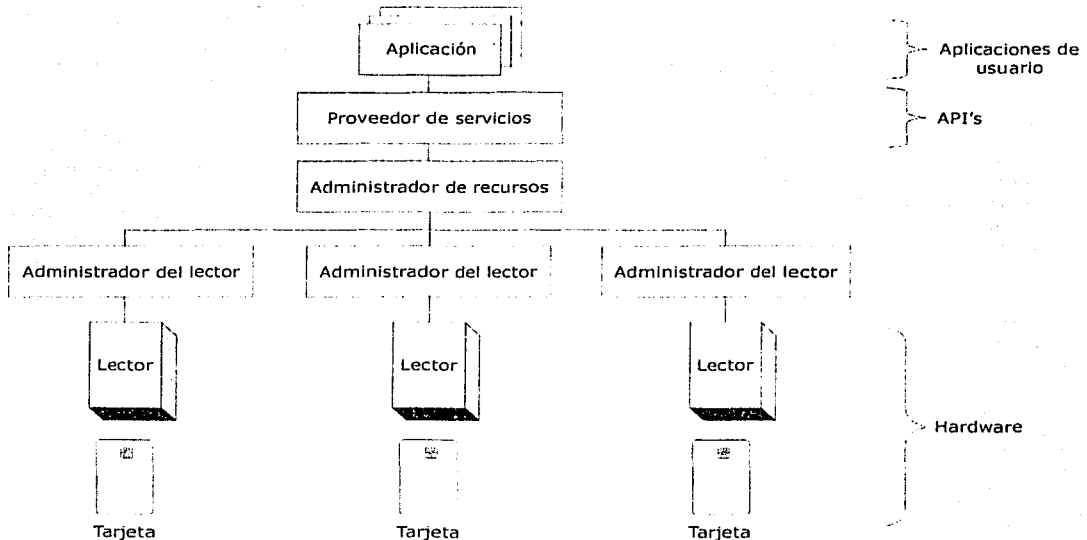
Figura 3.20 Arquitectura general del estándar PC/SC.
