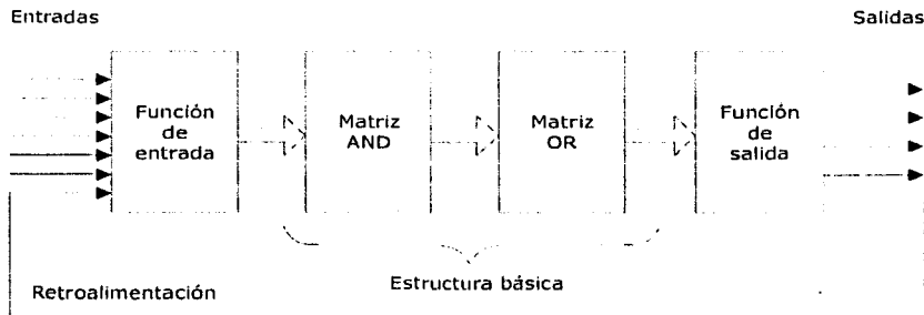
Figura 1.7 Estructura General de un PLD
