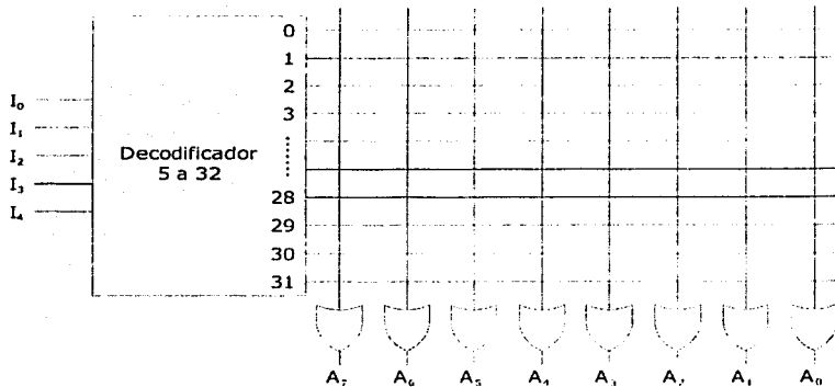
Figura 1.8 Lógica interna de una ROM de 32 x 8
