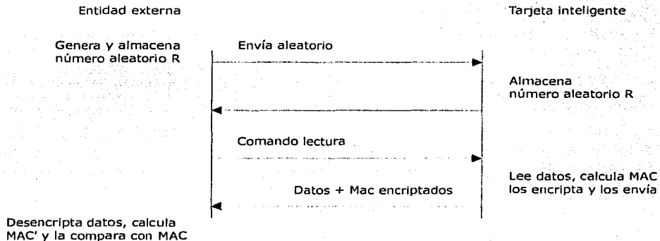
Figura 3.16 Operación de lectura en modo protegido y encriptado
