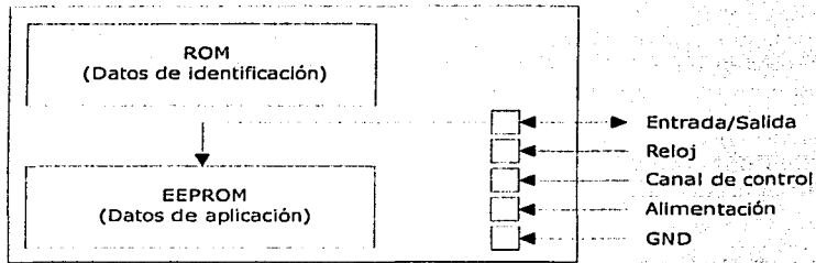
Figura 2.6 Esquema de bloques para una tarjeta de memoria
