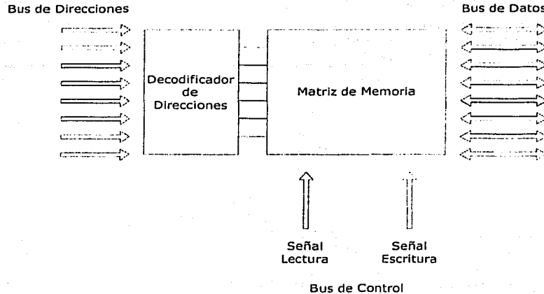
Figura 1.4 Diagrama de bloques de una memoria
