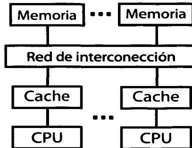
Figura 1.2: Estructura de los multiprocesadores de memoria compartida.
