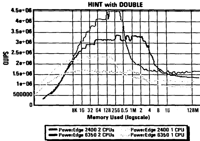
Figura 3.1: Curvas HINT de PowerEdge 2400 Dell y servidores 6350.
