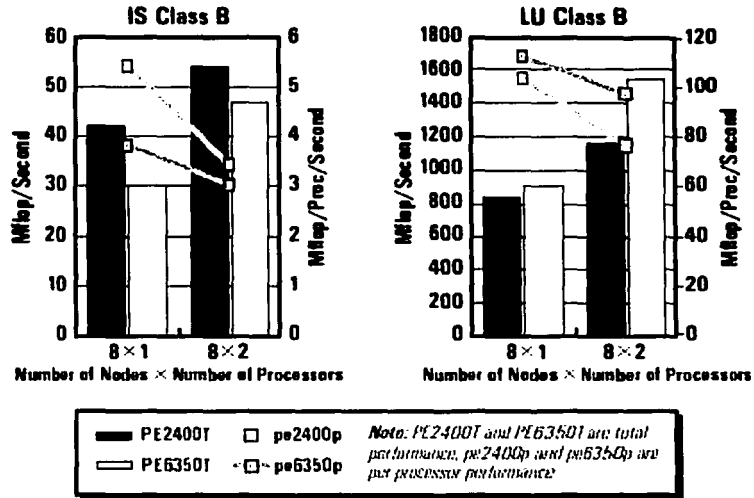
Figura 3.3: Desempeño de programas LU e IS de NPB sobre dos Cluster Beowulf Dell
