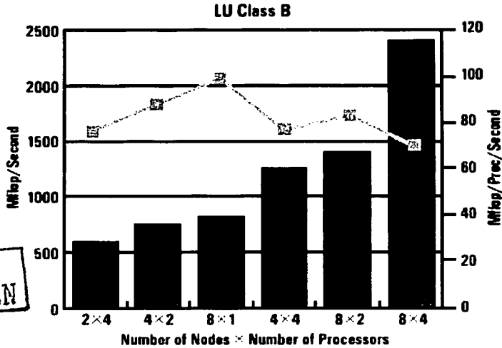
Figura 3.2: Desempeño de un programa LU.
