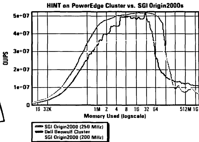
Figura 3.10: HINT sobre un Cluster Beowulf Dell y SGI Origin2000s.
