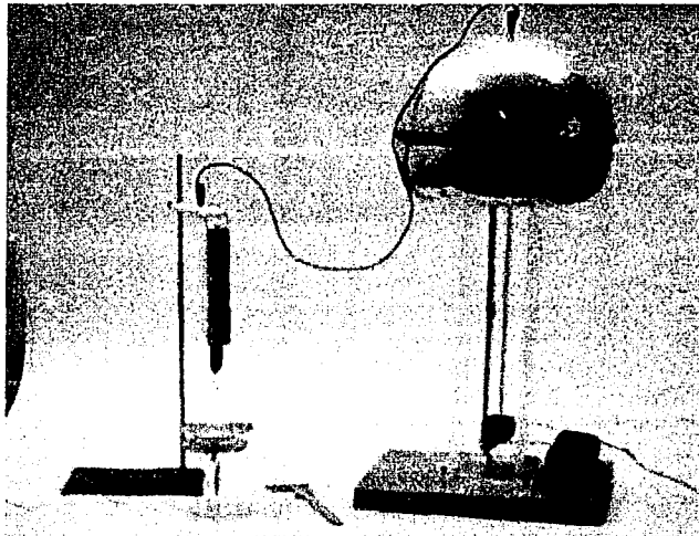
Fig 17. La figura muestra dos platos capacitivos, separados entre sí, uno de ellos se encuentra conectado al generador y está sujeto de un dinamómetro, y el otro, está conectado a Tierra
