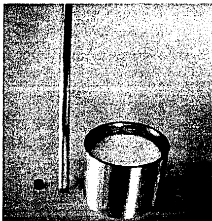
Fig. 34. Tubo de aluminio con imán y lámpara.
