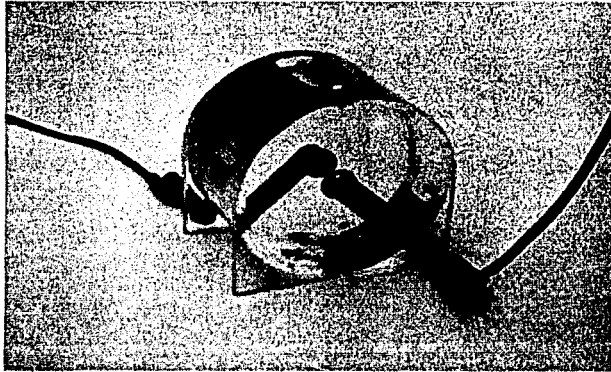
Fig 8. Caja de acrílico con electrodos esféricos
