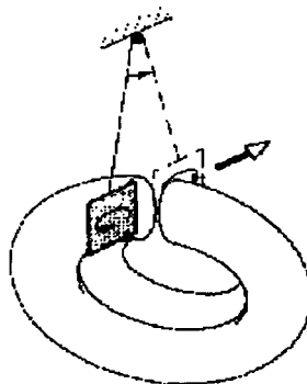
Fig 31 Placa de aluminio que oscila en forma pendular entre los polos de un imán, debido a las corrientes parásitas en la misma.
