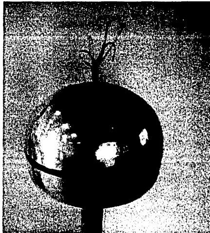
Fig.2. Conector con hilos de estambre, colocado en la parte superior del Generador Van de Graaff
