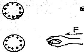
Fig 11. En la figura se muestra el trabajo que se tiene que realizar para vencer la fuerza repulsiva entre las cargas del mismo signo.
