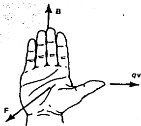
Fig 18. Se muestra la regla de la mano derecha, que indica la dirección del vector de fuerza magnética, en función de los vectores B y qv .
