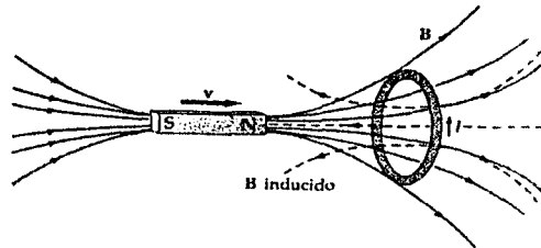
Fig.27. Imán de barra acercándose a un conductor
