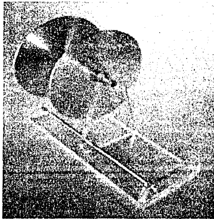
Fig 16. Capacitor variable con movimiento que permite variar el área entre las placas
