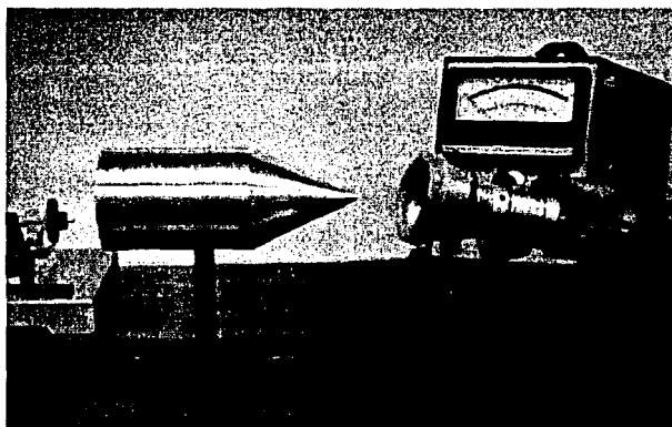
Fig 6: Conductor cónico con electrómetro
