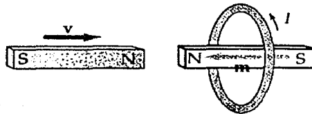
Fig 28. Se muestra la fuerza magnética que aparece en la espira, de tipo repulsiva, debido a la dirección de la corriente que circula a través de ella, y que se puede comprobar con la regla de la mano derecha.
