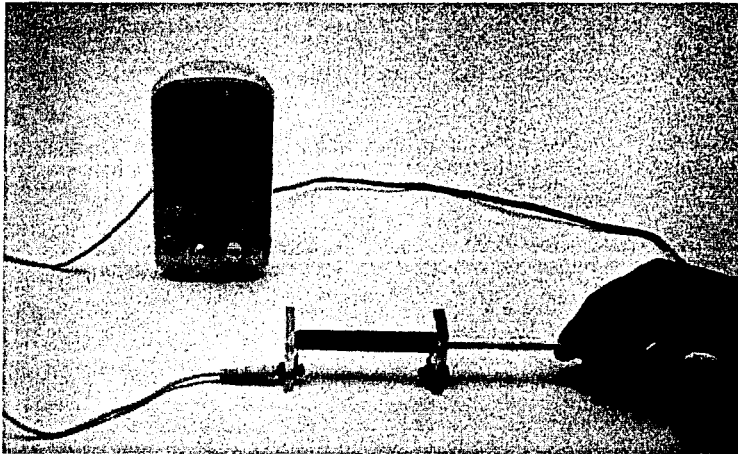
Fig.27. Experimento de Barkhausen
