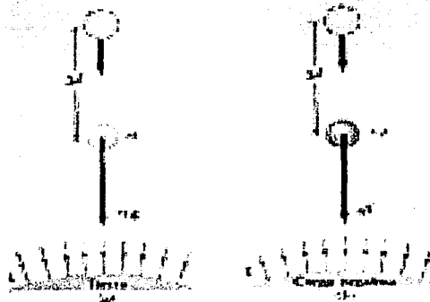
.Fig 10. En la figura se muestra la analogía entre la energía potencial gravitatoria y la energía potencial electrostática
