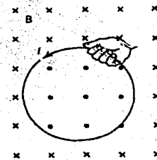
Fig. 19. Regla de la mano derecha para conductores de corriente
