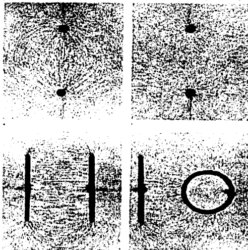
Fig 7. Se muestran en la figura, algunos patrones de campo eléctrico debidos a distintas configuraciones geométricas
