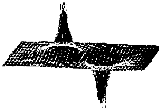
Fig.13. Se muestra en la figura una reconstrucción tridimensional del caso mostrado líneas arriba., para una carga positiva y otra negativa.
