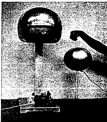
Fig 4: Partículas de confetti entre dos esferas conductoras.
