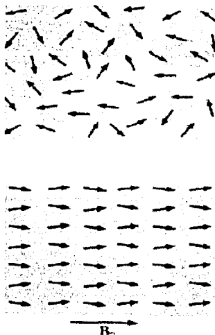
Fig 22. La primera figura muestra la orientación aleatoria de los dominios, en ausencia de magnetización, la segunda muestra la alineación de los dominios ante la magnetización.
