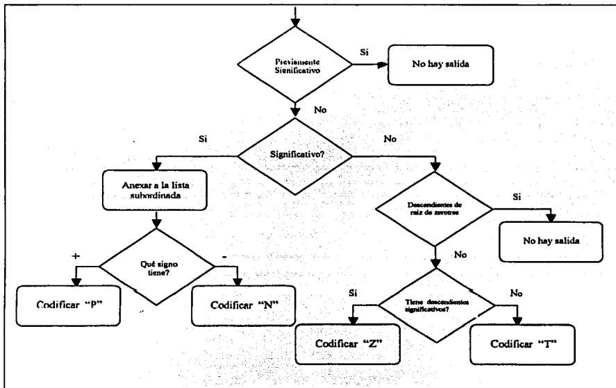
Figura 4.6 Diagrama de bloques del paso dominante
