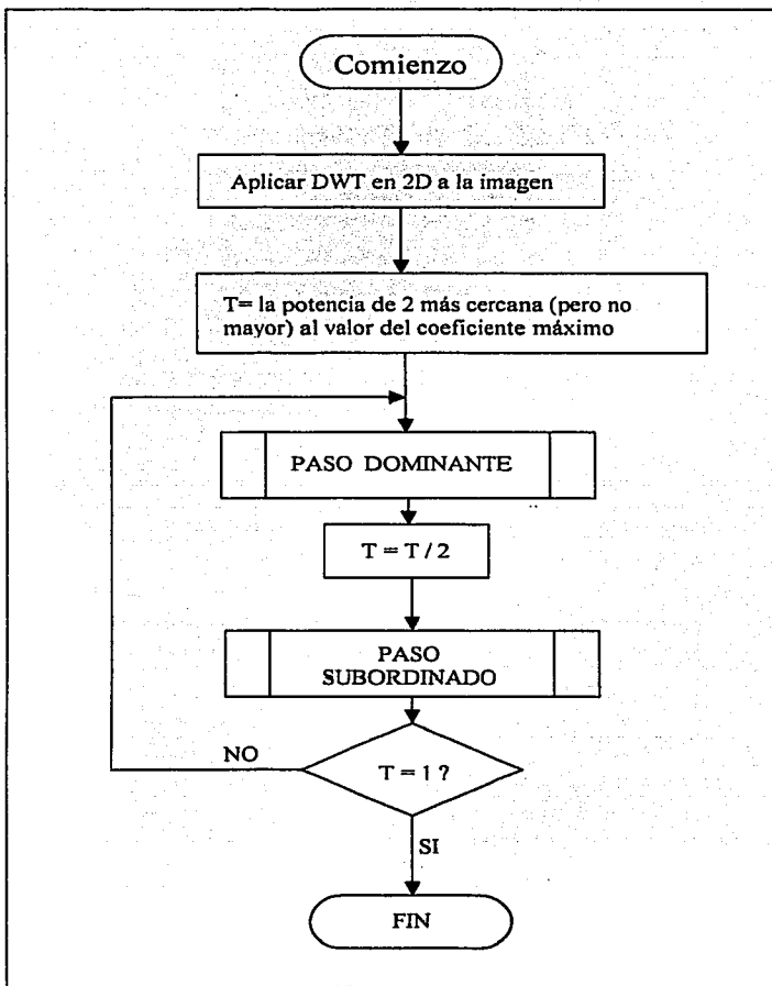
Figura 4.5 Diagrama de bloques del EZW
