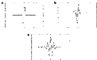
Figura 3.1.(a) Wavelet de Haar, (b) Wavelet de Daubechies, (c) Wavelet de Morlet.
