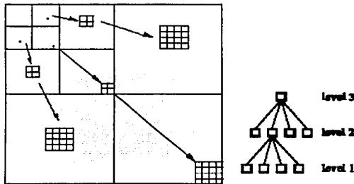
Figura 4.1 Estructura zerotree
