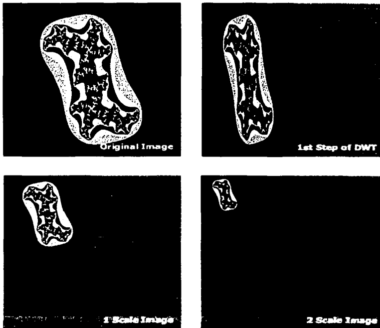
Figura 3.7 DWT en dos dimensiones
