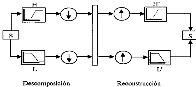
Figura 3.4. Esquema wavelet (Descomposición y reconstrucción)
