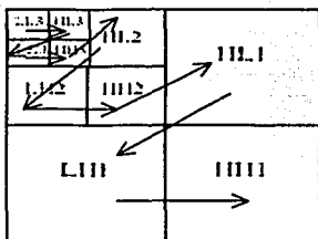
Figura 4.3 Disposición de los coeficientes wavelet de tres escalas
