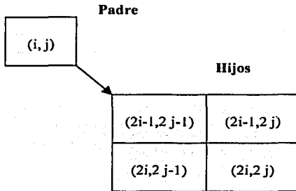
Figura 4.2 Localización de los coeficientes hijos con respecto al padre
