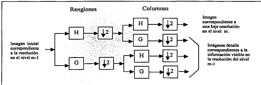
Figura.3.5 Diagrama de la DWT directa para una imagen
