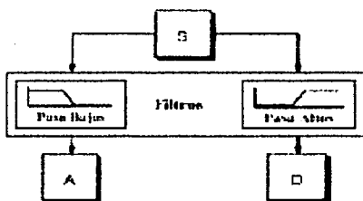
Figura 3.2. Diagrama de descomposición de señales
