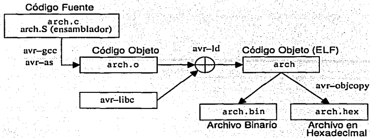
Figura 4.2: Proceso de compilación con la cadena de herramientas de desarrollo de GNU para los microcontroladores AVR.
