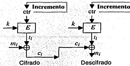
Figura 2.5: Diagrama del modo Contador.
