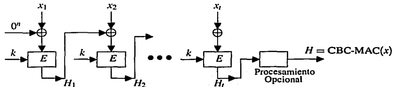
Figura 2.10: Obtención del CBC-MAC para un mensaje x = x_1|x_2|\dots|x_i
