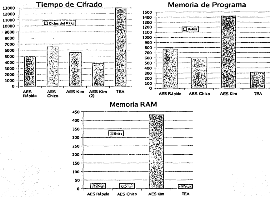
Figura 5.1: Gráficas comparativas para las implantaciones que funcionan sobre un microcontrolador de la familia AVR. Para AES Kim (2) no contamos la expansión de clave.
