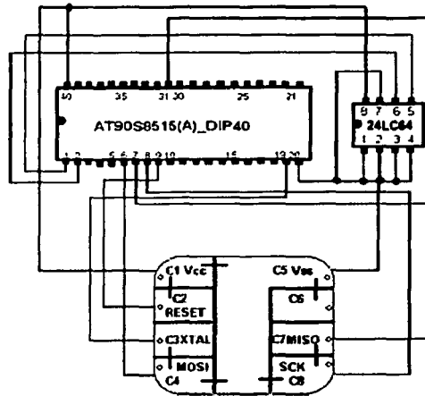
Figura 4.8: Esquema representativo de la interconexión del microcontrolador, la memoria y los contactos para la tarjeta Fincard 2 . Imagen tomada de [8].
