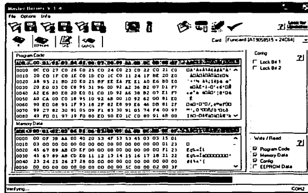
Figura 4.6: Master Burner verificando la programación de la tarjeta después de cargar SOSSE en ella.
