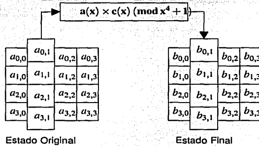
Figura 3.4: Representación del paso MixColumns para uno de los renglones del estado.
