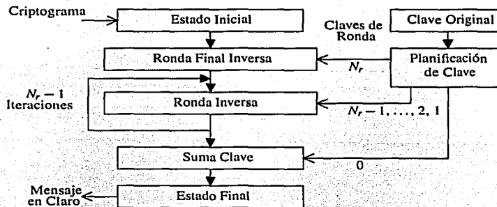
Figura 3.7: Diagrama del algoritmo de descifrado.
