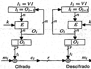
Figura 2.4: Diagrama del modo OFB.
