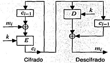
Figura 2.2: Diagrama del modo CBC .
