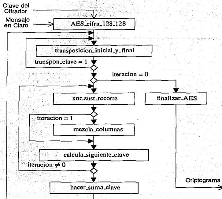
Figura 4.3: Esquema del flujo del programa en ensamblador con los bloques más importantes.
