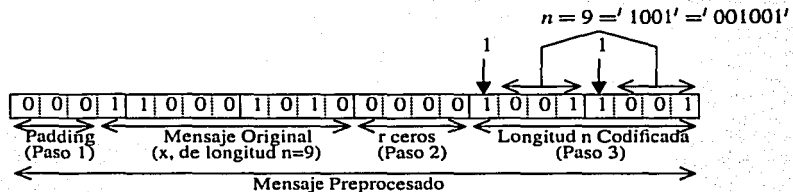
Figura 2.9: Preprocesamiento de la cadena x = "10001010" para obtener su hash. r = 4 .
