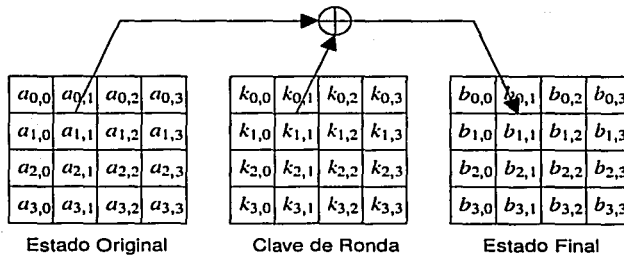
Figura 3.5: Representación del paso AddRoundKey enfatizando la transformación de un byte del estado.
