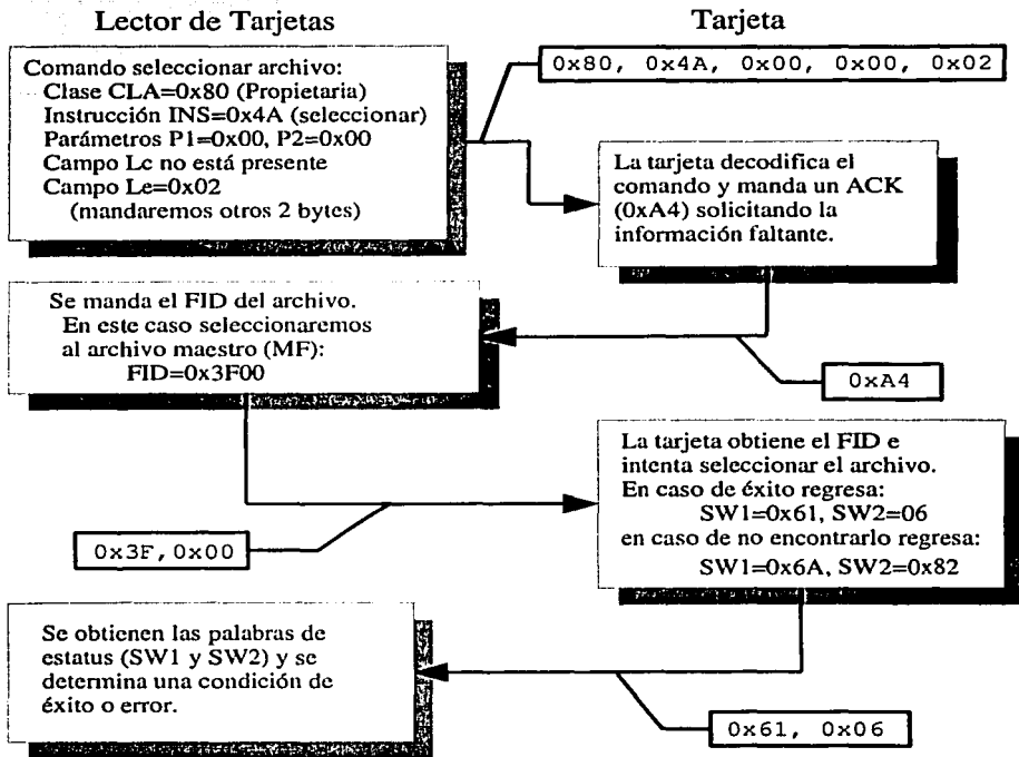
Figura 1.3: Comunicación entre el lector y la tarjeta al seleccionar un archivo.
