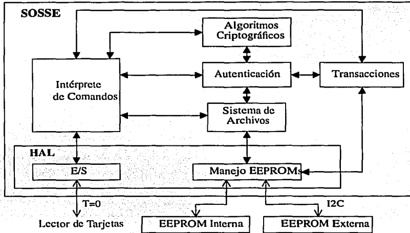
Figura 4.4: Esquema representando los flujos de datos más importantes en SOSSE .
