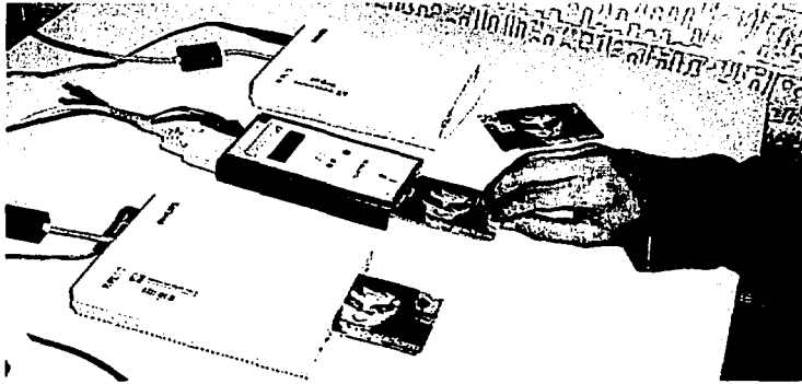
Figura 4.5: El programador de tarjetas (centro) y los lectores de tarjetas (arriba y abajo).
