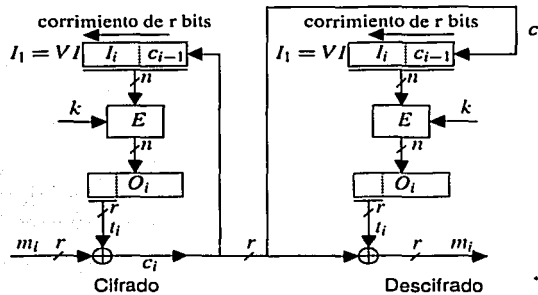
Figura 2.3: Diagrama del modo CFB.
