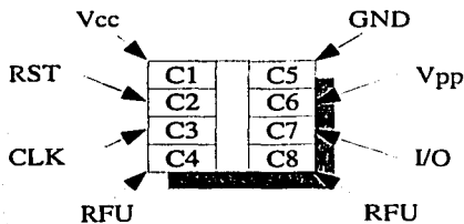
Figura 1.1: Disposición y función de los contactos de acuerdo a ISO 7816-2 .
