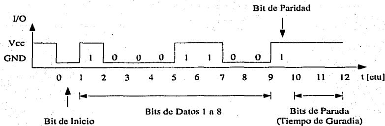
Figura 1.2: Transmisión del byte "00110001" o 0x31 siguiendo la convención directa.
