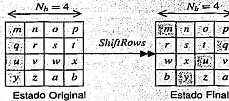
Figura 3.3: Paso ShiftRows para el AES.
