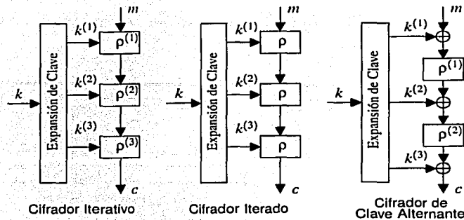
Figura 2.6: Tres tipos de cifradores de bloques.
