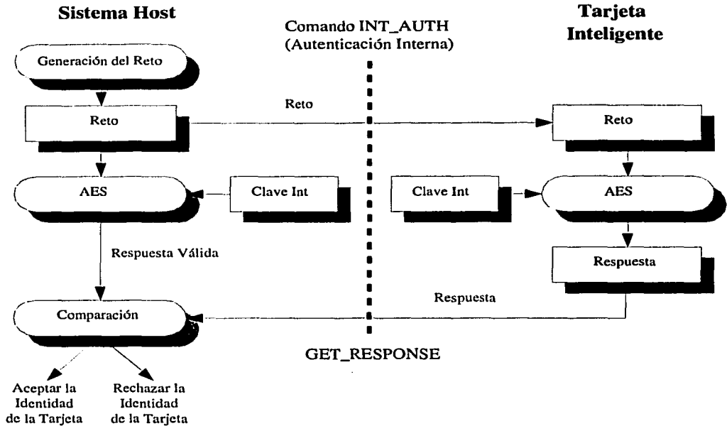
Figura 4.10: Diagrama que muestra el protocolo de autenticación de la tarjeta con el host .
