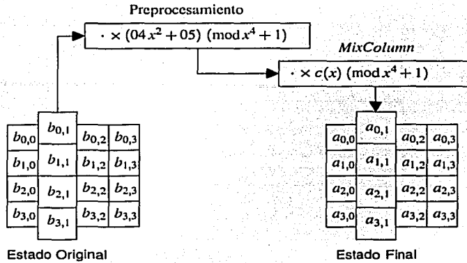
Figura 3.9: Paso InvMixColumns realizado mediante un preprocesamiento y la transformación MixColumn .
