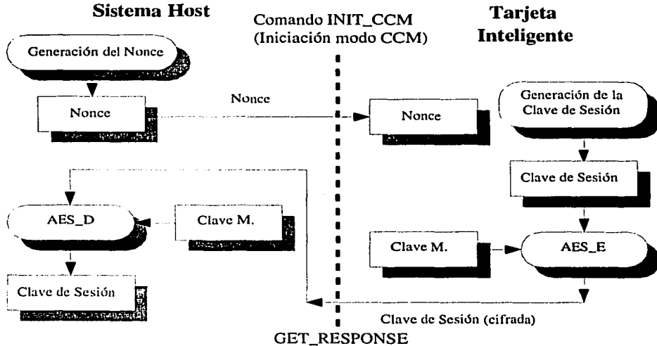
Figura 4.11: Generación e intercambio de la clave de sesión y el nonce mediante el comando INIT_CCM .
