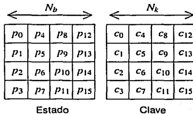
Figura 3.1: Disposición del estado inicial ( N_b = 4 ) y de la clave del cifrador ( N_k = 4 ).
