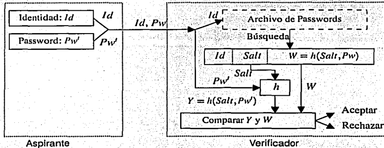
Figura 2.11: Esquema de la autenticación débil incorporando una función unidireccional h y un salt .
