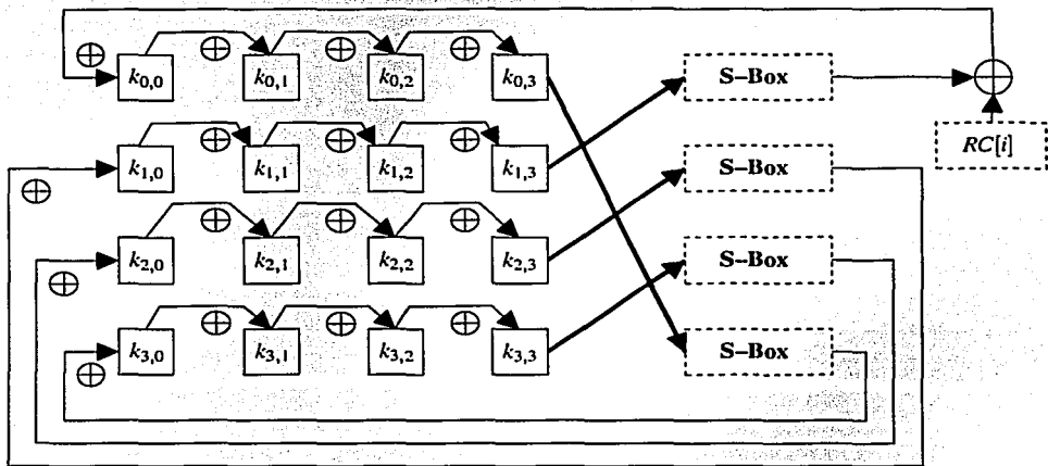
Figura 3.6: Transformación de la clave de ronda i - 1 en la clave de ronda i . (Ver las notas para entender el significado del diagrama).
