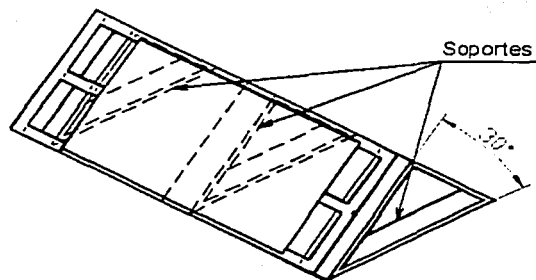
Figura 4.4 Estructura de soporte.
