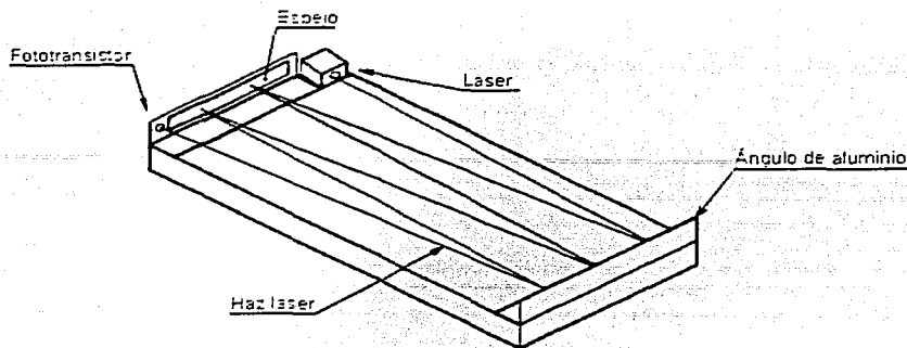
Figura 3.11 Plataforma con sistema mono-láser.
