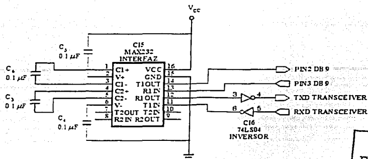
Figura 5.3 Interfaz MAX232 con el transceiver.
