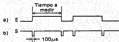
Figura 4.15 a) Señal proveniente de los sensores; b) Señal de salida de la interfaz generadora de pulsos.
