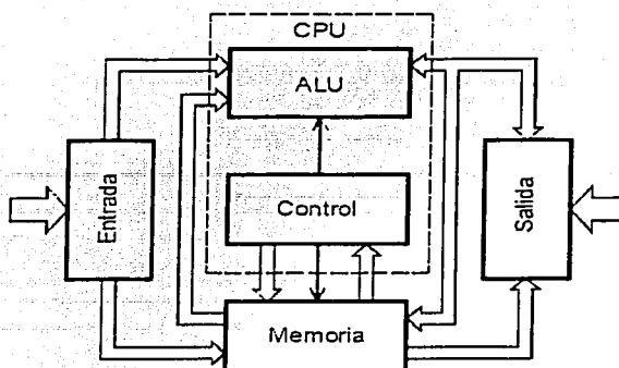
Figura 2.4 Diagrama general de un microcontrolador.
