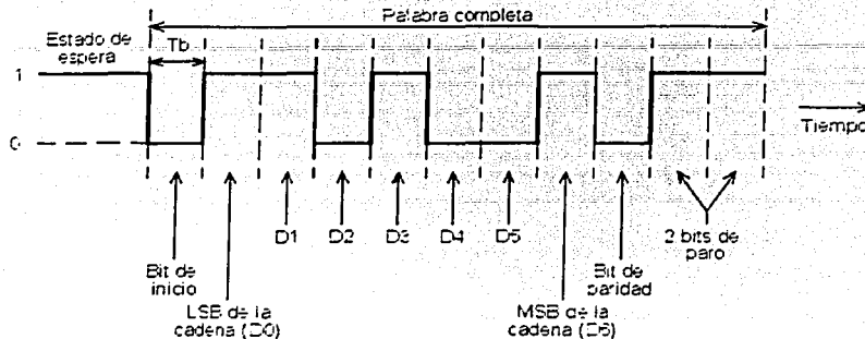
Figura 2.6 Transmisión serial de datos.
