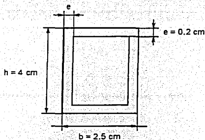
Figura 4.3 Sección transversal de la solera.
