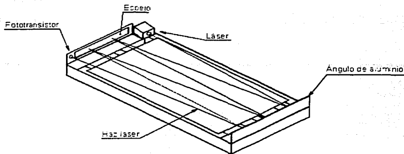
Figura 4.5 Imagen completa de la plataforma diseñada.
