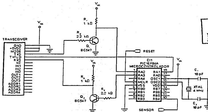
Figura 5.2 Conexión entre el PIC y el transceiver.
