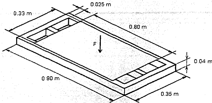
Figura 4.1 Estructura de la plataforma de medición.
