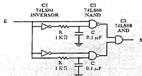
Figura 4.14 Interfaz para adecuar la señal de entrada del Precision Timer.
