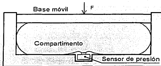
Figura 3.7 Plataforma con sensor de presión.
