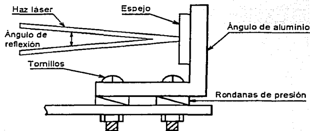
Figura 4.6 Mecanismo de calibración de la posición vertical de incidencia del haz láser.
