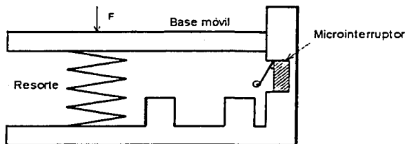
Figura 3.3 Plataforma con microinterruptor.
