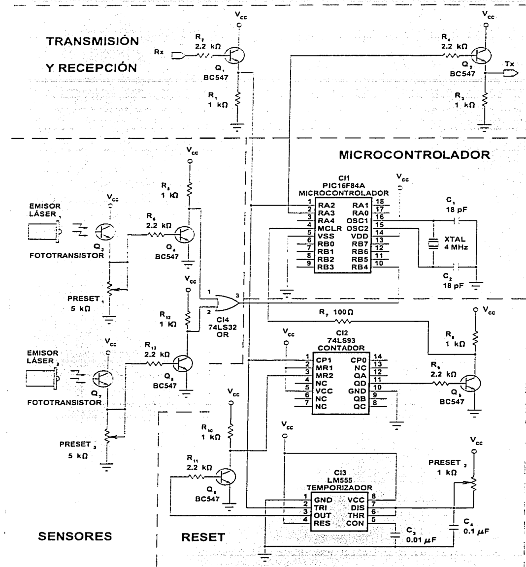
Figura 4.9 Diagrama general del circuito electrónico.
