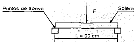
Figura 4.2 Barra de solera con dos puntos de apoyo sometida a una fuerza central.
