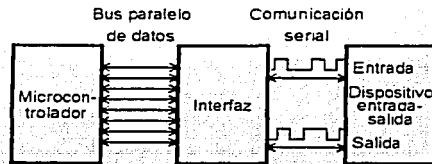
Figura 2.5 Comunicación serial entre un microcontrolador y un dispositivo externo.
