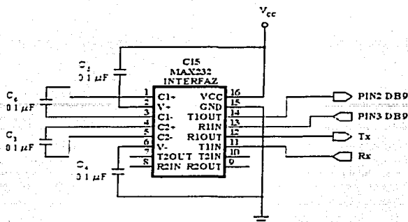
Figura 4.12 Interfaz MAX232C.
