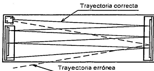
Figura 4.7 Mecanismo de calibración de la posición horizontal de incidencia del haz láser.
