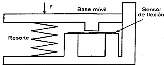
Figura 3.5 Plataforma con sensor de flexión.
