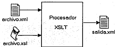
Figura 2.9 Procesador XSLT
