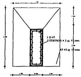
PLANTA s/e ZAPATA Z3 ZAPATA AISLADA s/e
