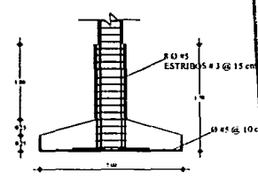
CONCRETO f_c = 250 \text{ KG/CM}^2 ALZADO ZAPATA Z1 ZAPATA AISLADA s/e
