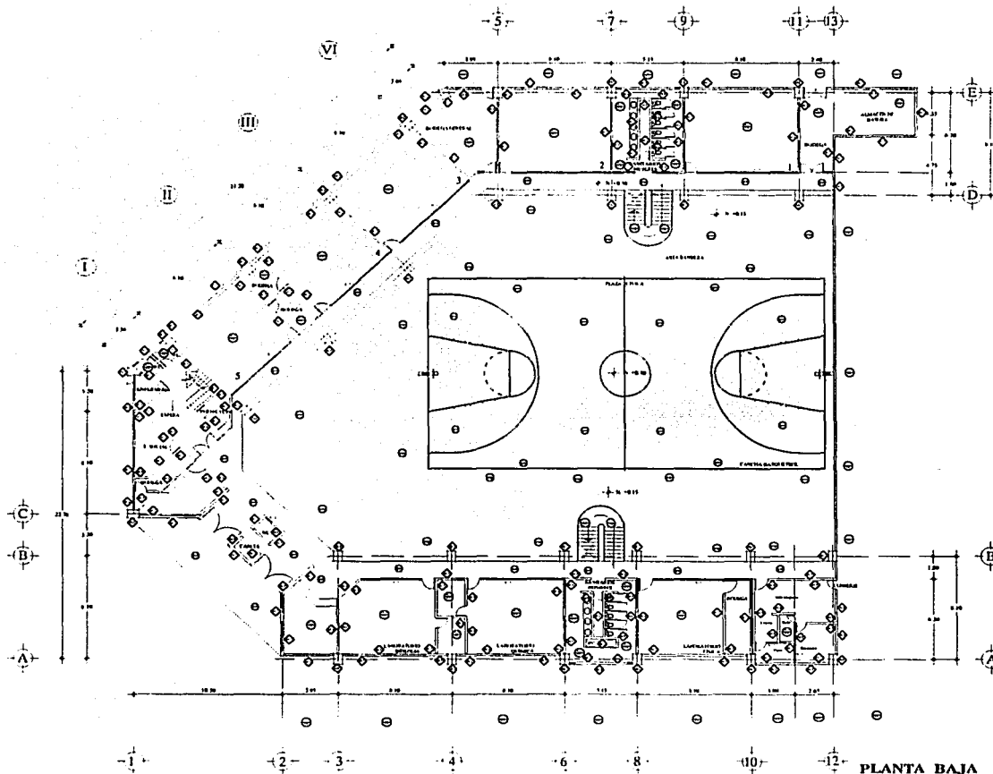
PLANTA BAJA ACABADOS
