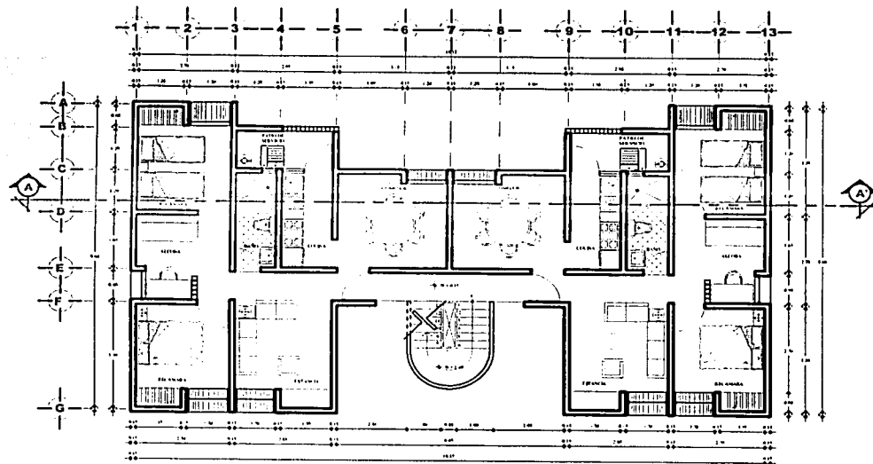
PLANTA TIPO
