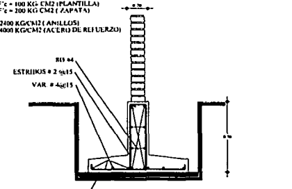
PLANTILLA DE CONCRETO f_c = 100 \text{ KG/CM}^2 ZAPATA Z2 ZAPATA CORRIDA s/e
