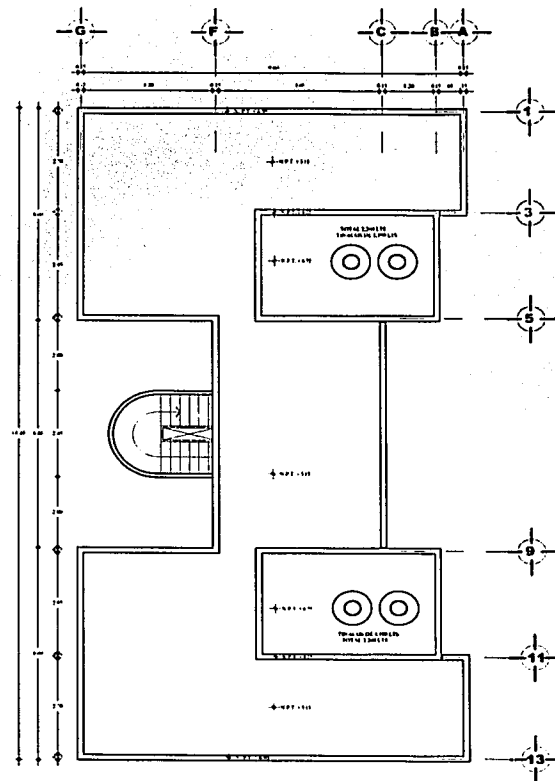
PLANTA DE AZOTEA
