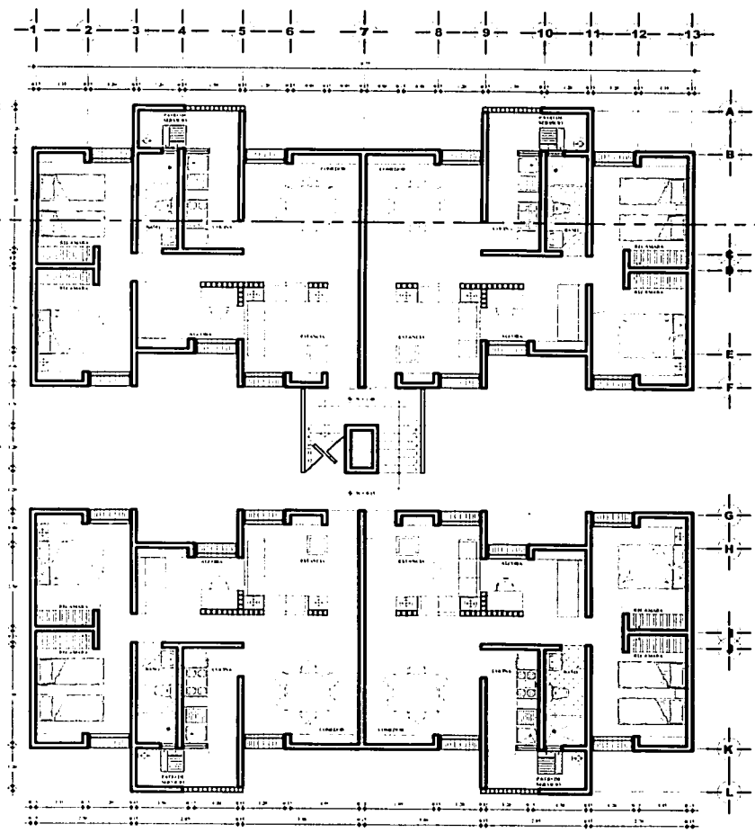
PLANTA TIPO
