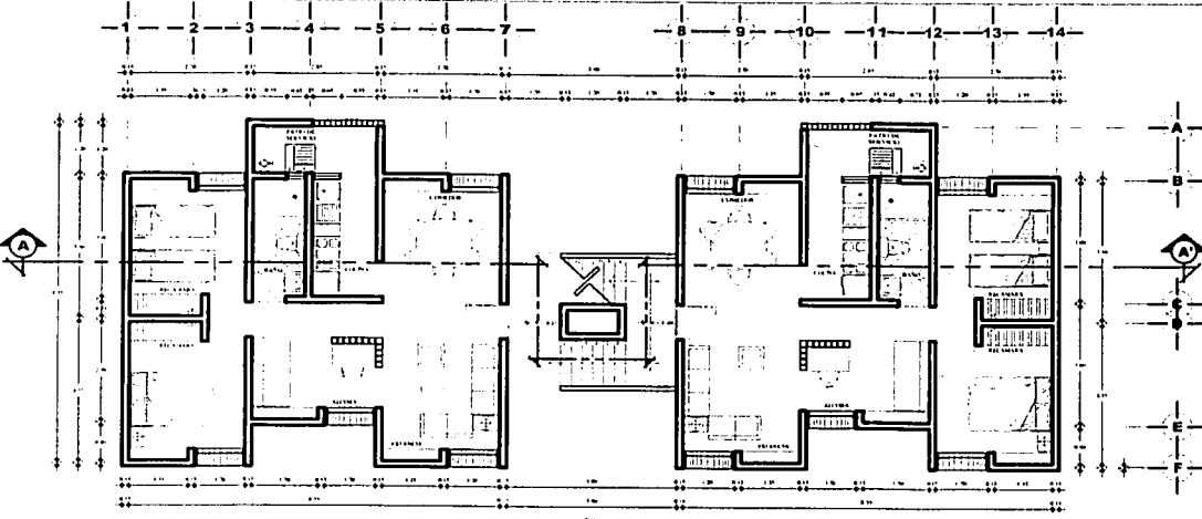
PLANTA TIPO
