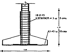
ALZADO ZAPATA Z3 ZAPATA AISLADA s/e
