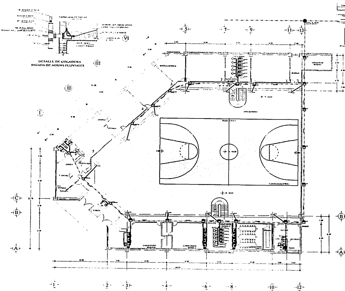
PLANTA BAJA SANITARIA
