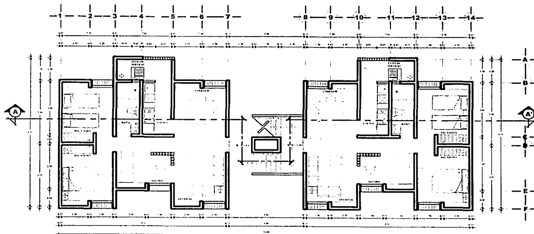
PLANTA TIPO
