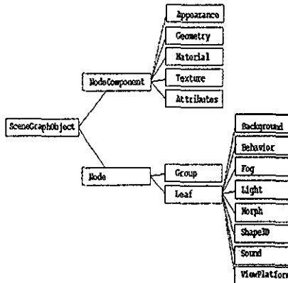
Figura 4.11: Jerarquía en la clase NodeComponent
