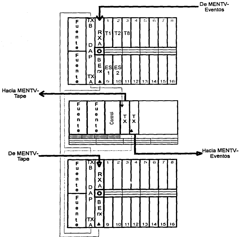
Figura 5.32. Conexiones para el equipo en MENES (anillo 1).
