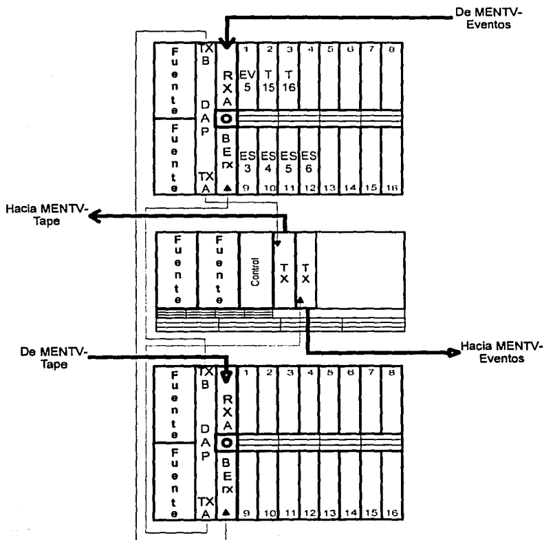
Figura 5.33. Conexiones para el equipo en MENES (anillo 2).
