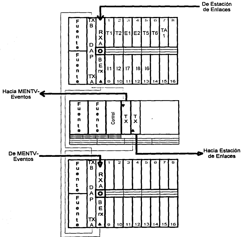
Figura 5.28. Conexiones para el equipo en INFOTV (anillo 1).
