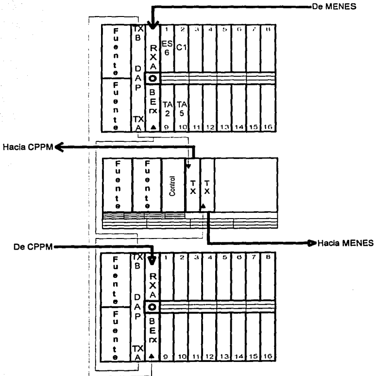
Figura 5.35. Conexiones para el equipo en MENTV-Tape (anillo 2).
