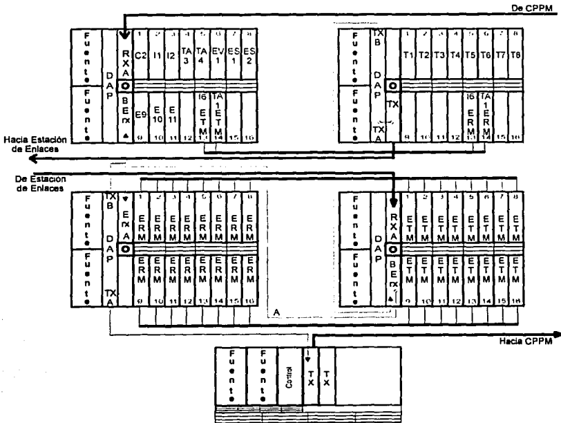
Figura 5.24. Conexiones para el equipo en Telesistema (anillo 1).
