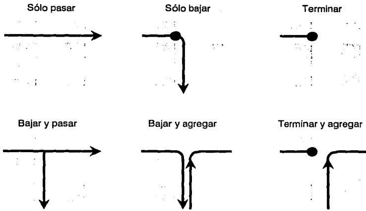
Figura 5.17. Funciones Drop/Add/Pass (bajar, agregar, pasar).
