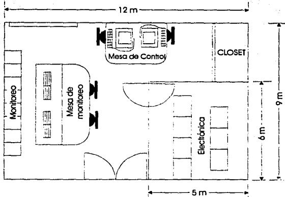
Figura 5.11. Dimensiones de Telesistema.
