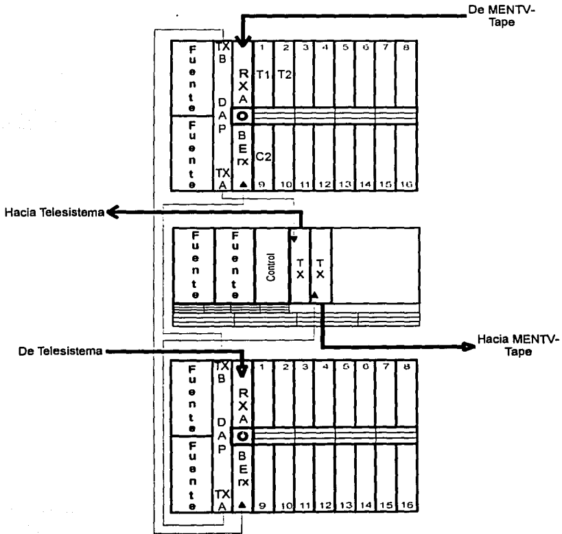
Figura 5.36. Conexiones para el equipo en CPPM (anillo 1).
