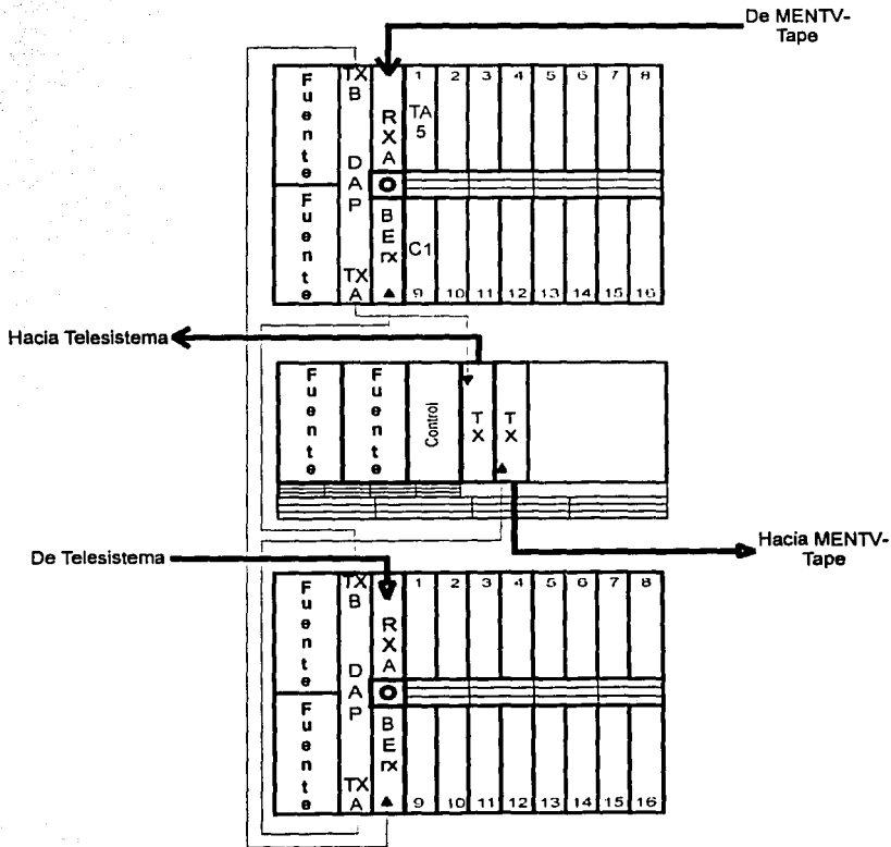
Figura 5.37. Conexiones para el equipo en CPPM (anillo 2).
