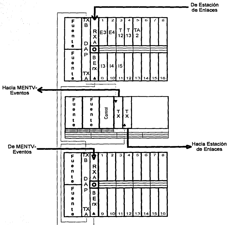
Figura 5.29. Conexiones para el equipo en INFOTV (anillo 2).
