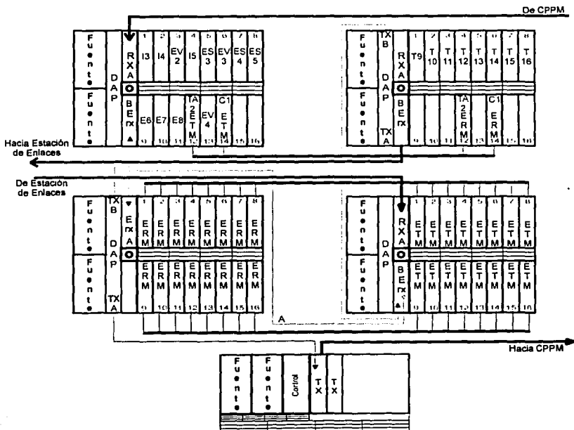
Figura 5.25. Conexiones para el equipo en Telesistema (anillo 2).
