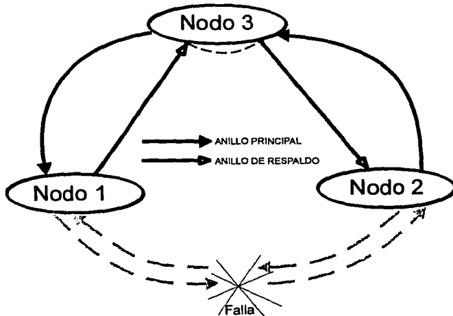
Figura 5.22. Falla entre el nodo 1 y nodo 2.
