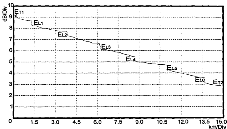
Figura 5.40. Medición de la atenuación real entre E. de Enlaces e INFOTV.
