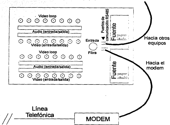
Figura 5.20. Esquema de conexión para monitoreo y control remoto.
