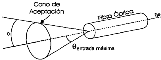
Figura 2.8. Cono de aceptación.
