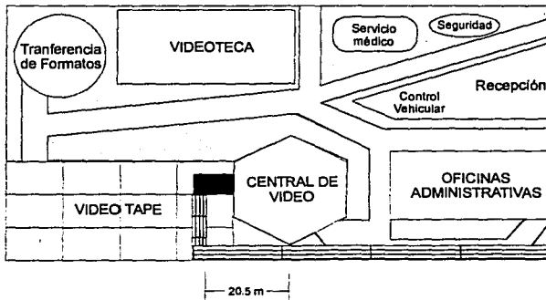
Figura 5.12. Ubicación del nodo en MENTV-Tape.
