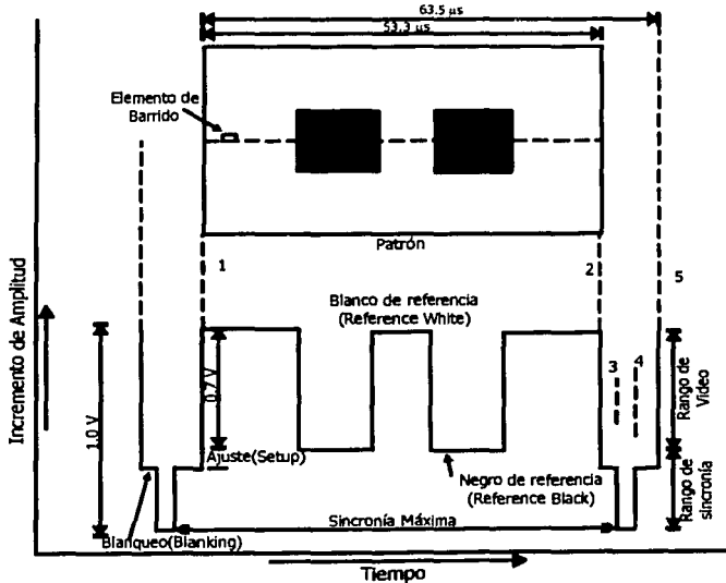
Figura 2.2. Señal de luminancia.
