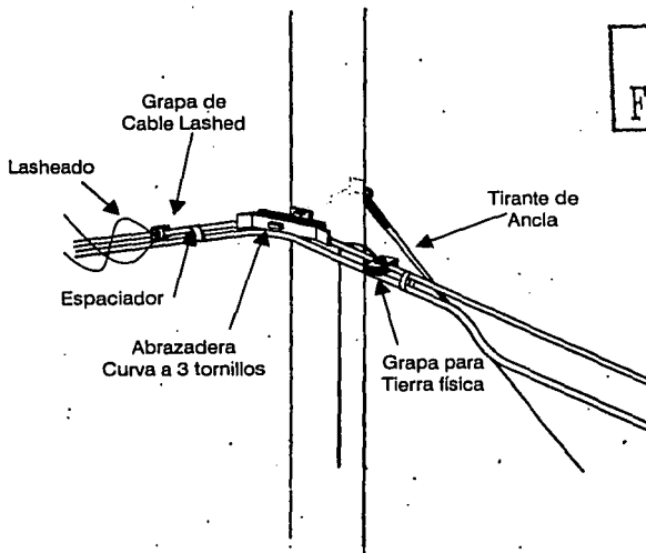
Figura 5.5. Poste con ángulo recto.
