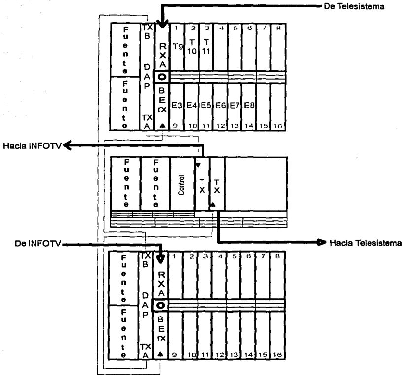
Figura 5.27. Conexiones para el equipo en Estación de Enlaces (anillo 2).
