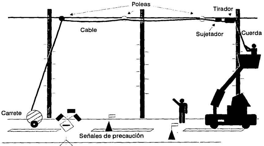
Figura 5.8. Procedimiento en tirada de cable.
