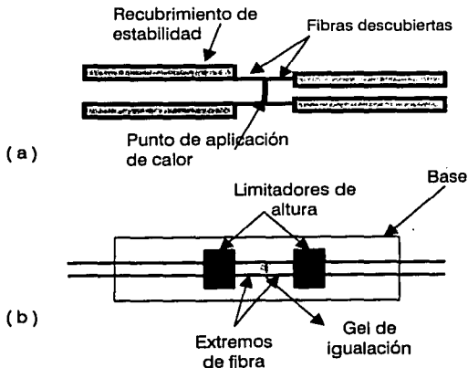
Figura 5.1. Empalmes por fusión (a) y mecánicos (b).
