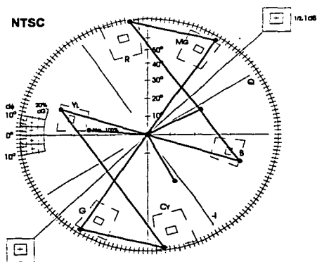
Figura 3.5. Vectorscopio mostrando un error en la ganancia y fase de la señal de crominancia.
