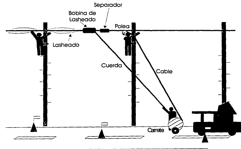
Figura 5.9. Procedimiento de "lasheado".
