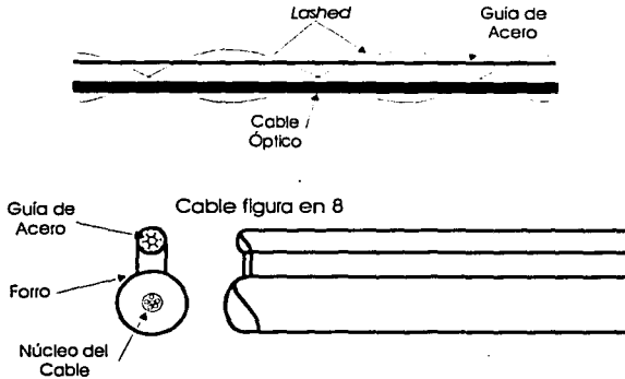
Figura 5.2. Tipos de soporte en tendidos aéreos.
