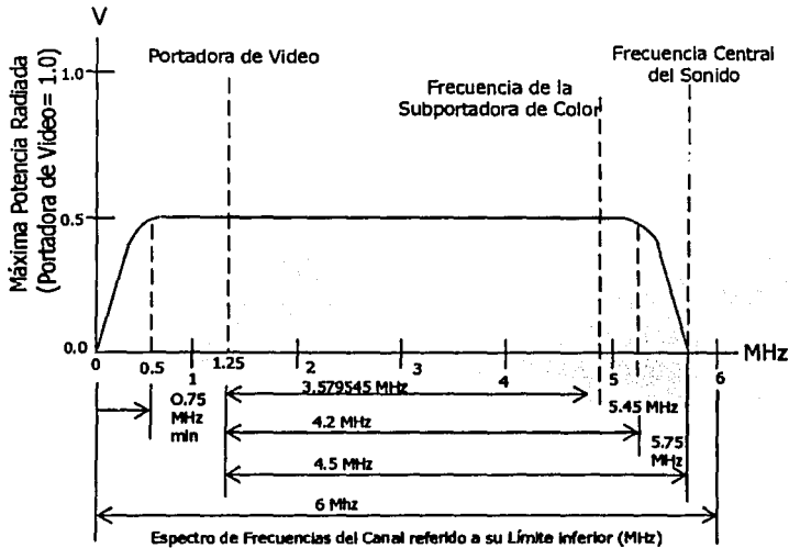
Figura 2.3. Componentes de señal de televisión.
