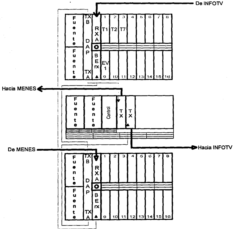
Figura 5.30. Conexiones para el equipo en MENTV-Eventos (anillo 1).
