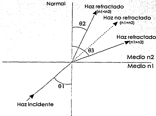
Figura 2.7. Refracción de la luz.
