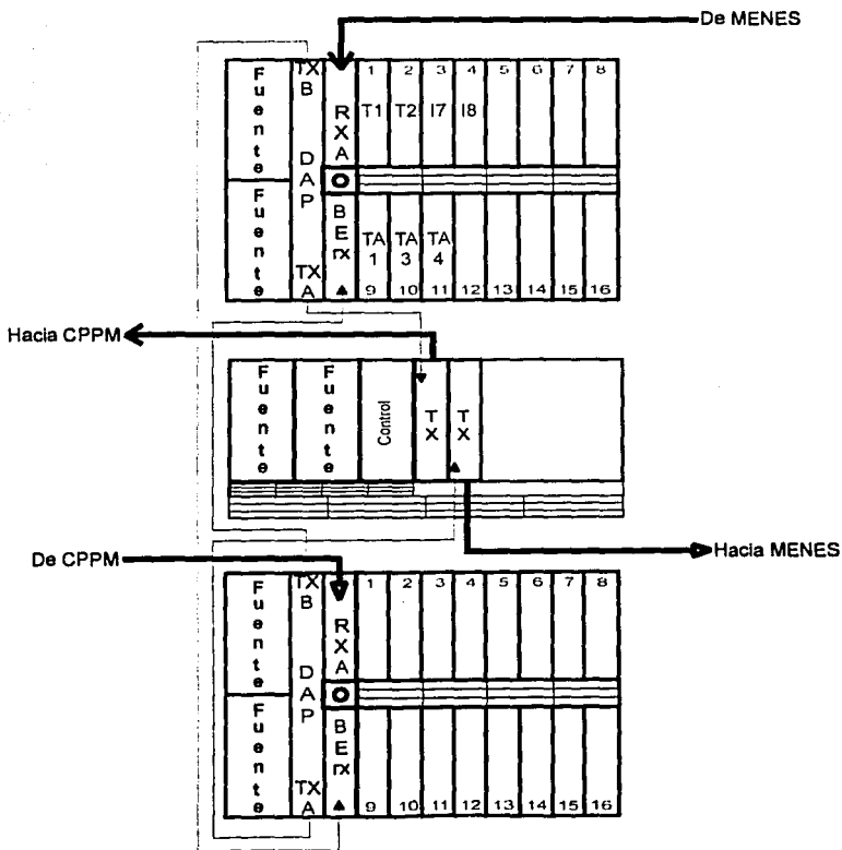
Figura 5.34. Conexiones para el equipo en MENTV-Tape (anillo 1).
