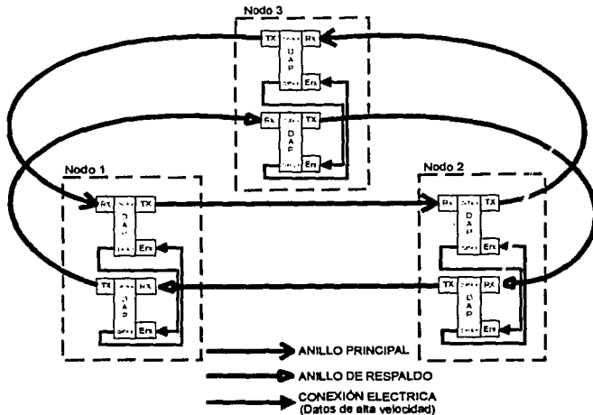
Figura 5.21. Configuración de equipos en sistema redundante.
