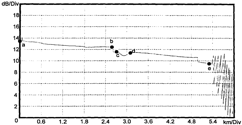
Figura 5.39. Características de medición y detección de eventos en el OTDR.
