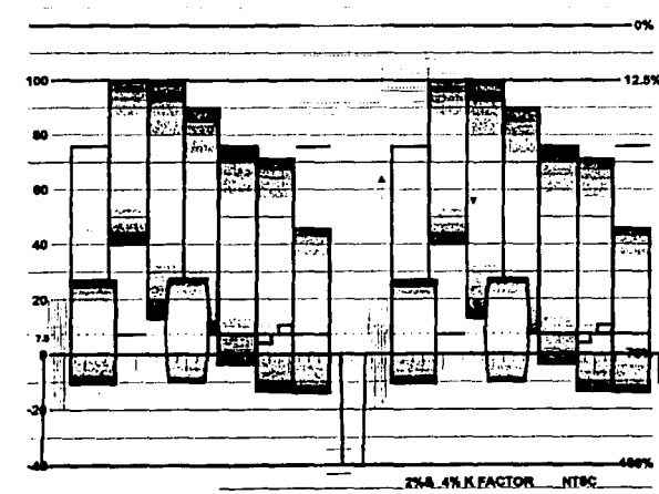
Figura 3.2. Forma de onda desplegando una señal de barras de color.
