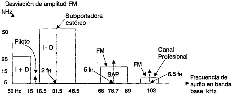
Figura 3.1. Espectro en frecuencia de varias señales multiplexadas a la vez.
