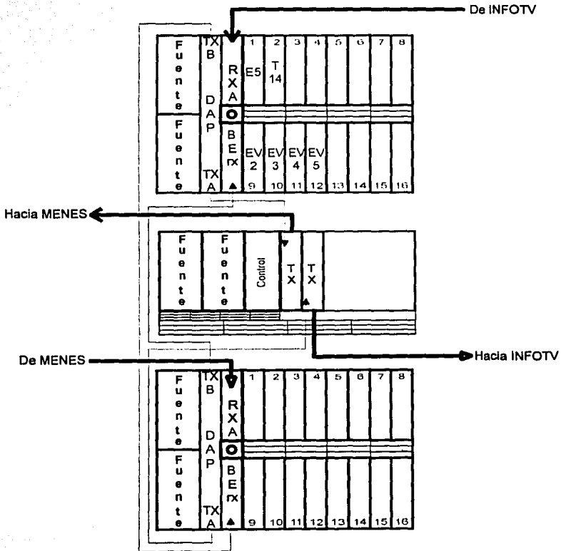
Figura 5.31. Conexiones para el equipo en MENTV-Eventos (anillo 2).
