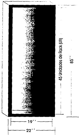
Figura 5.14. Rack para montar equipo.
