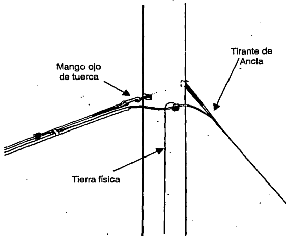
Figura 5.6. Fin de poste con sujeción de tirante de ancla.
