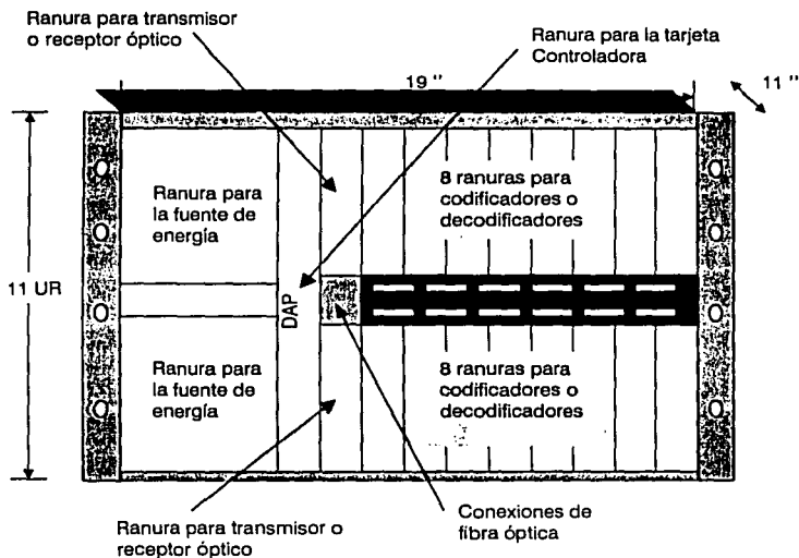
Figura 5.16. Módulos de transmisión y/o recepción.
