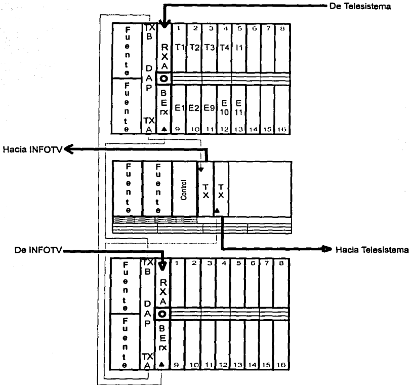
Figura 5.26. Conexiones para el equipo en Estación de Enlaces (anillo 1).
