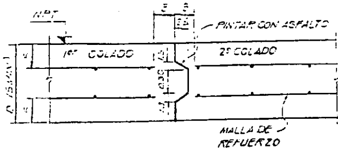
JUNTA DE COLADO LATERAL (A TOPE)
