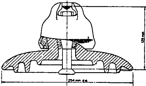
AISLADOR TIPO SUSPENSION
