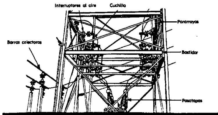
Interruptores al aire, montados sobre el bastidor de una subestación
