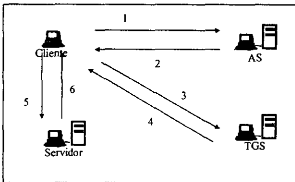
Figura 4.3.1: Proceso de autenticación Kerberos
