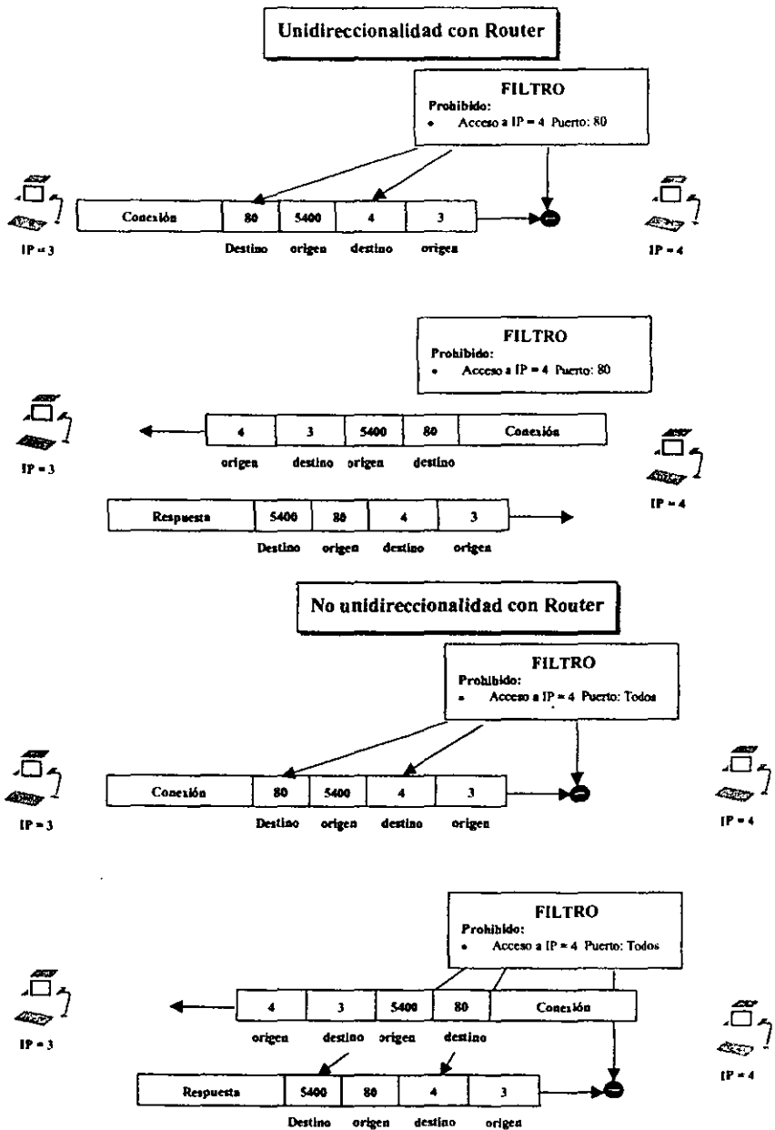
Figura 2.5.2: Direccionalidad con filtros sencillos
