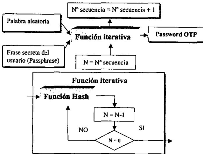
Figura 3.4.1: Algoritmo de una OTP
