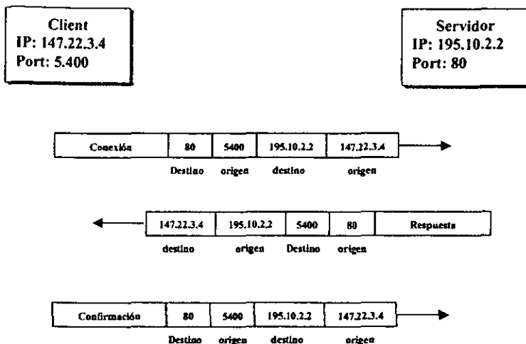
Figura 2.5.1: Apertura de sesión TCP.
