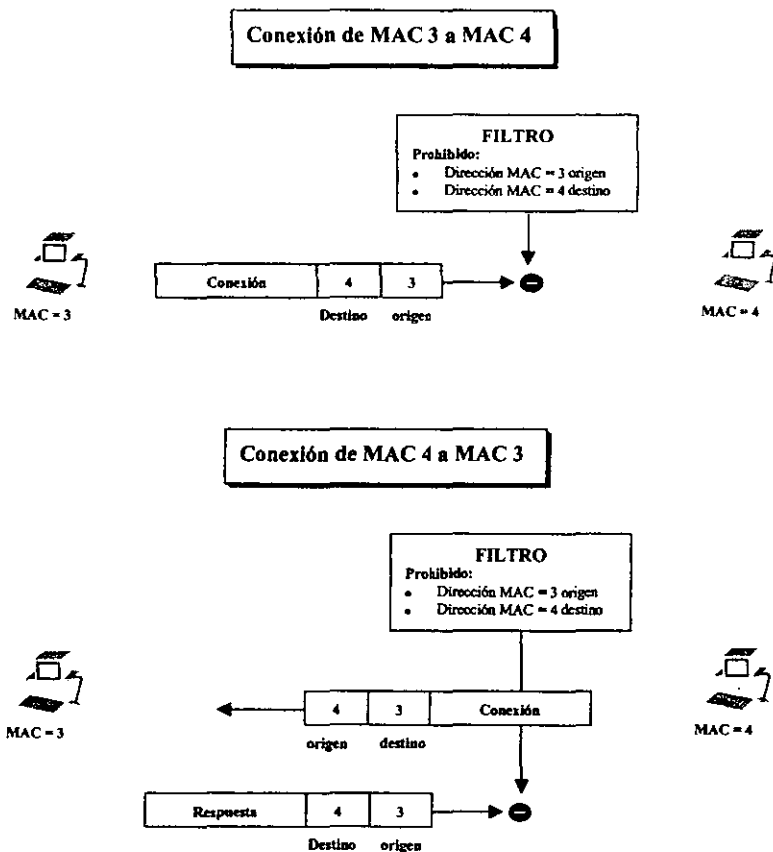
Figura 2.2.1: Bidireccionalidad en filtrado de MAC.
