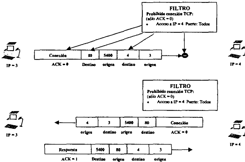
Figura 2.5.3: Direccionalidad con Firewall.
