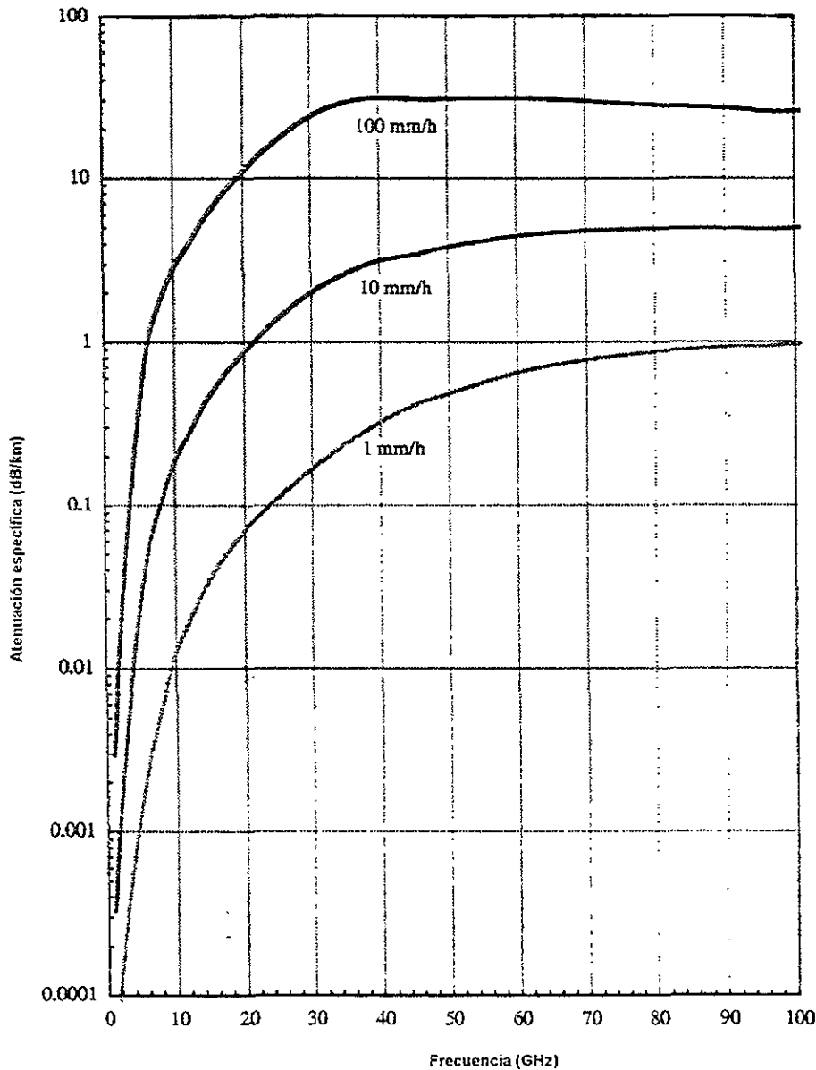
Figura 7. Atenuación específica ocasionada por la lluvia. Los cálculos son para gotas esféricas y una ley de distribución Laws and Parson para el tamaño de las gotas
