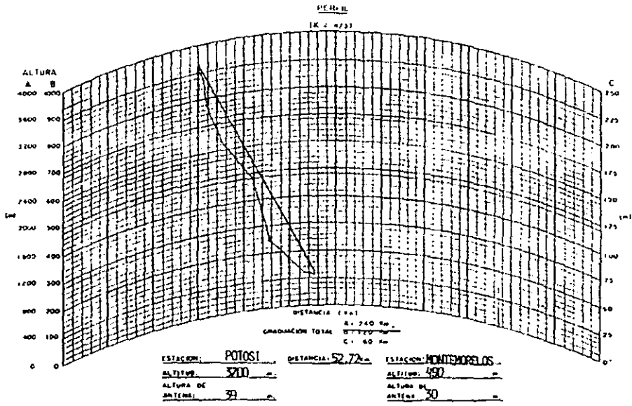
Figura 6.13 Perfil del enlace El Potosí – Montemorelos
