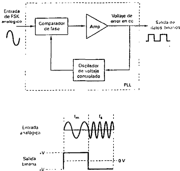
Figura 6.2 Demodulación de FSK-PLL
