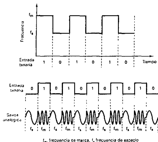
Figura 6.1 Transmisión de FSK binario
