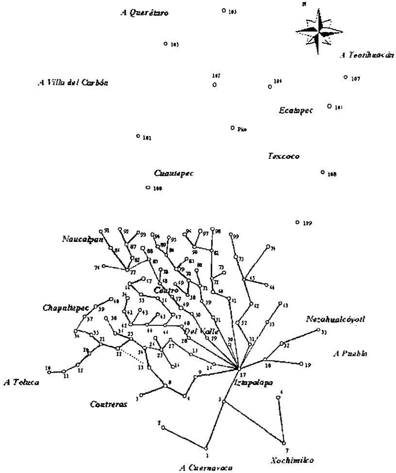
Figura 7.1 Red local actual en el área metropolitana
