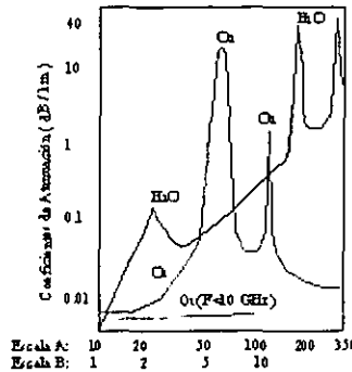
Figura 6.5 Atenuación por gases atmosféricos
