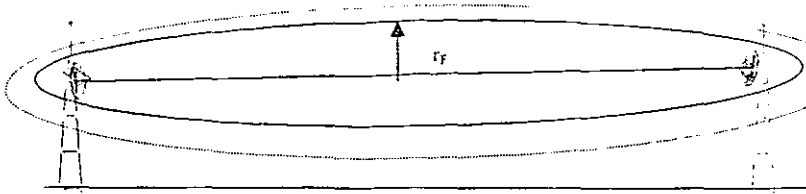
Figura 6.7 Zonas de Fresnel rodeando el haz directo
