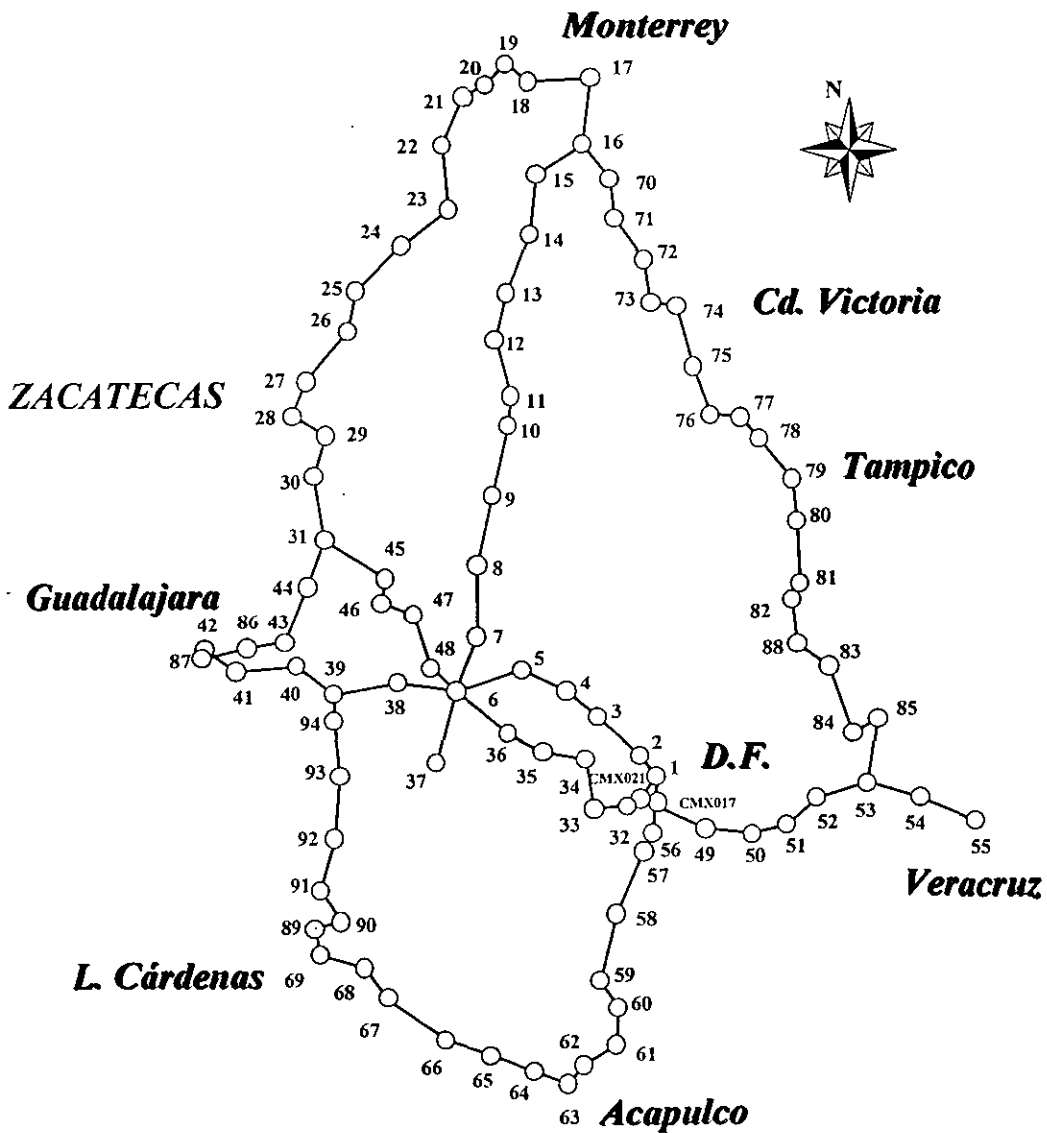
Figura 8.12 Propuesta del back-bone, red a nivel nacional.
