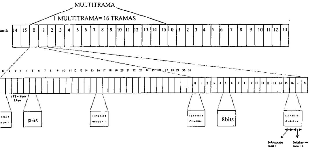
Figura 1-2. Estructura de trama para señal digital de 2 [Mbits]
