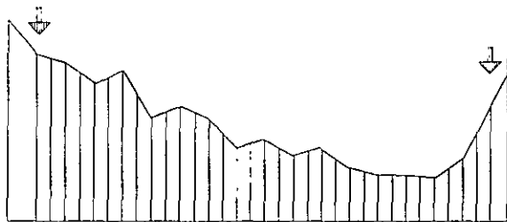
Figura 6.10 Rugosidad del terreno, referida al nivel del mar.
