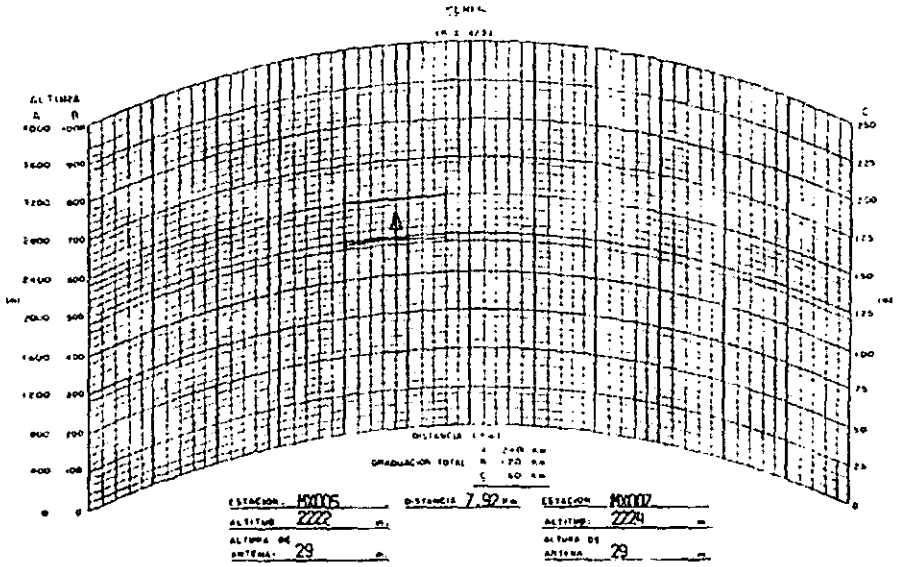
Figura 6.14 Perfil del enlace CMX005-CMX007
