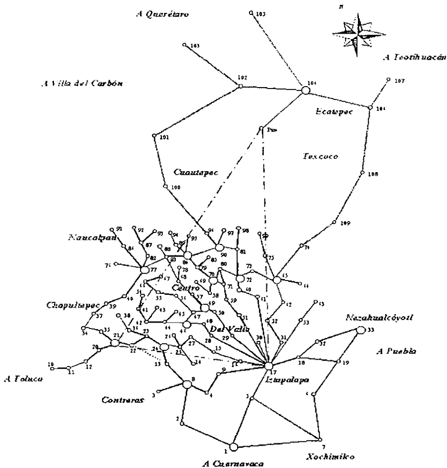
Figura 7.5 Red local optimizada
