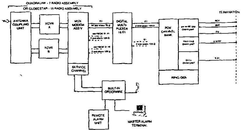
Figura 4.4 Diagrama de bloques y niveles
