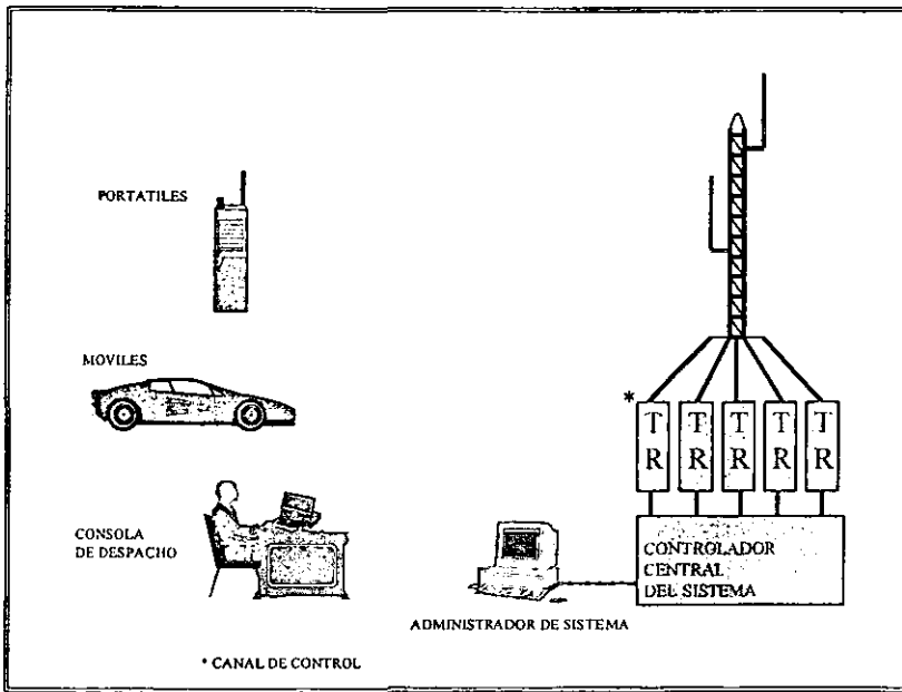
Figura 1.4 Trunking Analógico
