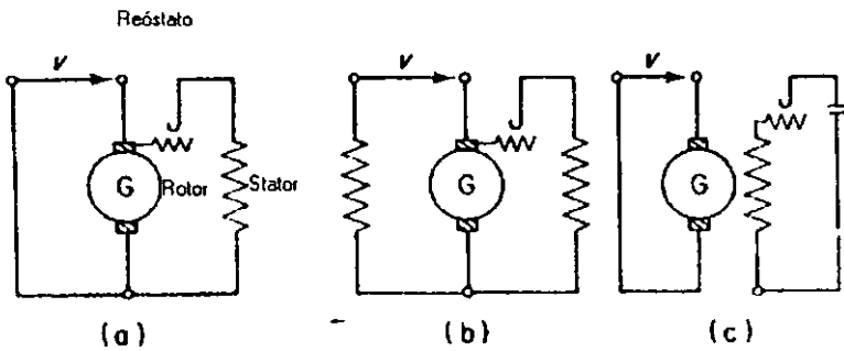
Figura 1.14 Métodos de excitación de generadores CD: (a) excitación cerrada; (b) excitación compuesta; (c) excitación separada.
