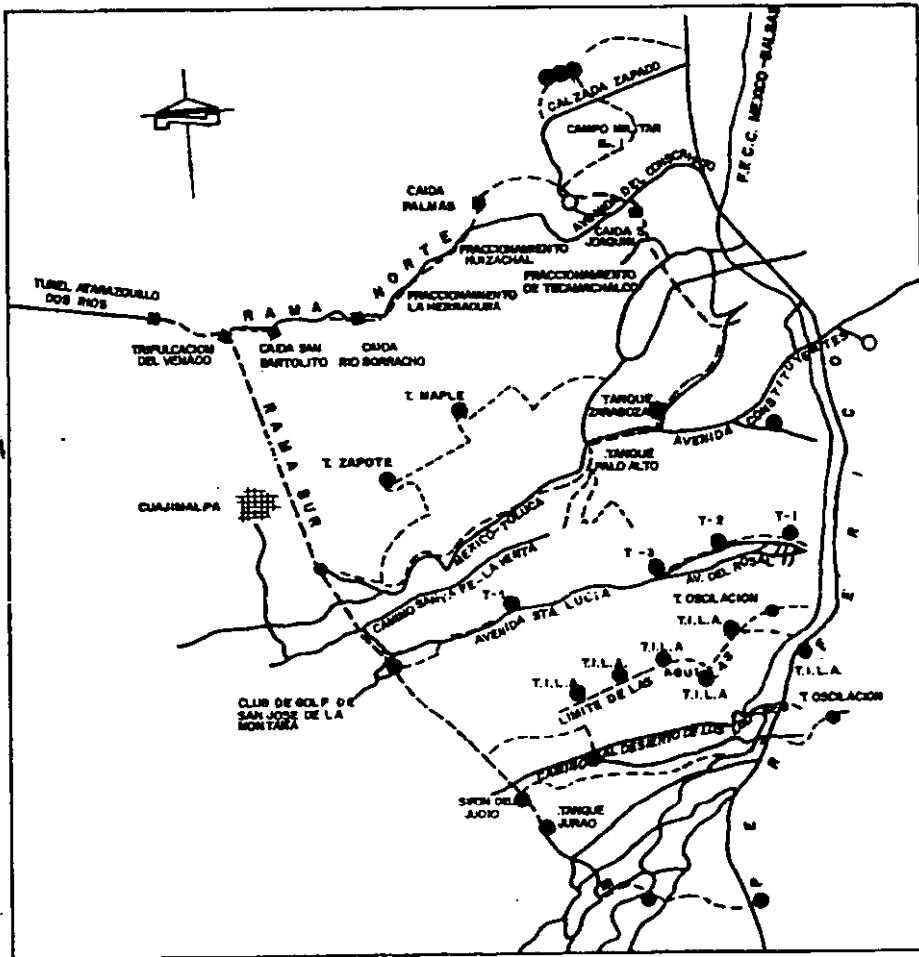
Figura 2.10 Croquis del Sistema Lerma
