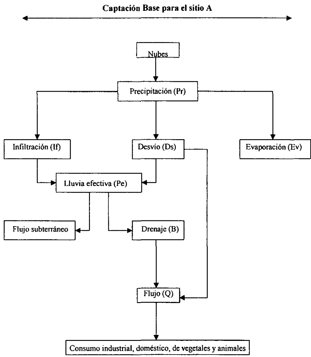
Figura 1.0 Esquema del Ciclo del Agua para una Captación Base
