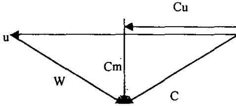
Figura 1.8 Triángulo de velocidades
