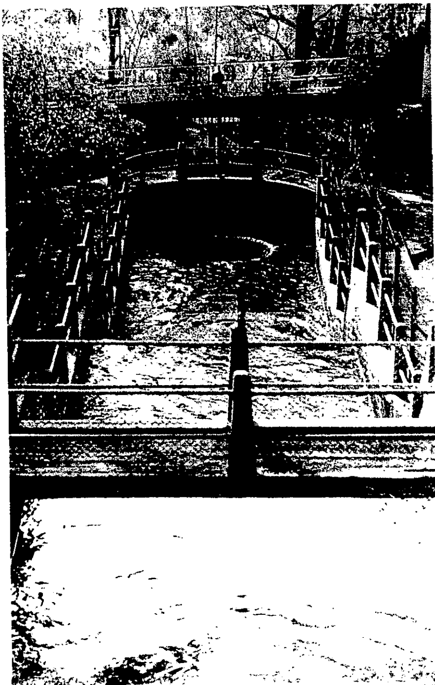
Foto 12. By-pass en forma de vertedores reductores de velocidad. Caída "San Joaquín".
