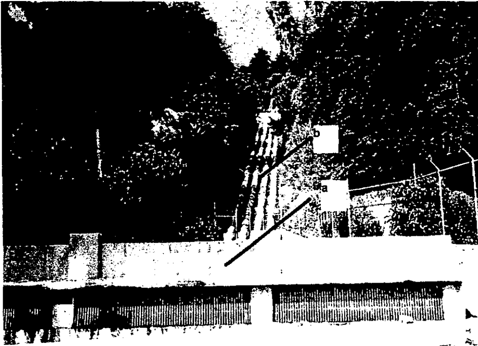
Foto 3 a)Caja rompedora de presión para salvar desnivel y b) by-pass en "San Bartolito".
