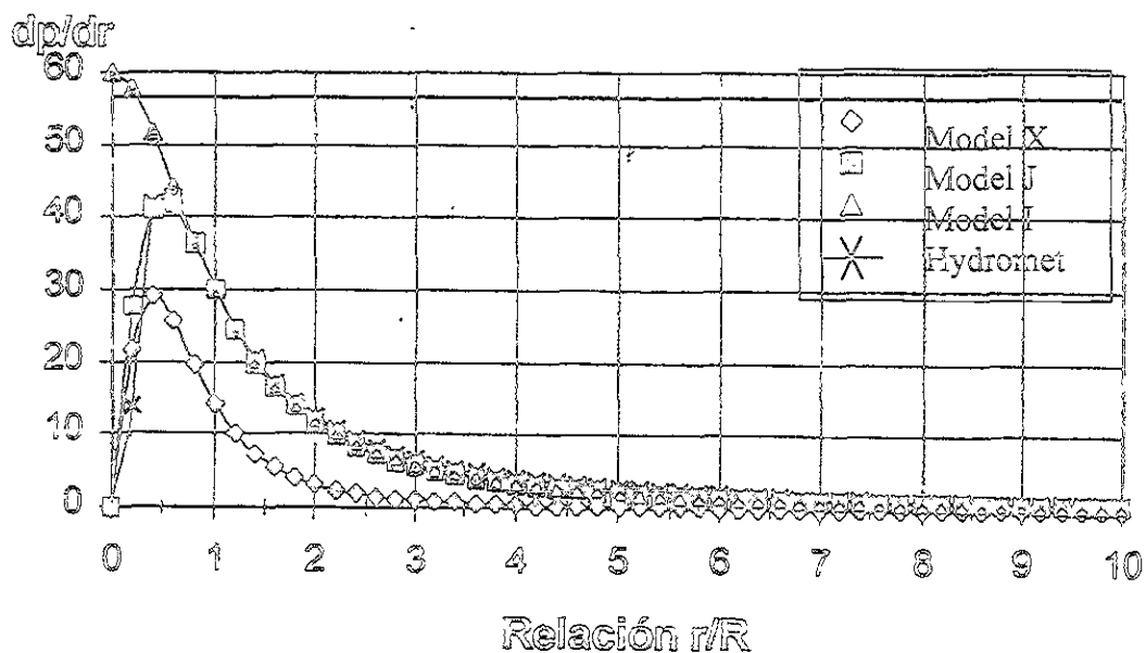
Figura 2.5. Resultados de dp/dr vs. r/R obtenidos para los diferentes modelos considerados, utilizando R = 10 millas náuticas, P_R = 962 mbs y \max(r dp/dr) = 30 mbs
