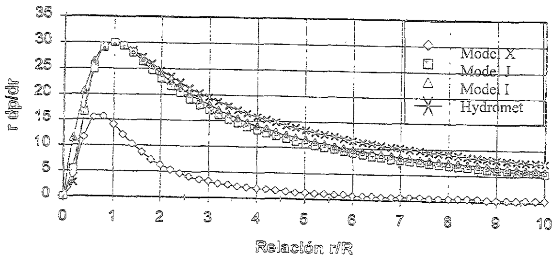
Figura 2.5. Resultados de dp/dr vs. r/R obtenidos para los diferentes modelos considerados, utilizando R = 10 millas náuticas, P_R = 962 mbs y \max(r dp/dr) = 30 mbs
