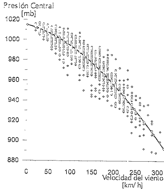
Figura 3.4. Distribución de los datos de presión vs. velocidad de viento, para la vertiente Atlántica, así como el la curva de ajuste propuesta.
