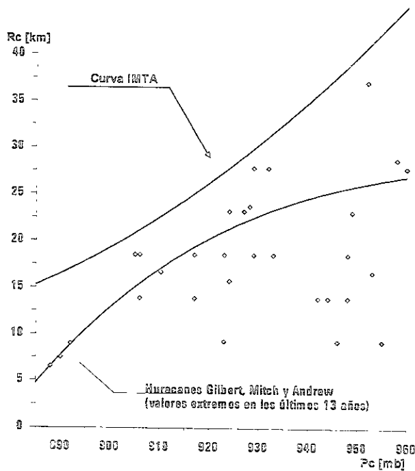
Figura 3.6. Ajuste entre los datos de P_C vs. R_C . Se presentan dos ajustes el propuesto por el IMTA y el de este estudio.
