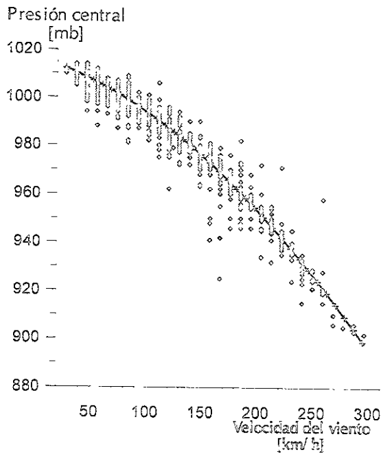
Figura 3.5. Distribución de los datos de presión vs. velocidad de viento, para la vertiente Pacífica, así como el la curva de ajuste propuesta.
