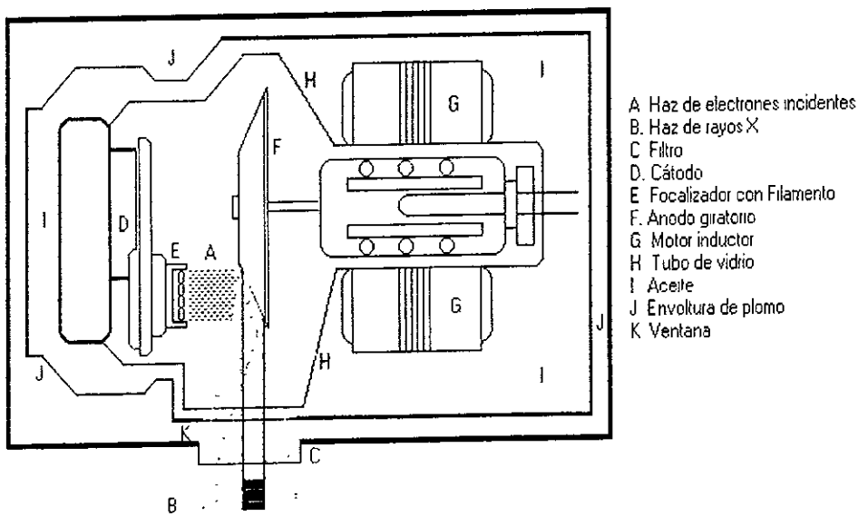
Fig 3 Tubo de rayos X con ánodo giratorio (Modificado de Douglas, 1987)
