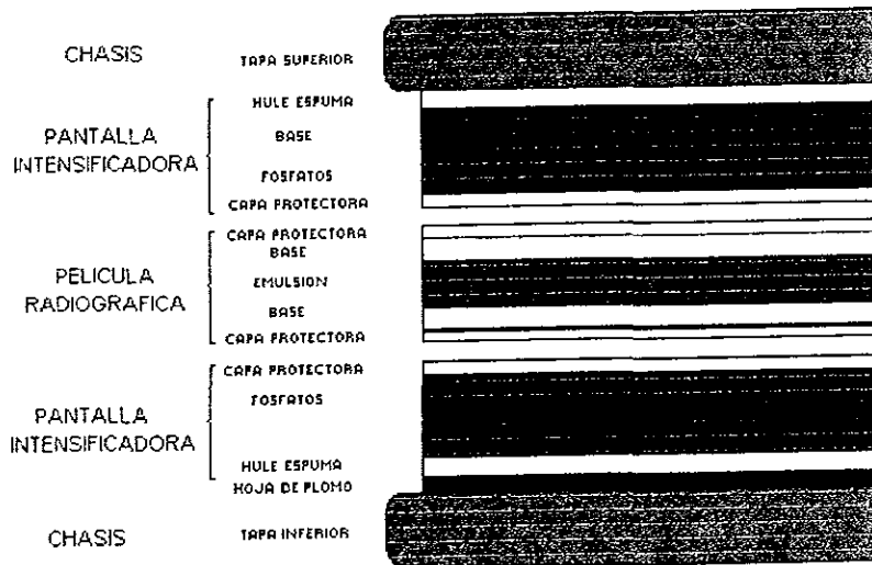
Fig 13. Corte Transversal Chasis, Pantallas Intensificadoras, Película
