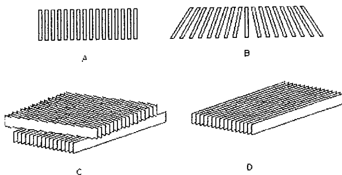
Fig 9. A) Perpendicular (corte transversal), B) Focalizada (corte transversal), C) Cruzada, D) Lineal
