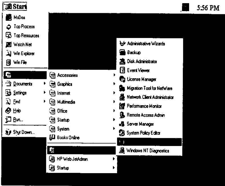
Figura 1.4.2.1 Windows NT
