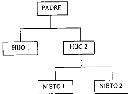
Figura 1.6.1.1. Estructura jerárquica.
