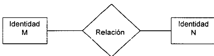
Figura 1.6.3.3. Relaciones.
