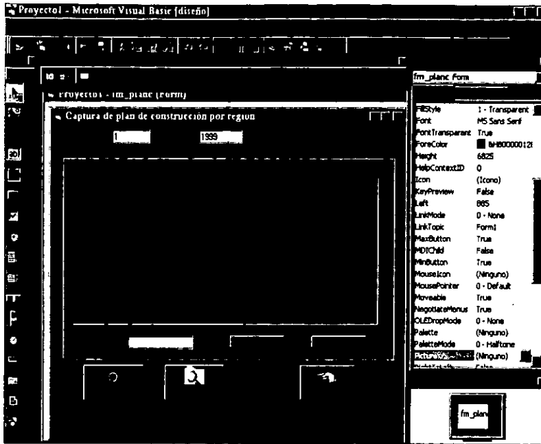
Figura 3.3.9. Control rejilla.
