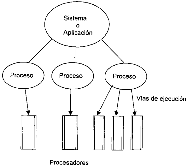
Figura 1.4.2.3. Procesamiento simétrico.
