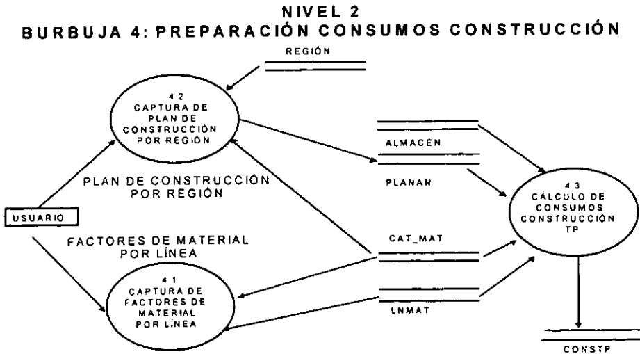
Figura 3.1.2.11. Burbuja 4: Generación de consumos. Nivel 2.
