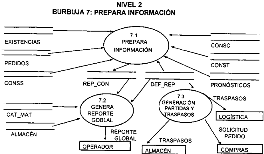
Figura 3.1.2.14. Burbuja 7: Preparación de la información. Nivel 2.
