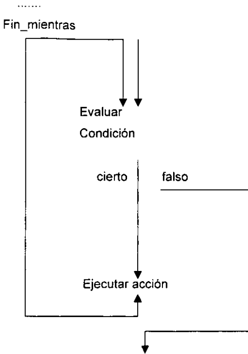
Figura 1.2.5. Estructura mientras.
