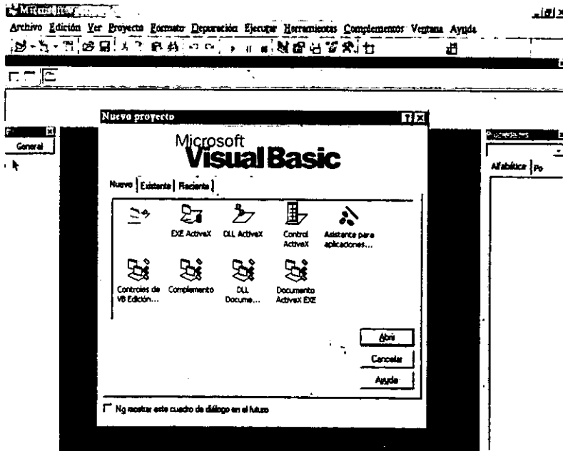
Figura 3.3.1. Nuevo proyecto.
