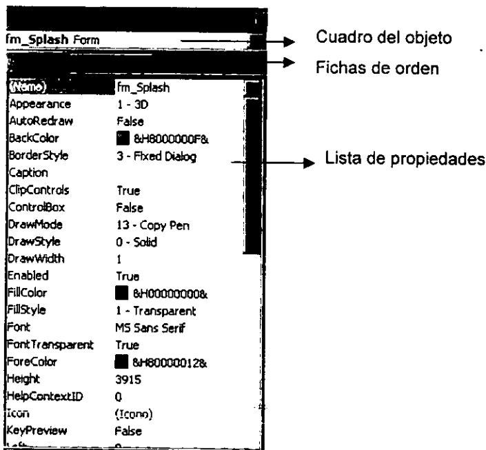
Figura 3.3.4. Ventana Propiedades.
