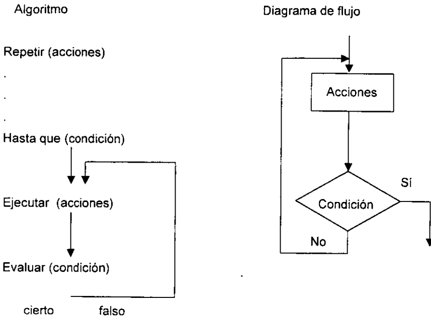
Figura 1.2.6. Estructura DOUNTIL.
