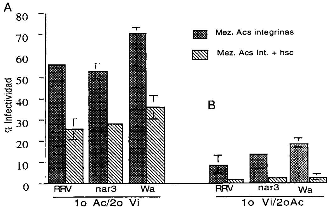
Figura. 5 Acs contra las integrinas \alpha , \beta 2, \beta 3 y la proteína hsc70, bloquean el 99% la infectividad de los rotavirus, cuando se incuban después de unir el virus a la célula. Todo el procedimiento se hizo a 4 °C. La mitad de la placa se incubó primero con rotavirus durante 50 minutos, para permitir que éstos se unieran a la célula, se lavaron y segundo se incubaron con el Ac durante 50 minutos (1o virus/2o Ac). Como control, en la otra mitad de la placa se invirtió el procedimiento (1o Ac/2o virus). Las células se lavaron y se continuó con la infección como se describe en materiales y métodos. Se mezclaron 20 \mu g/ml de Acs policlonales contra la integrinas \alpha , \beta 3 y \beta 2 o a la mezcla de Acs contra las integrinas se añadió 80 \mu g/ml de Acs policlonales contra la proteína hsc70. (A). Primero Ac/Segundo virus (B). Primero virus/Segundo Ac. Las barras representan el error estandar de al menos tres experimentos, realizados por duplicado.
