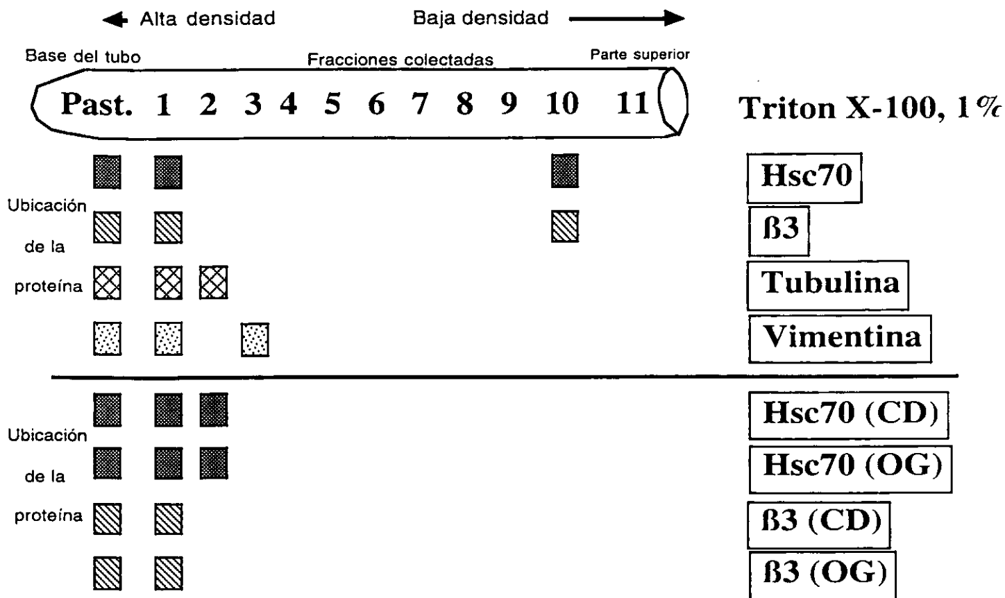
Figura. 10. Las proteínas hsc70 y la integrina \beta 3 se encuentran en los microdominios lipídicos. "rafts" en las células MA104. Las células se lisaron con 1% de Tritón X100 durante 30 minutos y sobre el lisado, en 40% de sacarosa, se hizo un gradiente lineal de sacarosa (5% - 30%) sin tritón X100. El gradiente fue centrifugado durante 15 - 22 hr a 200.000 x g en un rotor SW41. Las fracciones se recolectaron desde la parte inferior del tubo hasta la superior por aspiración (fracciones 1 al 11). Cada fracción se precipitó con 5 volúmenes de acetona y las fracciones se analizaron por Western blot utilizando Acs específicos. Como control, se hizo el mismo procedimiento a células previamente tratadas con ciclodextrina (CD), para retirar el colesterol de la membrana citoplasmática o a células lisadas con el detergente octil glucósido (OG) al 0.8%, en lugar del 1% de Tritón X100, para solubilizar los microdominios lipídicos. Los cuadros rellenos indican la presencia de la correspondiente proteína en cada fracción.
