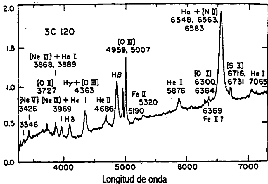
Figura 3: Espectro del núcleo de 3C120 (Tomado de Phillips & Osterbrock, 1975)
