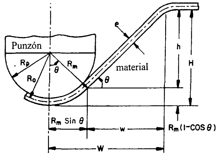
Figura 2.9. Análisis de la deformación, por el método de la membrana.
