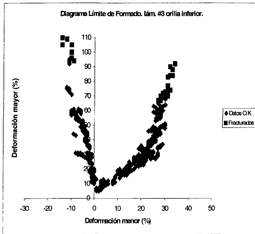
Figura 4.5. Diagrama límite de formado, lámina #3 para costado vehículo largo. Probetas de orilla inferior del rollo.
