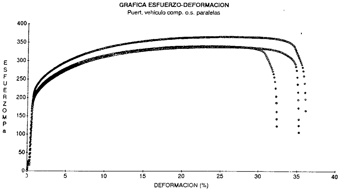
Figura 1.5. Gráfica esfuerzo-deformación, lámina puerta vehículo compacto, esquina superior, a 0° con respecto al eje de laminación.
