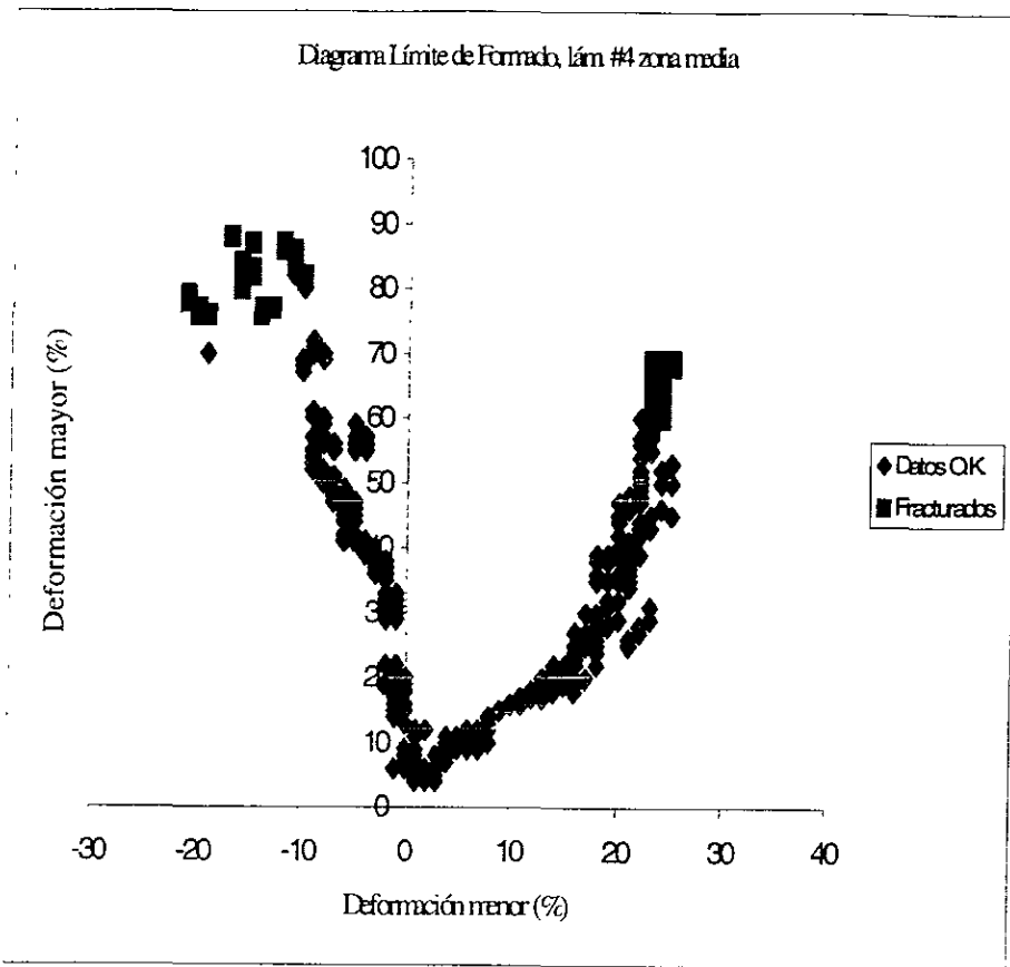
Figura 4.7. Diagrama límite de formado, lámina #4 para partes interiores. Probetas de zona media de rollo.
