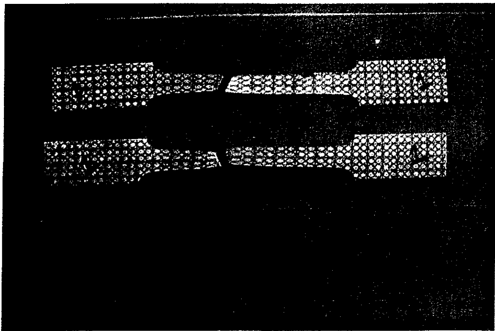
Figura 3.5. Probetas de tracción después del ensayo.
