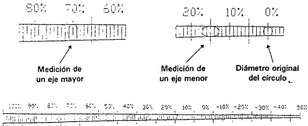
Figura 2.2. Regla flexible para medir el porcentaje de deformación.
