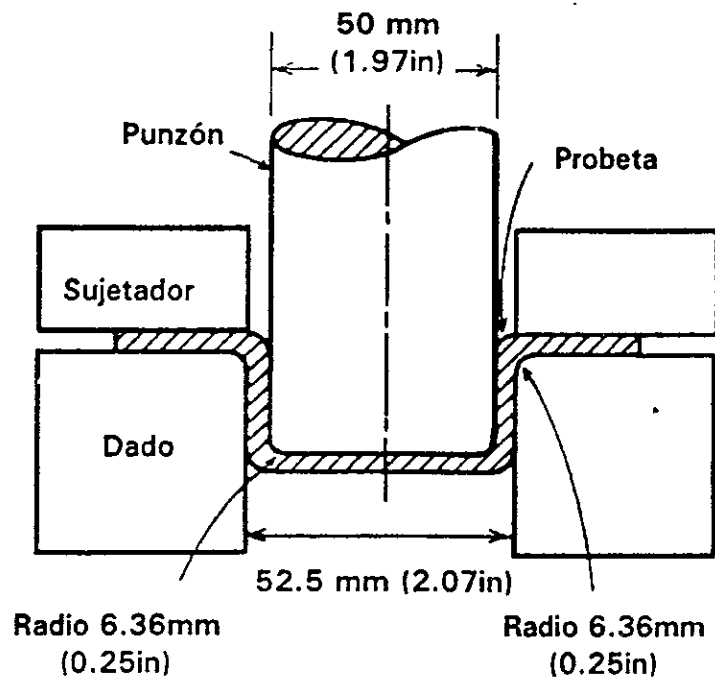
Figura 1.6. Herramental para ensayo Swift.
