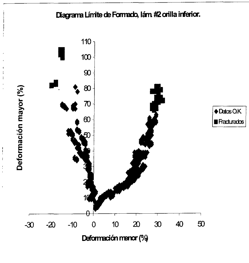
Figura 3.7. Diagrama límite de formado, lámina #2 para puertas vehículo compacto. Probetas de orilla inferior del rollo.
