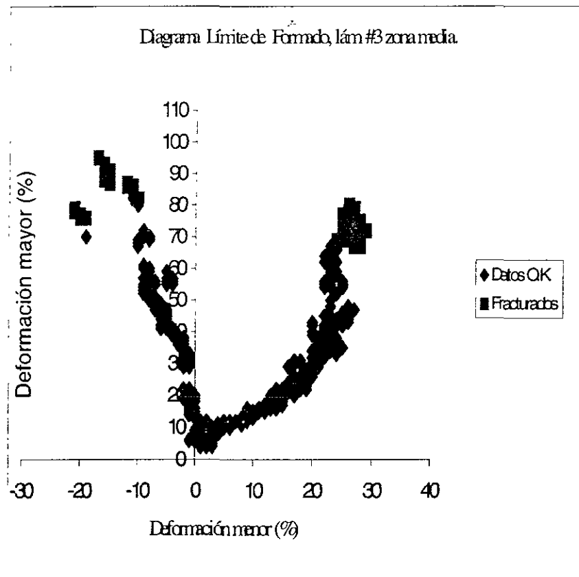
Figura 4.6. Diagrama límite de formado, lámina #3 para costado vehículo largo. Probetas zona media del rollo.
