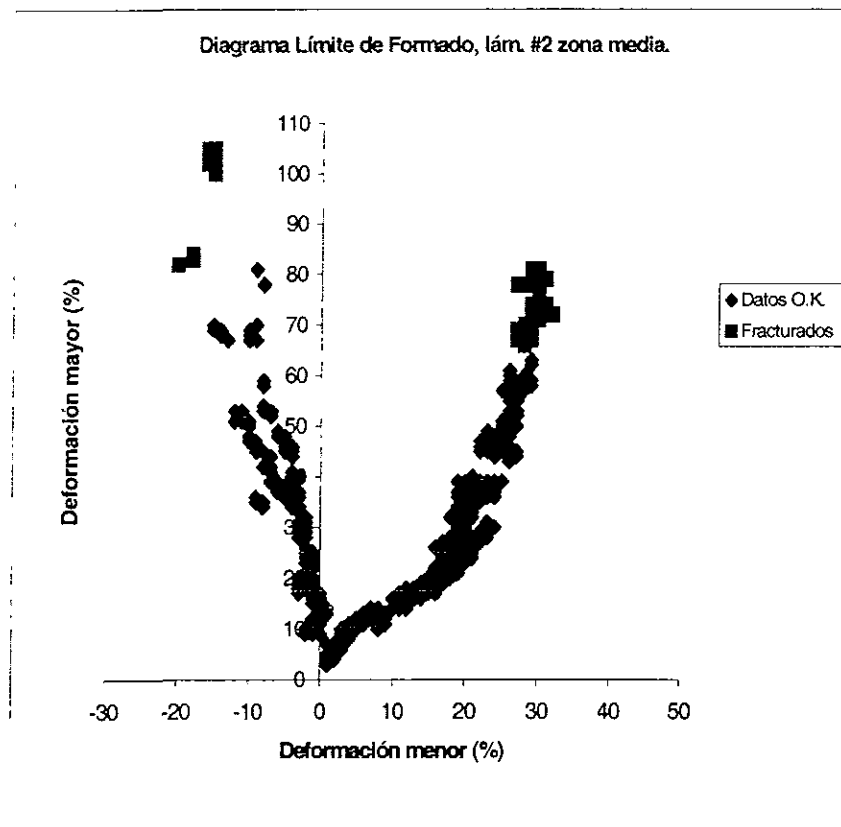
Figura 4.4. Diagrama límite de formado, lámina #2 para puertas vehículo compacto. Probetas de zona media del rollo.
