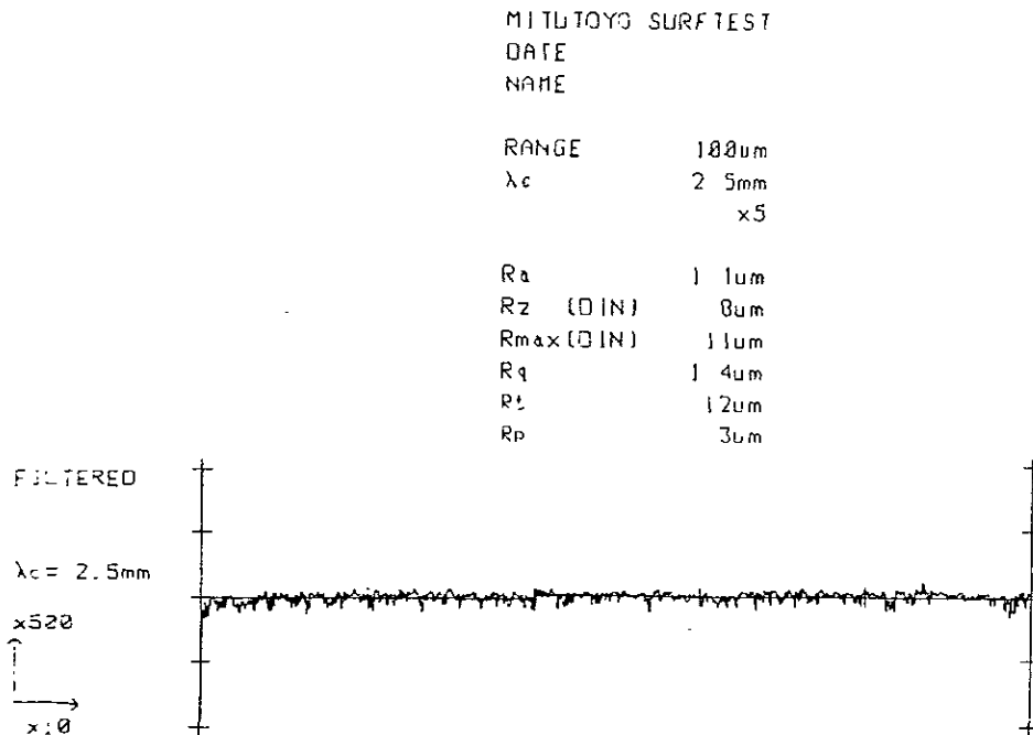
Figura 3.2. Gráfica de perfil de rugosidad, lámina #3 para costado vehículo largo.
