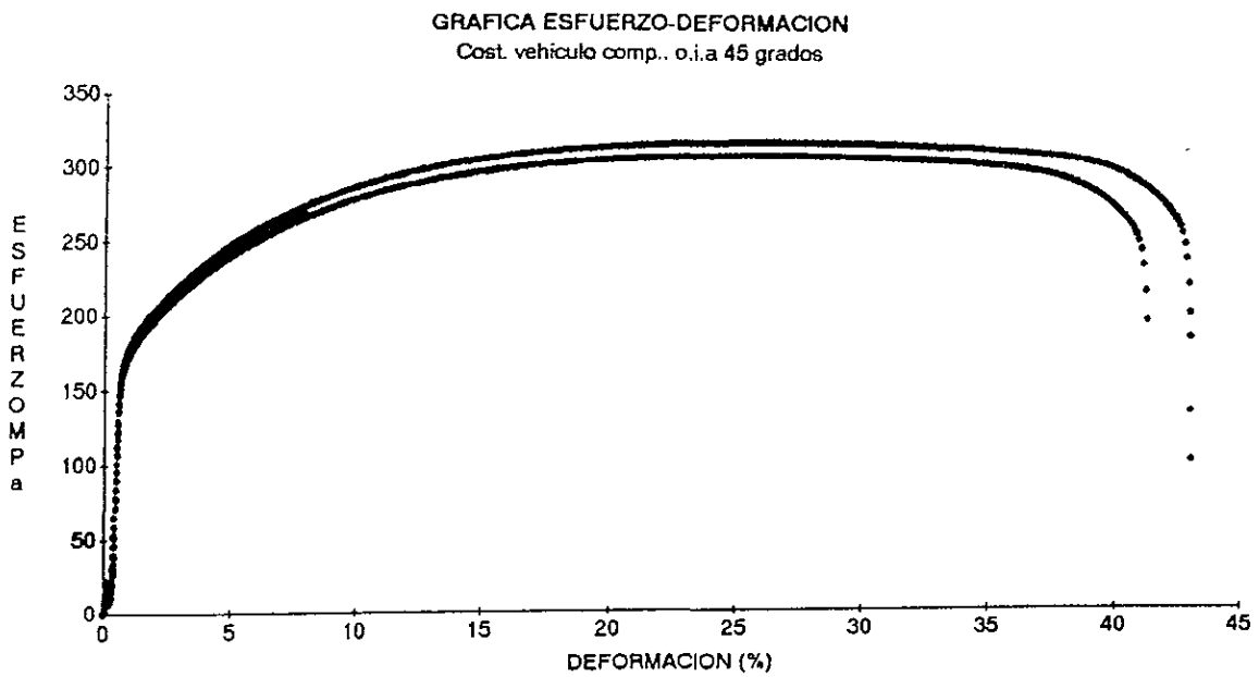
Figura 3.4. Gráfica esfuerzo-deformación, lámina #3 para costado vehículo compacto, esquina inferior, a 45° con respecto al eje de laminación.
