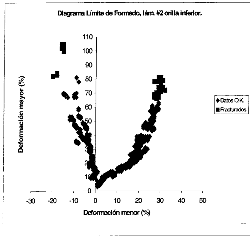
Figura 4.3. Diagrama límite de formado, lámina #2 para puertas vehículo compacto. Probetas de orilla inferior del rollo.
