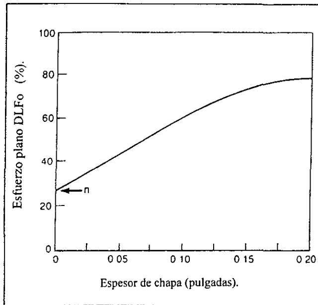
Figura 2.6. Efecto del espesor de material en el DLFo.
