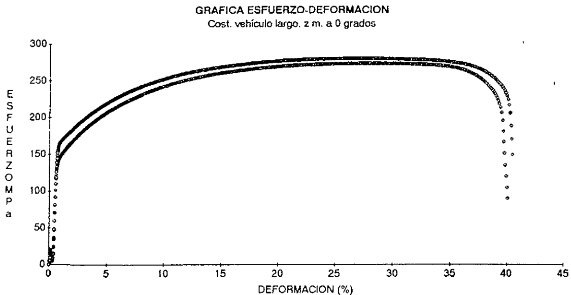
Figura 1.1. Gráfica esfuerzo-deformación, lámina para costado vehículo largo, zona media, a 0° con respecto al eje de laminación.
