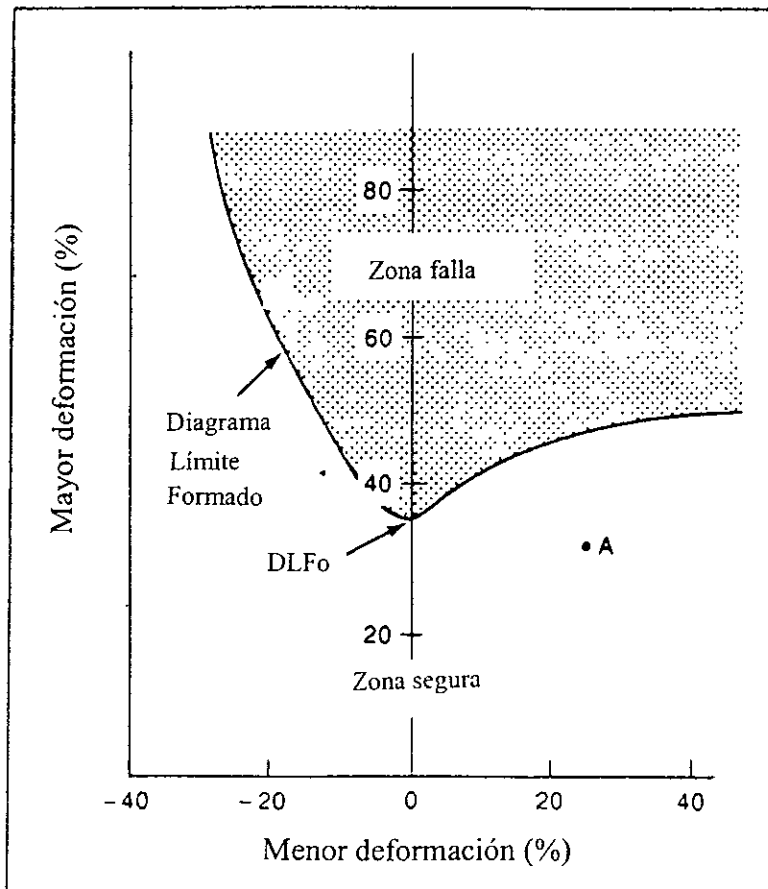
Figura 2.5. Representación de coordenada de deformación plana DLFo.
