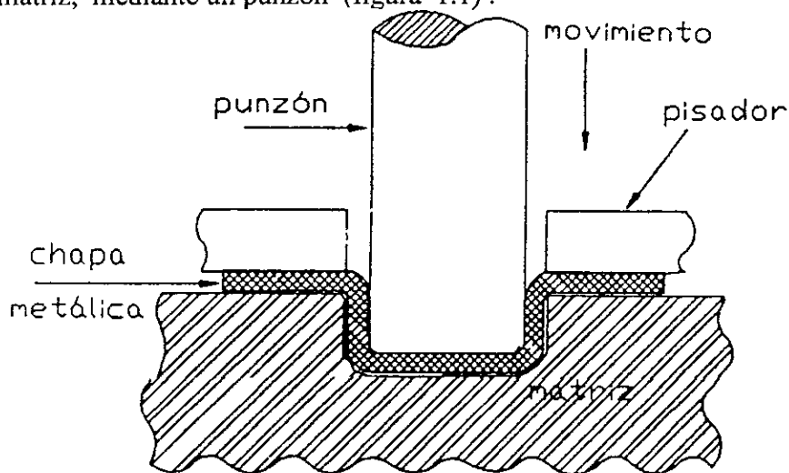
Figura 1.1. Operación de embutido. [Referencia. autor]
