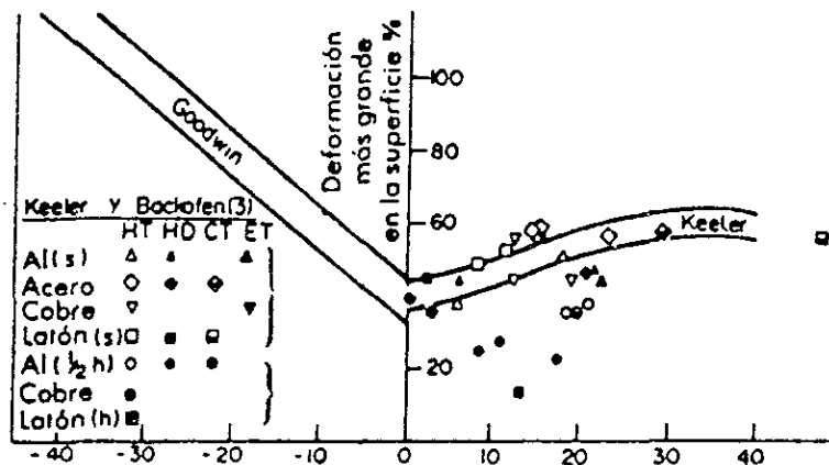
Figura 2.3. Diagrama límite de formado típico.
