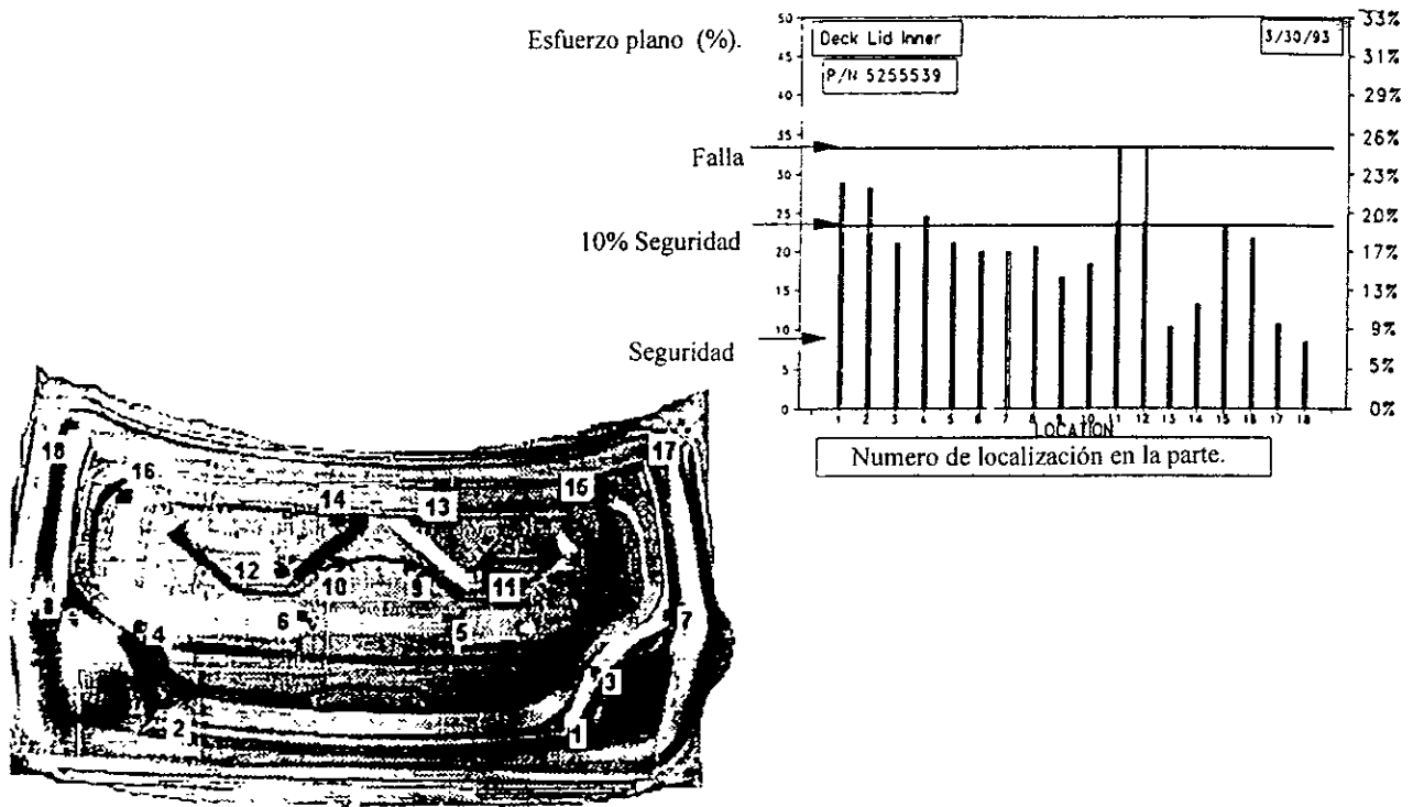
Figura 2.7. Gráfica de análisis de espesores, en las absisas con números se identifican los puntos estudiados, de la parte, y en las ordenadas las líneas de esfuerzo y relación de espesor, que limitan las zonas de seguridad y falla. [Referencia. autor]
