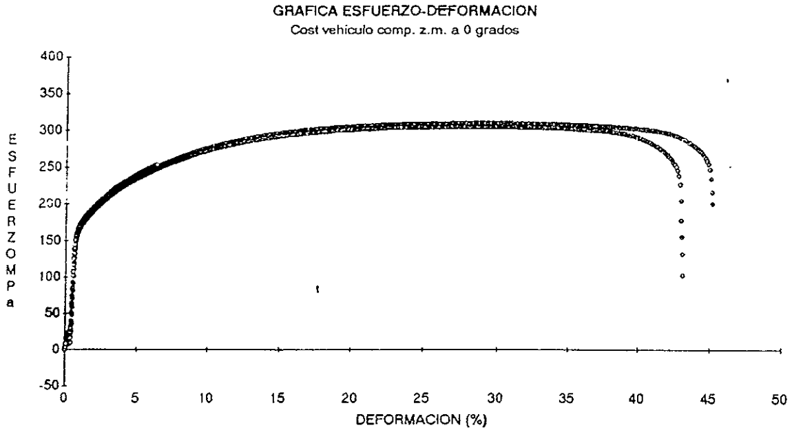
Figura 1.4. Gráfica esfuerzo-deformación, lámina para costado vehículo compacto zona media, a 0° con respecto al eje de laminación
