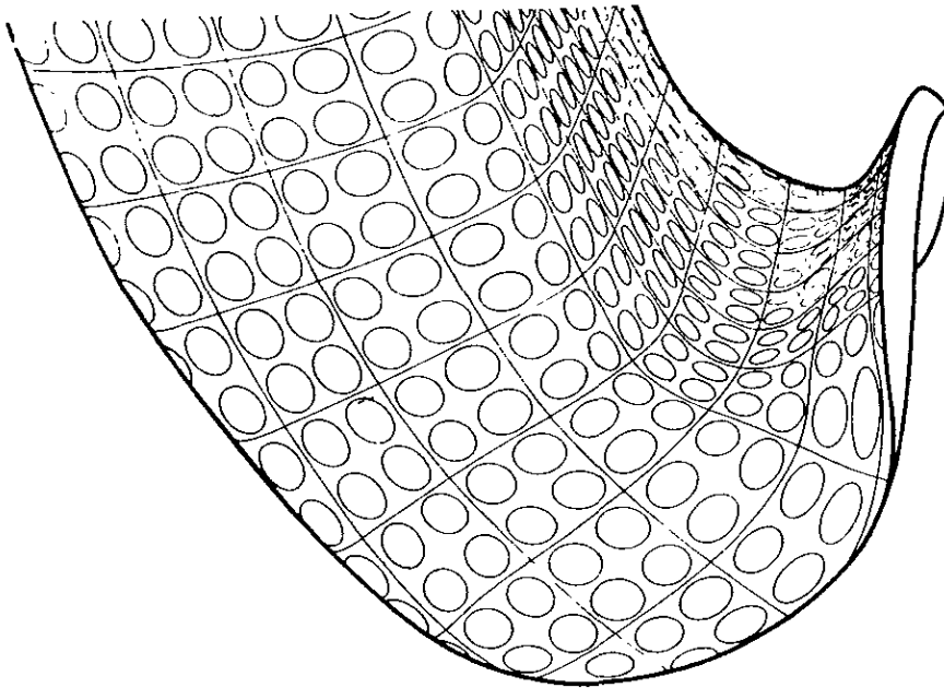
Figura 2.1. Ejemplo de malla circular sobre un parachoques, mostrando la deformación de la malla de círculos.
