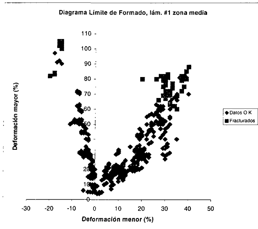
Figura 4.2. Diagrama límite de formado, lámina #1 para costado vehículo compacto. Probetas de zona media del rollo.
