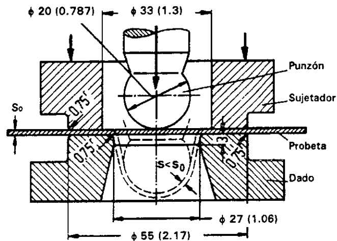
Figura 1.5. Herramental para ensayo Olsen (Erichsen). [Referencia. 14].
