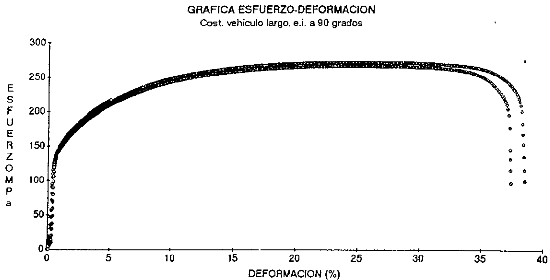
Figura 1.2. Gráfica esfuerzo-deformación, lámina para costado vehículo largo, esquina inferior, a 90° con respecto al eje de laminación.
