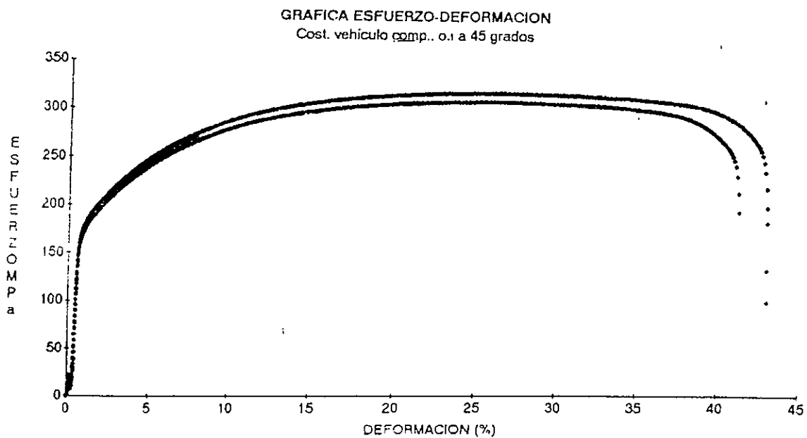
Figura 1.3. Gráfica esfuerzo-deformación, lámina para costado vehículo compacto, esquina inferior, a 45° con respecto al eje de laminación.
