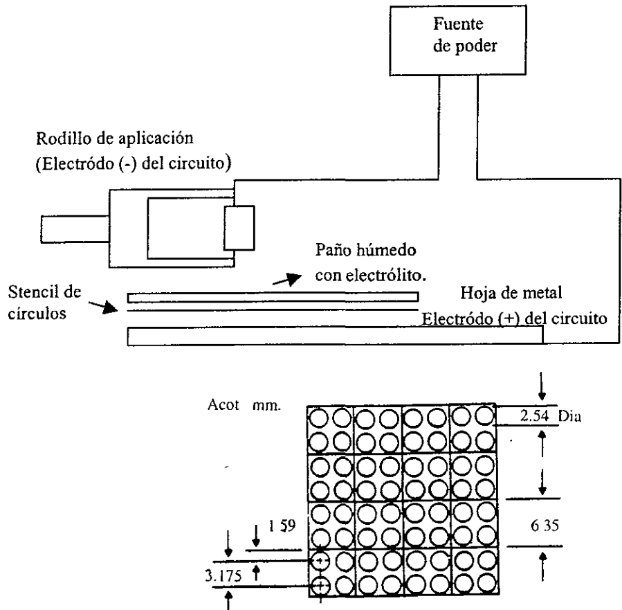
Figura 3.3. Diagrama del equipo para grabar la malla de círculos.
