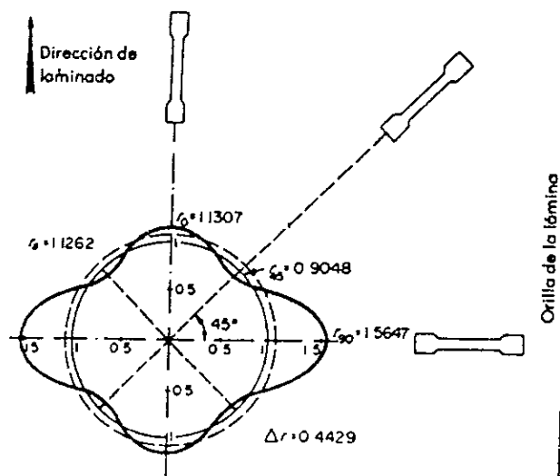
Figura 1.4. Variación típica del índice de anisotropía planar “r”. [Referencia: 13 ].
