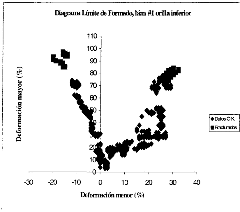
Figura 4.1. Diagrama límite de formado, lámina #1 para costado vehículo compacto. Probetas de orilla inferior de rollo.
