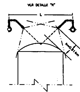
DETALLE "L" LOCALIZACION DE BOQUILLAS EN RECIPIENTES VERTICALES
