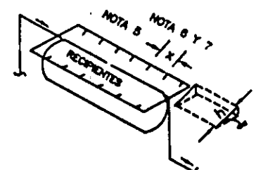
DETALLE "B" ARREGLO GENERAL LOCALIZACION DE BOQUILLAS EN RECIPIENTES HORIZONTALES
