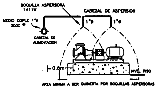
DETALLE "H" ARREGLO DE BOQUILLAS ASPERSORAS PARA PROTEGER BOMBAS
