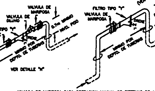
VALVULA DE MARIPOSA PARA OPERACION MANUAL DE SISTEMAS DE ASPIRACION
