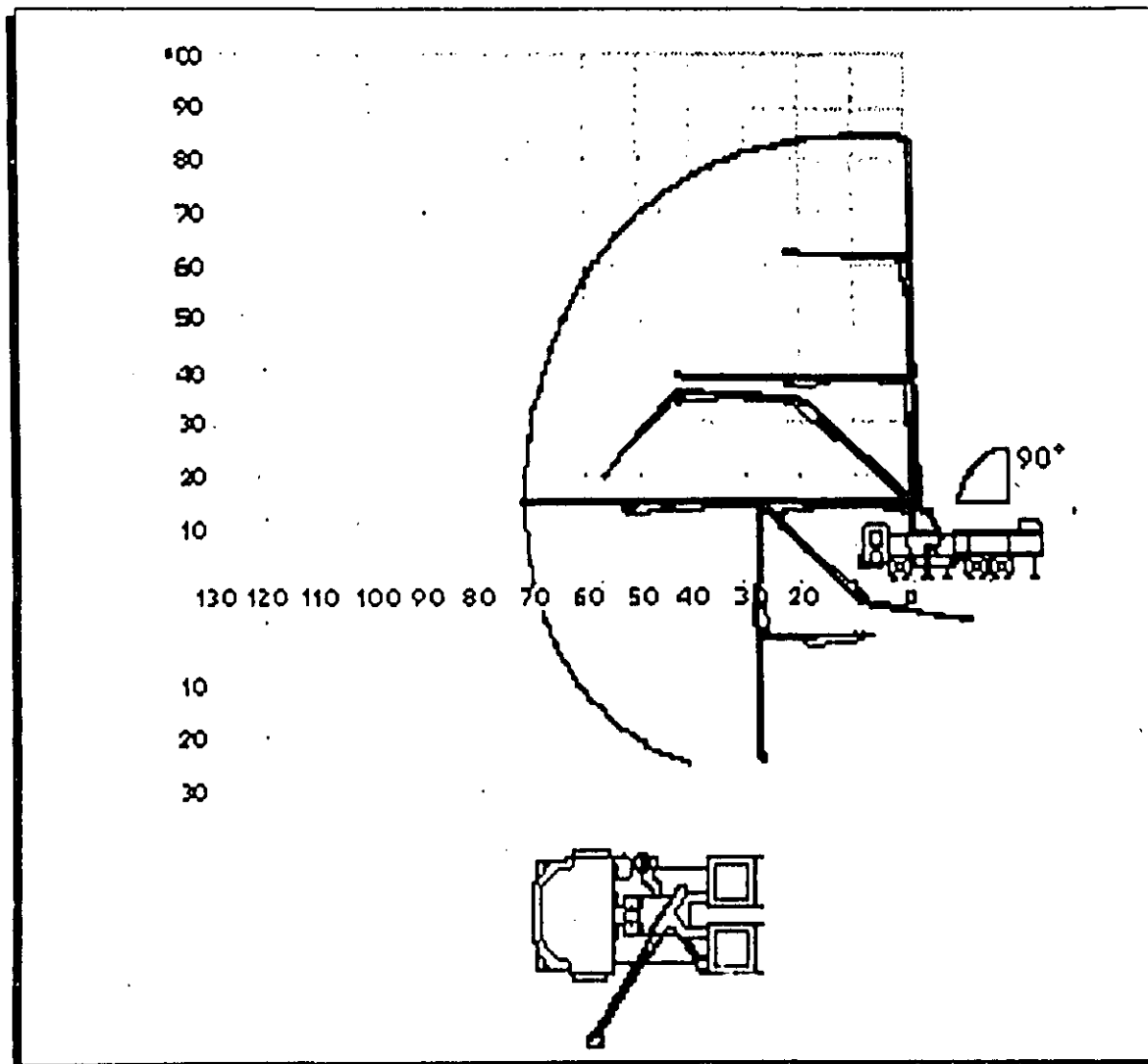
Figura 4.7 : Esquema para vehículos contra incendio, acoplados con pluma de tres brazos, para suministrar agua y/o espuma a gastos altos (2000 a 4000 gpm).
