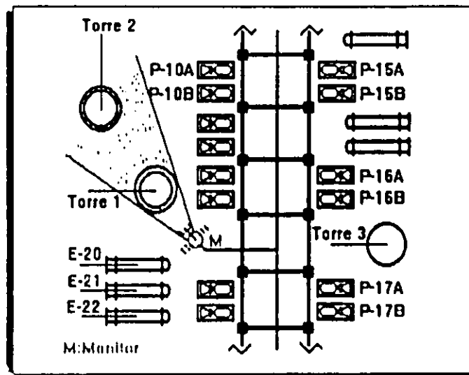
Figura 5.7 : Efecto de apantallamiento de la torre 1 sobre la torre 2, el monitor (M) no puede cubrir el área inmediata trasera a la torre 1, por lo tanto, la torre 2 puede quedar desprotegida.
