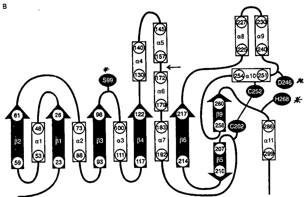
Figura 10. Representación esquemática de la estructura de la lipasa de P. glumae determinada por cristalografía de rayos X (a), y en el caso de la lipasa de Acinetobacter calcoaceticus deducida a partir de la anterior (b). Las flechas representan las hojas \beta y las barras las hélices \alpha ; los residuos de la triada catalítica están indicados con *. En ambos casos la hélice 5 corresponde a la tapa que cubre al sitio activo [152, 179].
