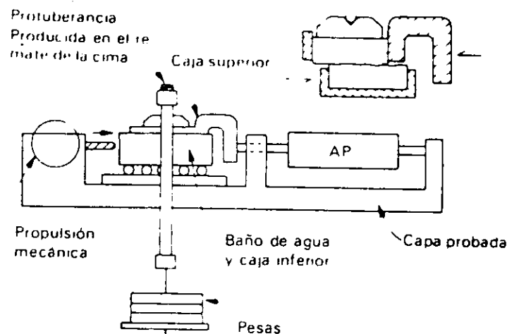
Fig. II.5 Elementos de una caja de esfuerzo cortante directo.
