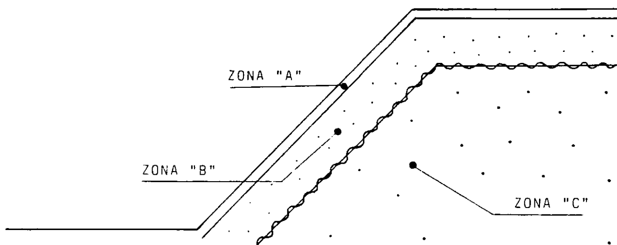
Fig. A.1 Ubicación de las zonas del talud.
