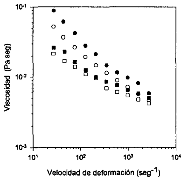
Figura 11. Reograma del caldo de cultivo de células de B. vulgaris crecidas en un fermentador agitado a 400 rpm (■, □) y a 700 rpm (●, ○). Reograma del caldo completo (■, ●) y del medio filtrado (□, ○).
