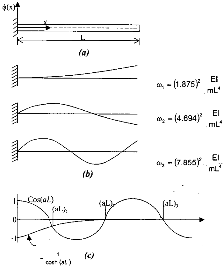
FIGURA III.1.1.2 Análisis de Vibración de una Viga en Cantiliver. a) Propiedades de una viga en cantiliver. b) Primeros tres modos de vibración. c) Términos de la ecuación de frecuencia.
