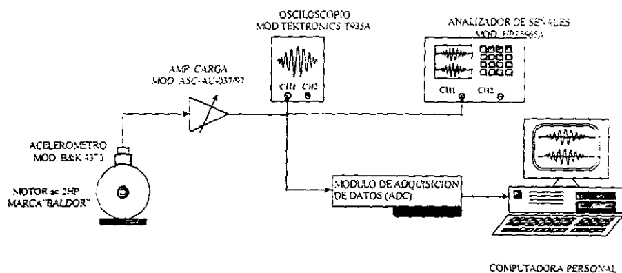
Figura 7.10.- Diagrama de conexión de la instrumentación utilizada para la prueba de campo.
