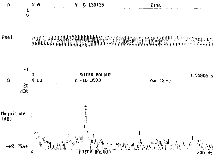
Figura 7.11.- Espectros en el tiempo y frecuencia del motor BALDOR tomado con el Analizador HP 35666A trabajando en condiciones normales de operación
