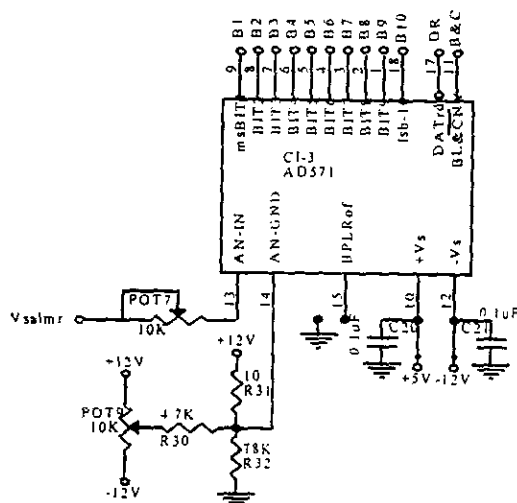
Figura 6.13.- Configuración del AD571.
