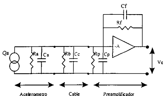
Figura 4.1.- Circuito equivalente del amplificador de carga conectado a un acelerómetro y cable.
