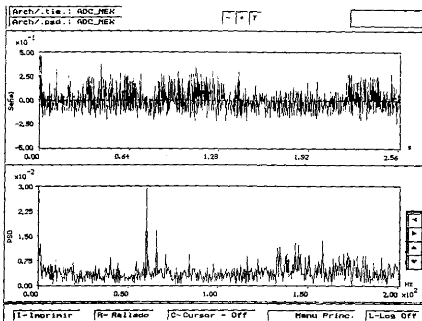
Figura 7.12.- Espectros en el tiempo y frecuencia del motor BALDOR tomado con el sistema de monitoreo trabajando en condiciones normales de operación.
