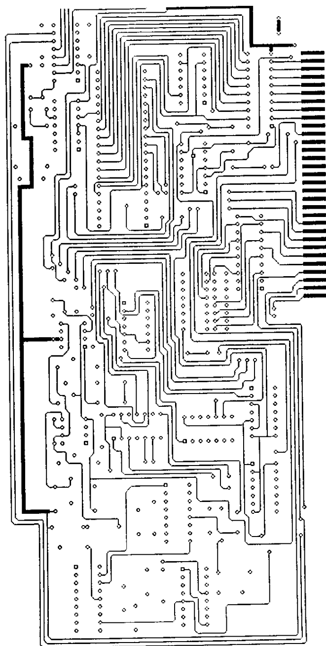
DIAGRAMA PCB DE LA TARJETA DE ADQUISICIÓN (LADO DE COMPONENTES)
