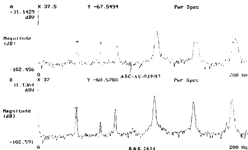
Figura 8.4.- Espectro en frecuencia de los amplificadores ASC-AU-039/97 y B&K 2634 con frecuencia de rotación del motor a 35 Hz.
