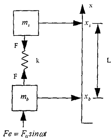
Figura 3.1.- Modelo simplificado de un acelerómetro.
