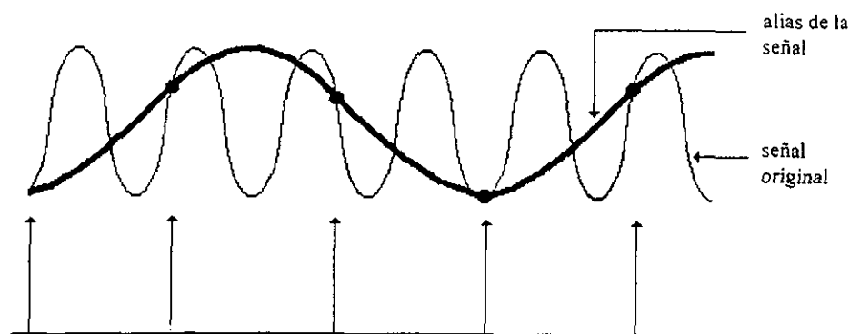
Figura 5.10.- Muestreo de una señal con f_s < 2f_c .
