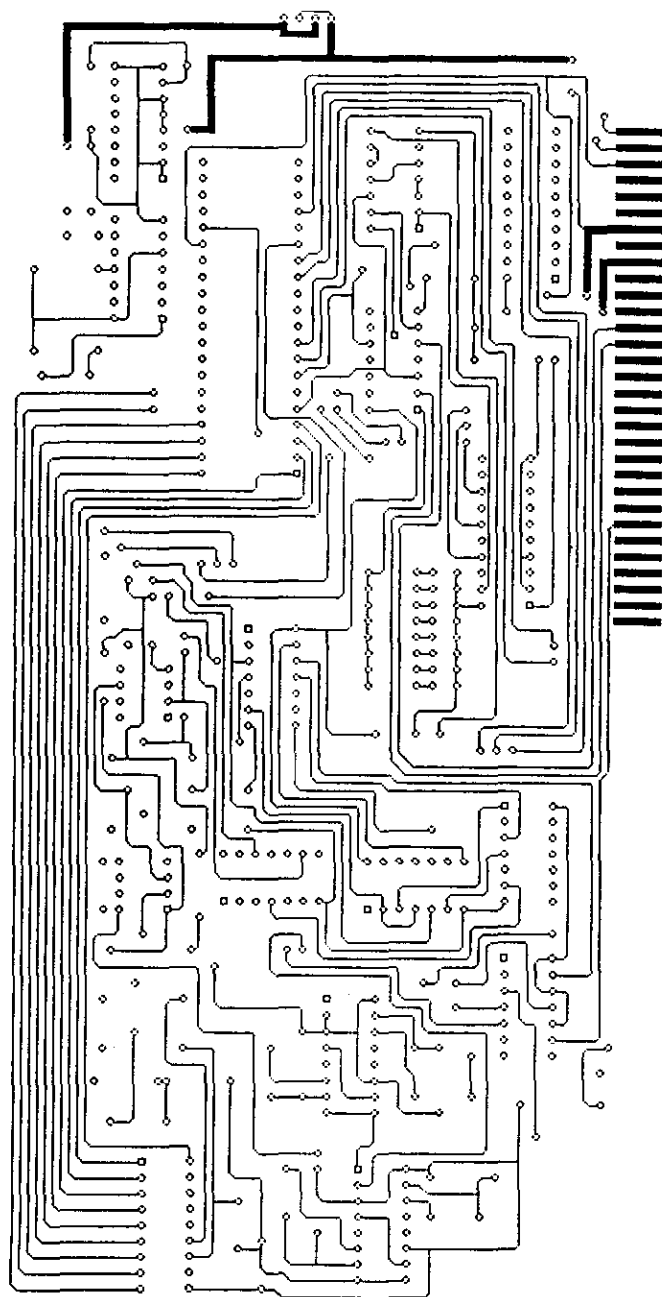
DIAGRAMA PCB DE LA TARJETA DE ADQUISICIÓN (LADO DE SOLDADURA)
