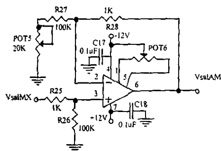
Figura 6.5.- Amplificador de ganancia unitaria.
