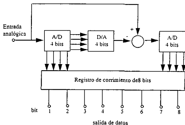
Figura 5.16.- Convertidor A/D del tipo paralelo de 8 bits
