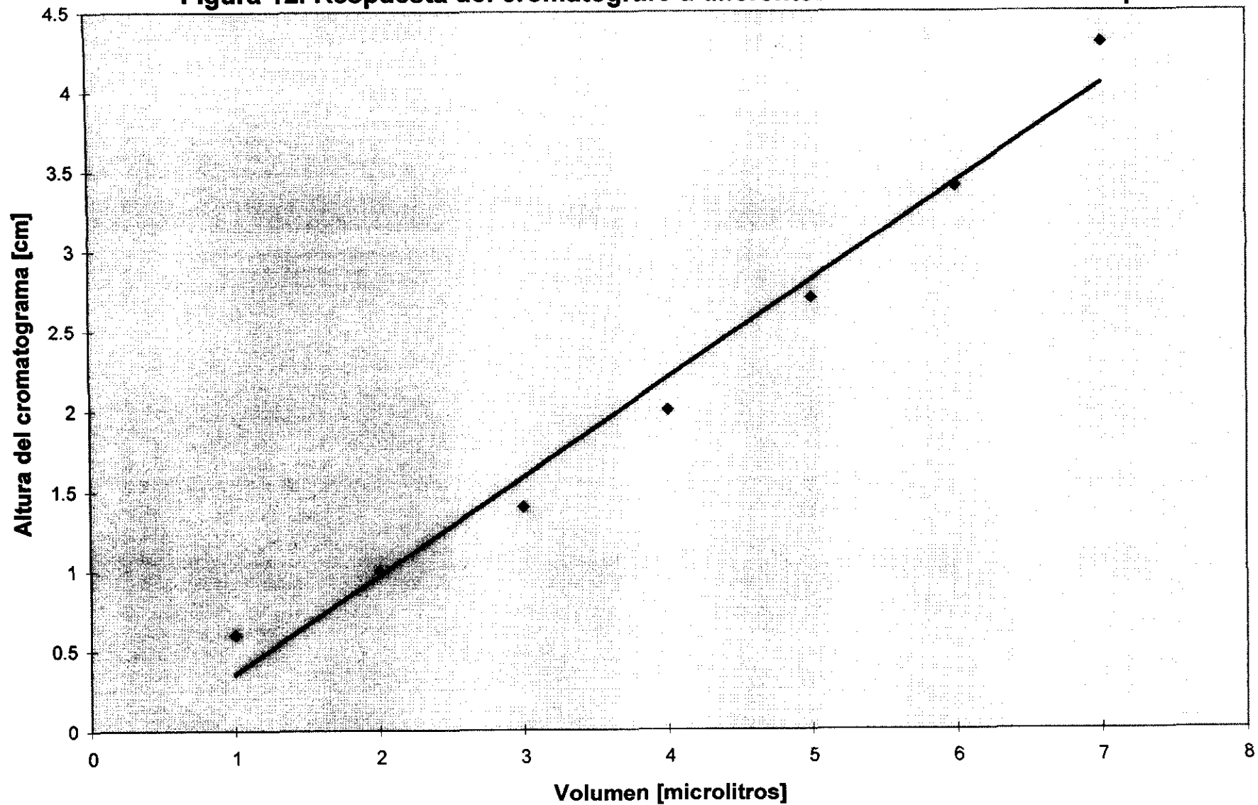
Figura 12. Respuesta del cromatógrafo a diferentes cantidades de metano puro
