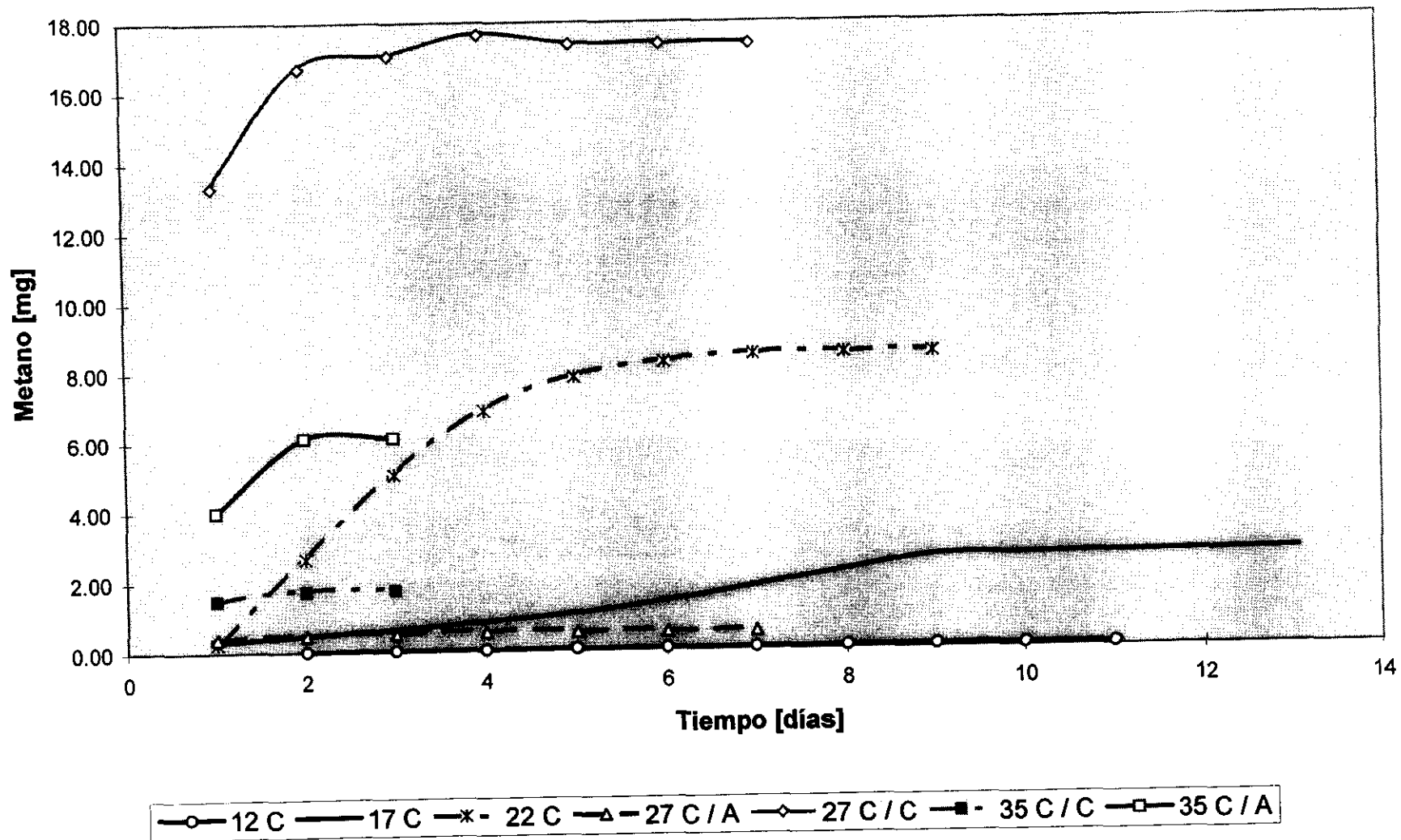
Figura 33. Metano emitido por excretas de bovino de engorda, en producción intensiva, con secado a varias temperaturas.
