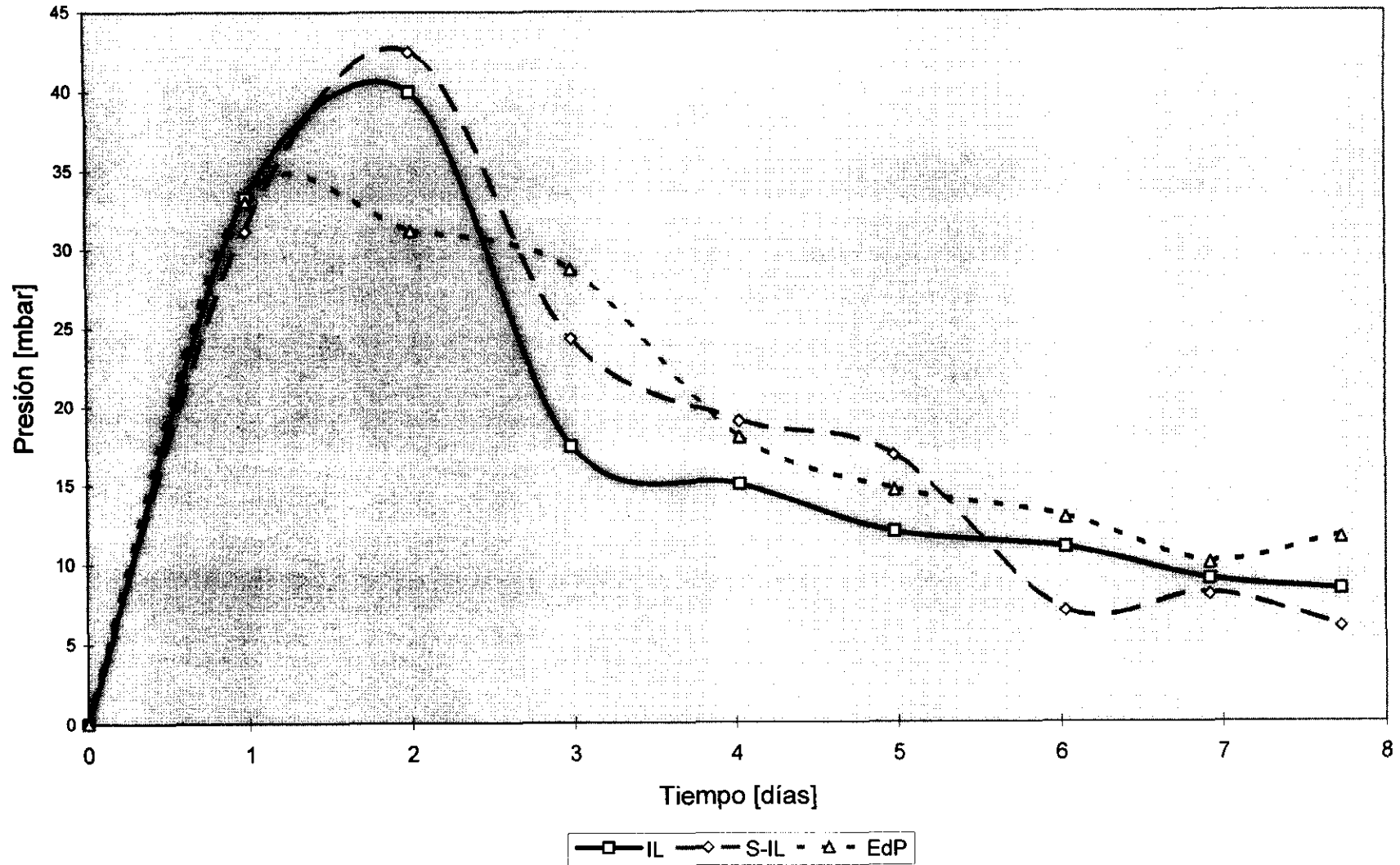
Figura 18. Variación de la presión diaria, con el tiempo de fermentación. 21 C.
