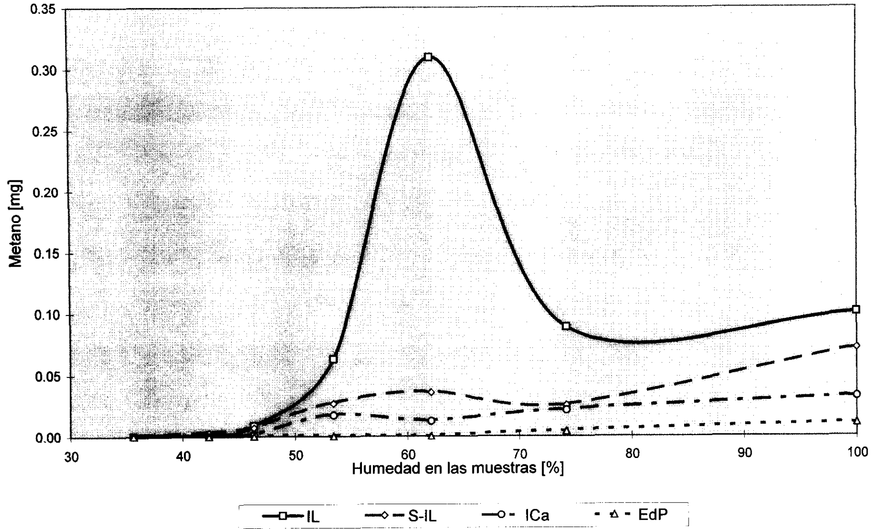
Figura 21. Emisiones diarias de metano como función de la humedad. 12 C.
