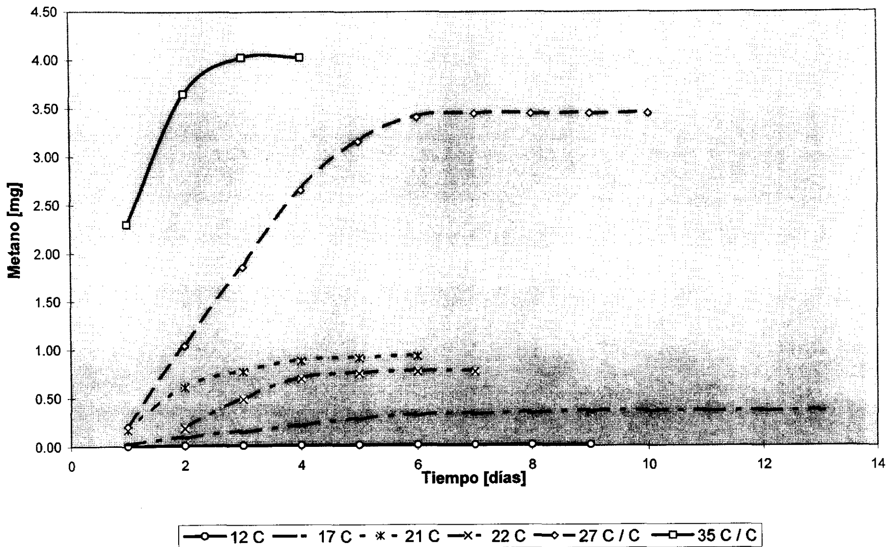
Figura 34. Metano emitido por excretas de bovino de doble propósito en pastoreo, con secado a varias temperaturas.
