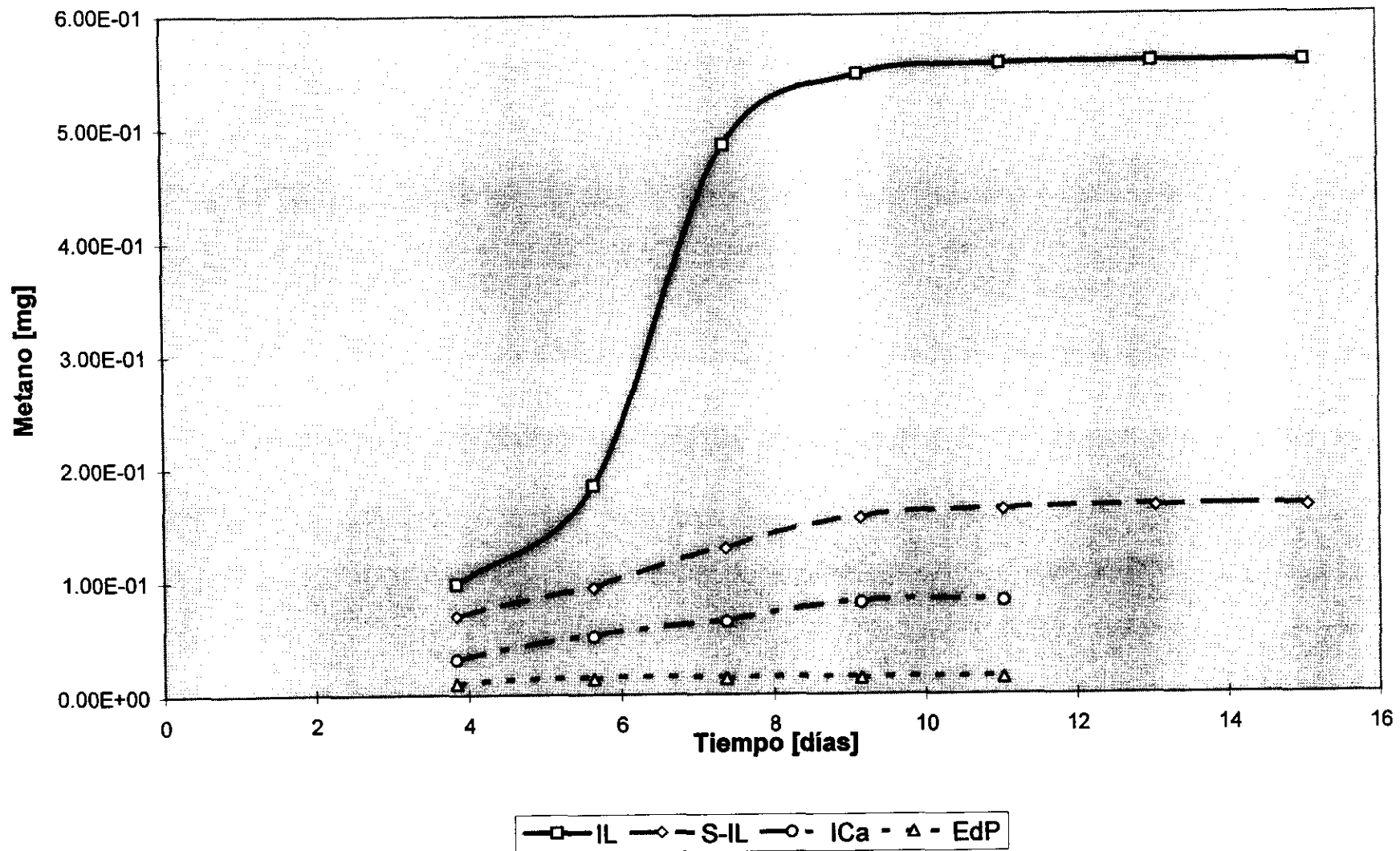
Figura 24. Emisiones de metano por muestras de excretas, como función del tiempo, a 12 C.
