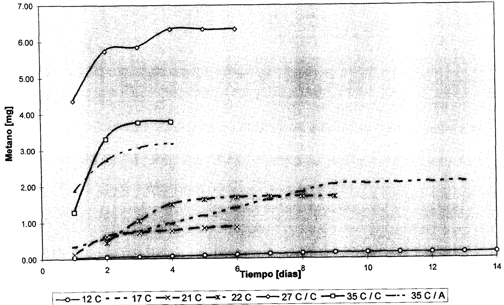
Figura 32. Metano emitido por excretas de bovino lechero semi-estabulado, con secado a varias temperaturas.
