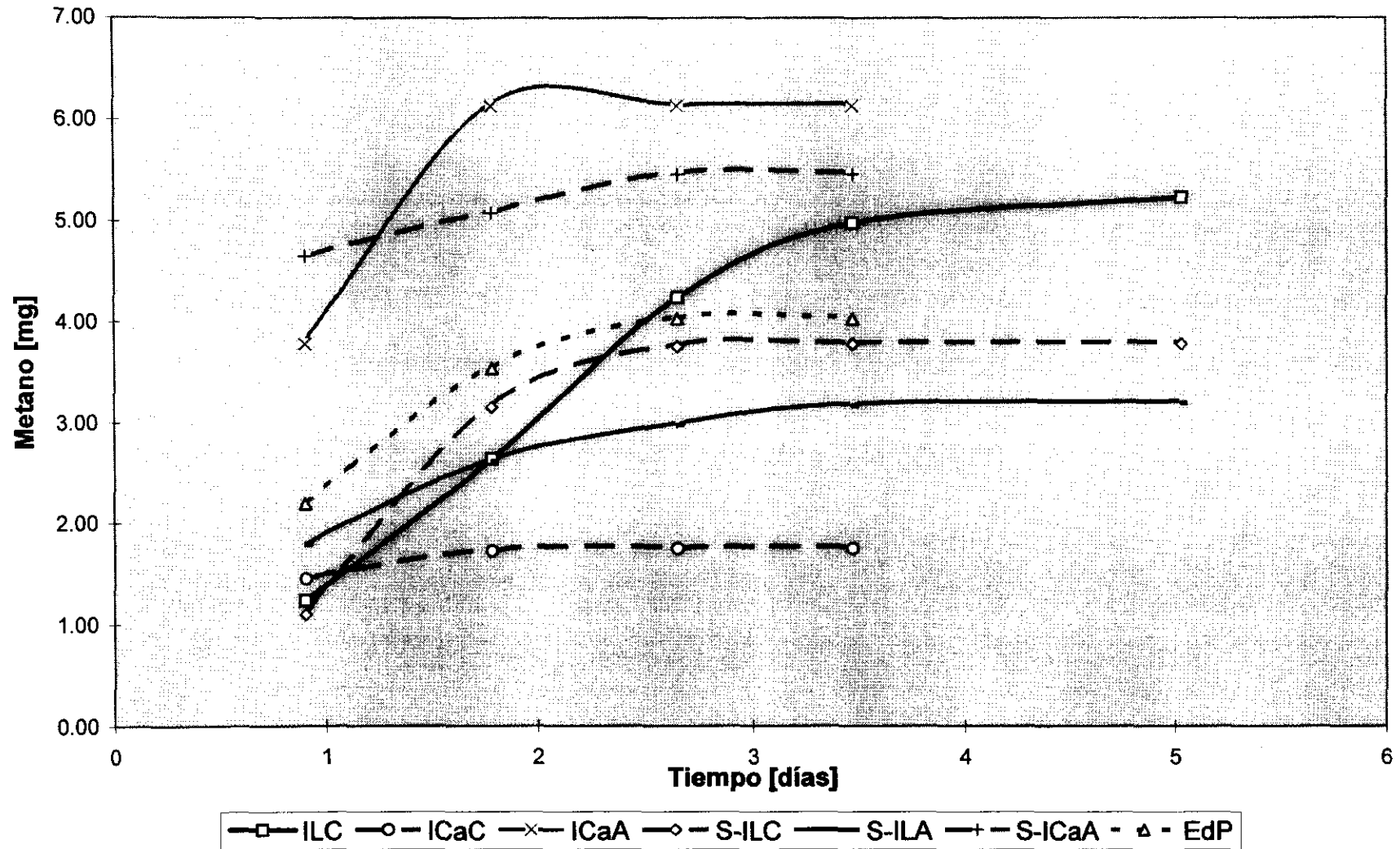
Figura 29. Emisiones de metano por muestras de excretas, como función del tiempo, a 35 C.
