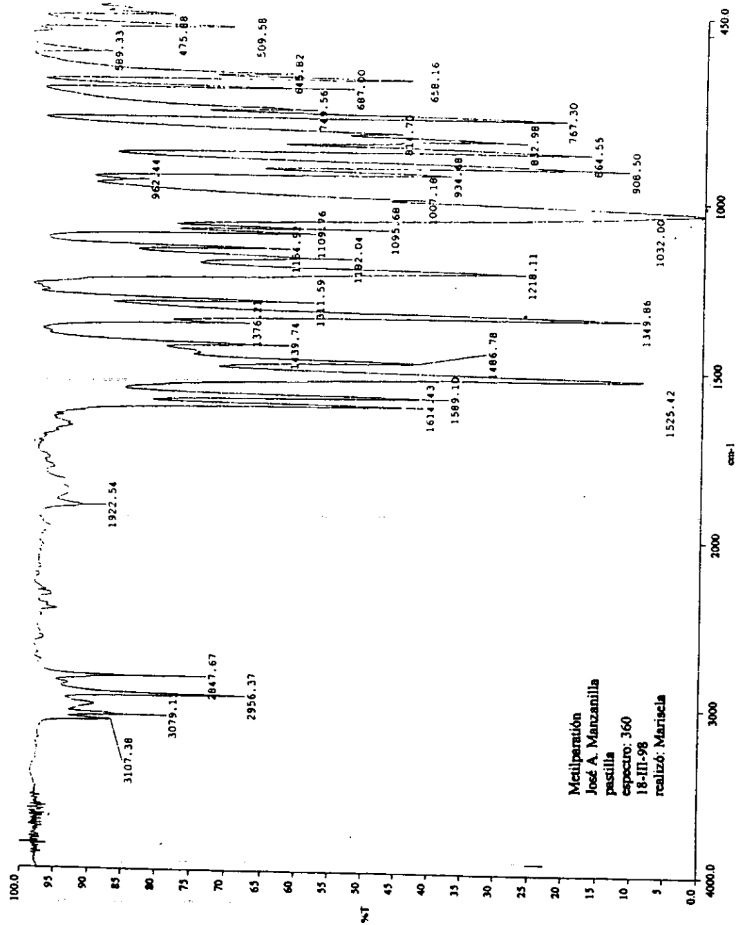
Espectro en el infrarrojo del mentiparación
