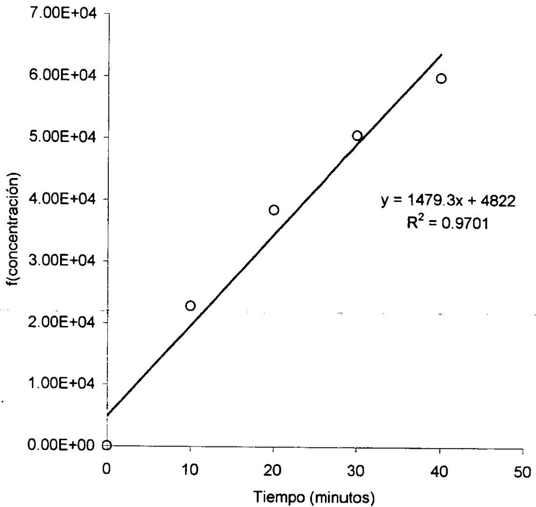
Figura II.8 Modelo matemático de segundo orden del método integral [f(\text{concentración}) = kt] , aplicado a la cinética del metilparatión a pH 12 y 30°C.
