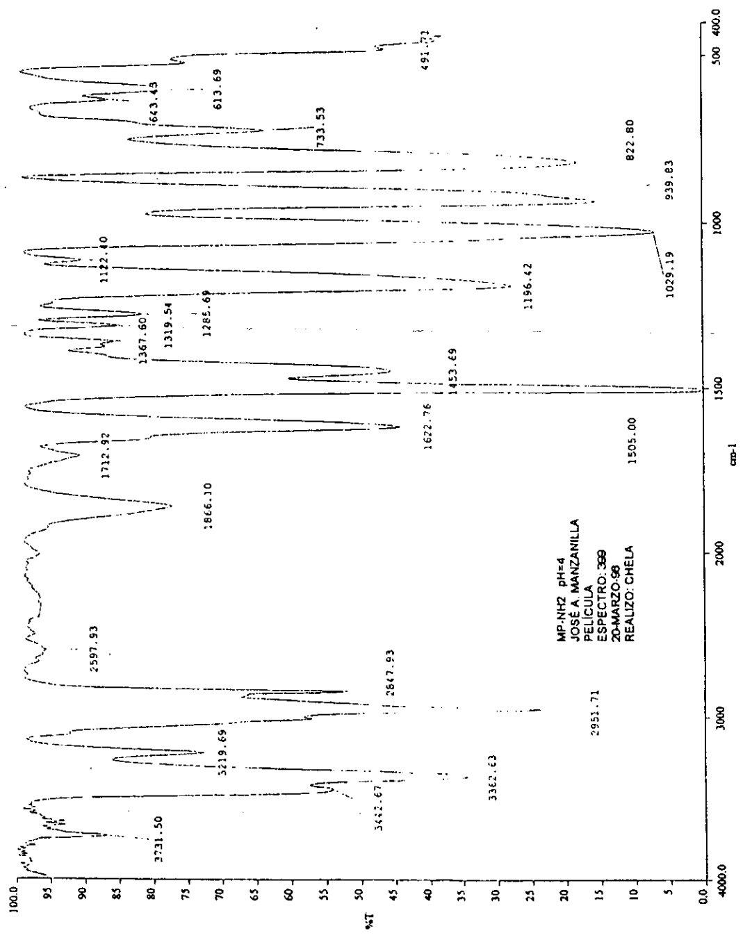
Figura III.15 Espectro en el infrarrojo del derivado amino del metilparatión
