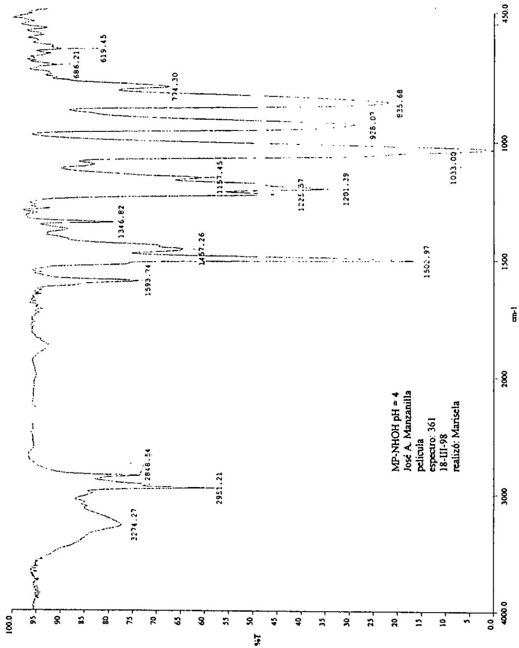
Figura III.16 Espectro en el infrarrojo del derivado hidroxilamino del metilparatión
