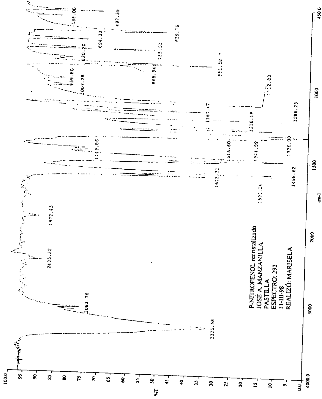
Espectro en el infrarrojo del paranitrofenol
