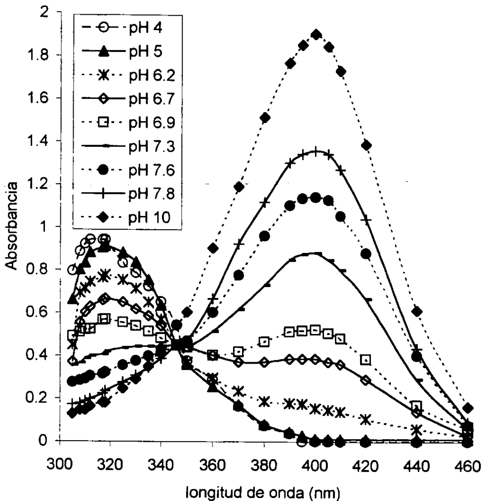
Figura II.1 Espectros de absorción del paranitrofenol (PNF) a diferentes valores de pH en medio acuoso amortiguado. [PNF] = 1 \times 10^{-4} mol/L
