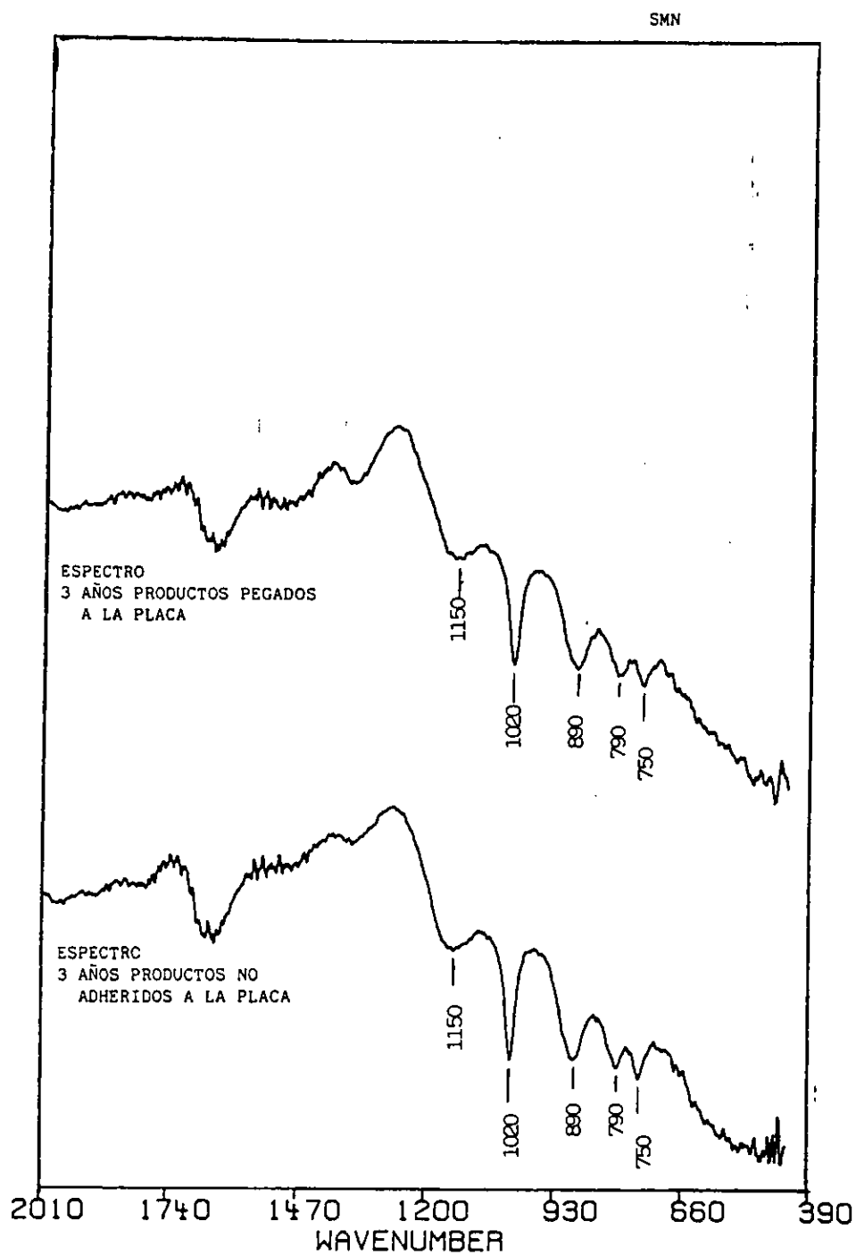
Figura 17 la goetita a tres años de exposición se presenta más crecida en sus dos bandas. Véase tabla 32.
