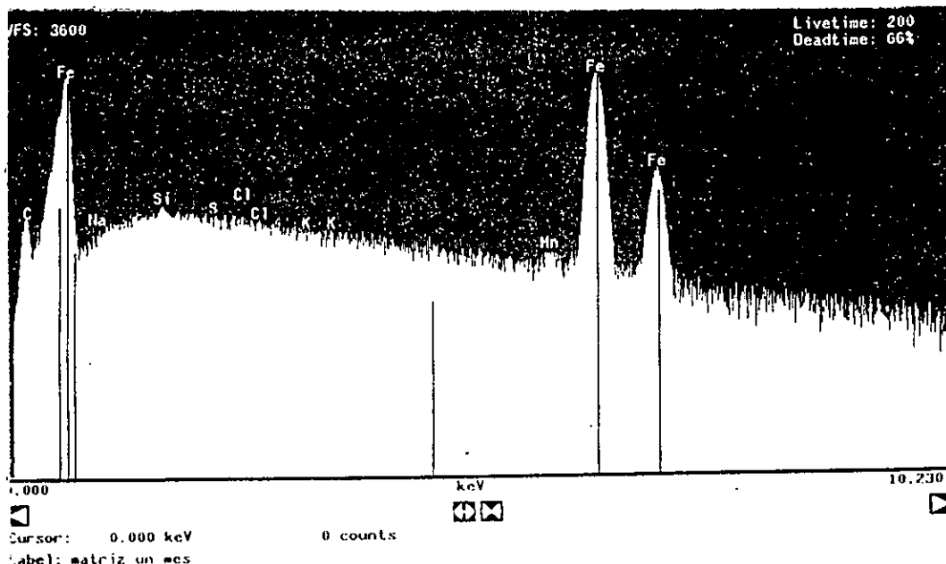
Figura 10e el espectro de EDS con la microsonda se da en escala logarítmica para mostrar más amplia la cantidad de cada elemento detectado, la probeta se expuso un mes a la atmósfera el punto 1 de la foto 10a no muestra oxidación, ni el espectro muestra oxígeno ni azufre.
