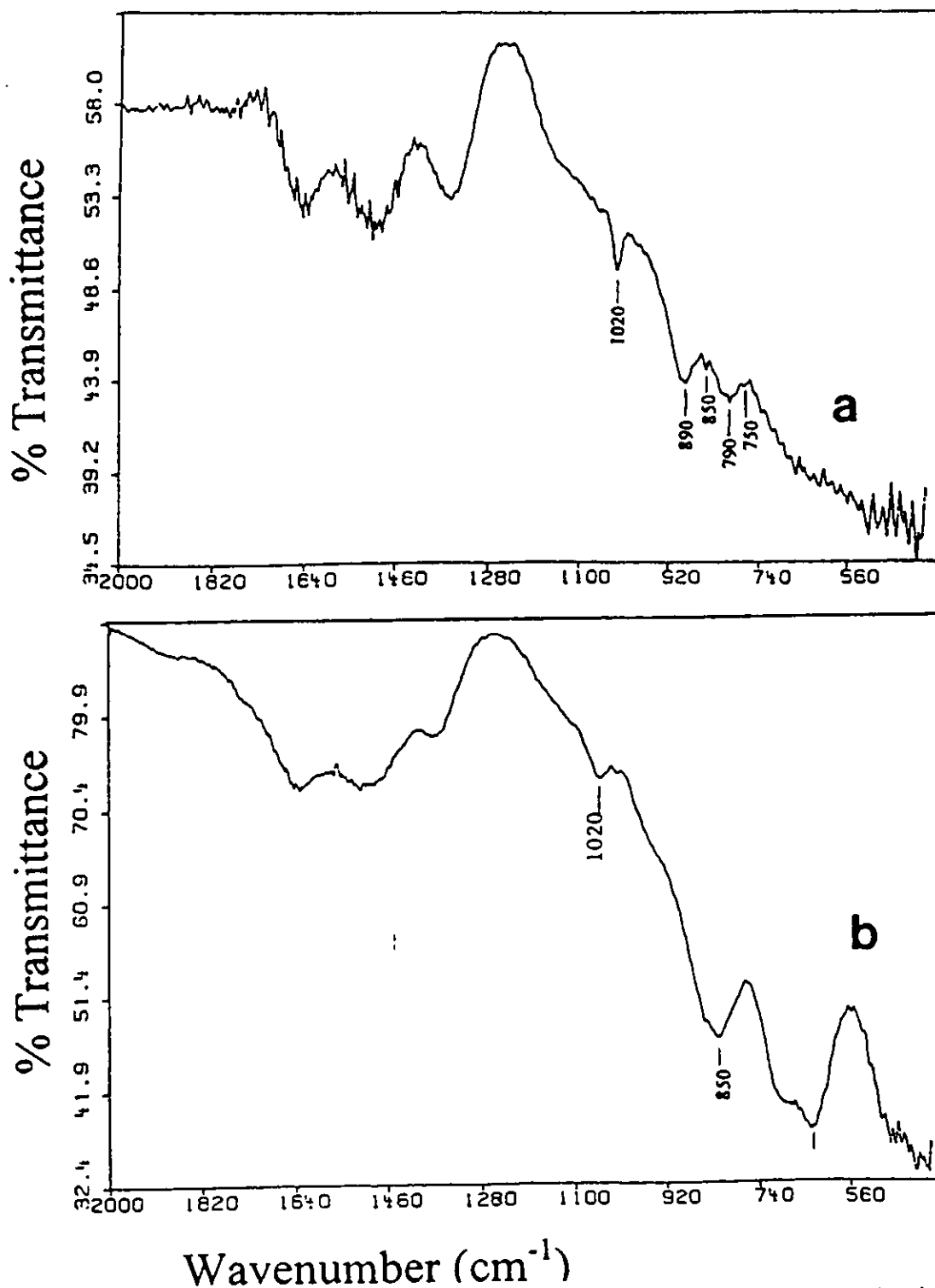
Figura 29(a) el espectro de la parte de arriba de la costra de óxidos de la placa expuesta en Veracruz (IIUV) por 1 año, se presentan las fases de lepidocrocita en 1020, la goetita en 890 y 790; y la akaganeita en la banda de 850. En la fig. 29(b) en el interior de la costra, se nota en el espectro que la fase predominante es la akaganeita en la banda de 850 y la magnetita alrededor de 630.
