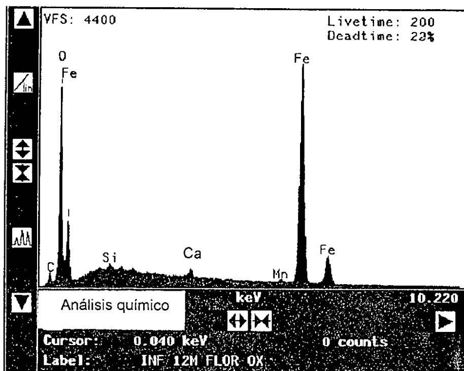
Figura 28f muestra una posible secuencia de oxidación de forma de picadura tipo flor, nótese la diferencia en oxidación con respecto a la figura 28c. Probeta expuesta 12 meses.
