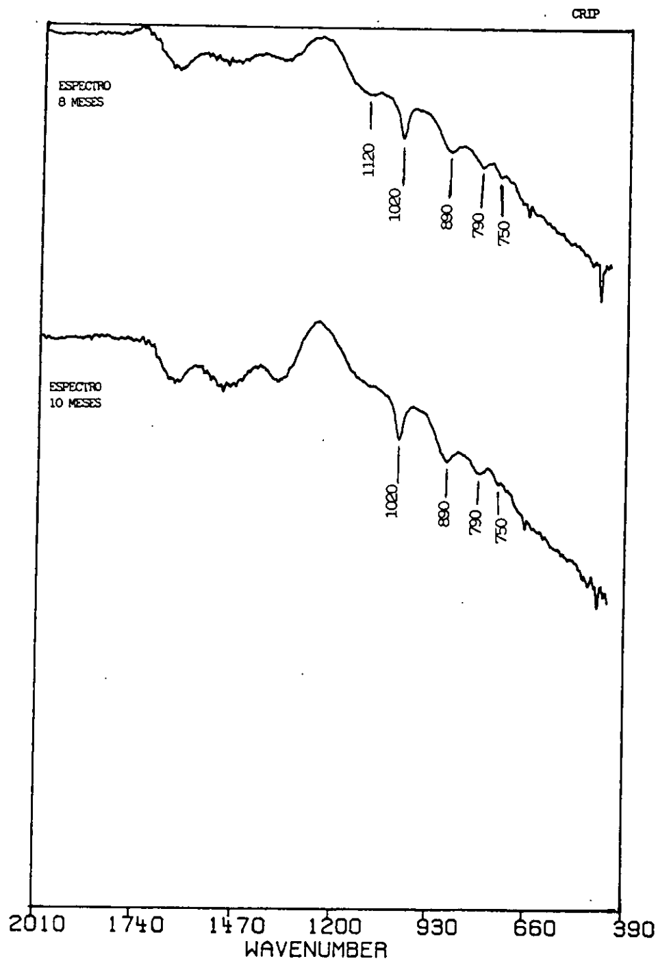
Figura 19 en el espectro de 8 meses la banda de 1120\text{ cm}^{-1} es más tenue que a siete meses. En el espectro de 10 meses se atenúa la banda de 1120.
