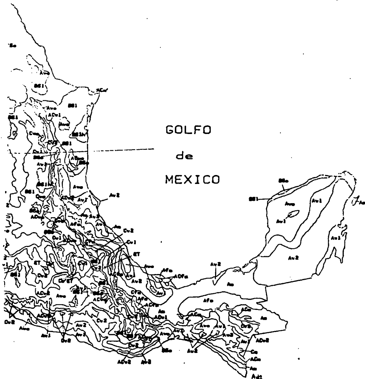
Figura 35 García introduce cambios en las asignaciones del clima para la península de Yucatán, parte del litoral del Golfo de México y parte del litoral del lado del Atlántico.
