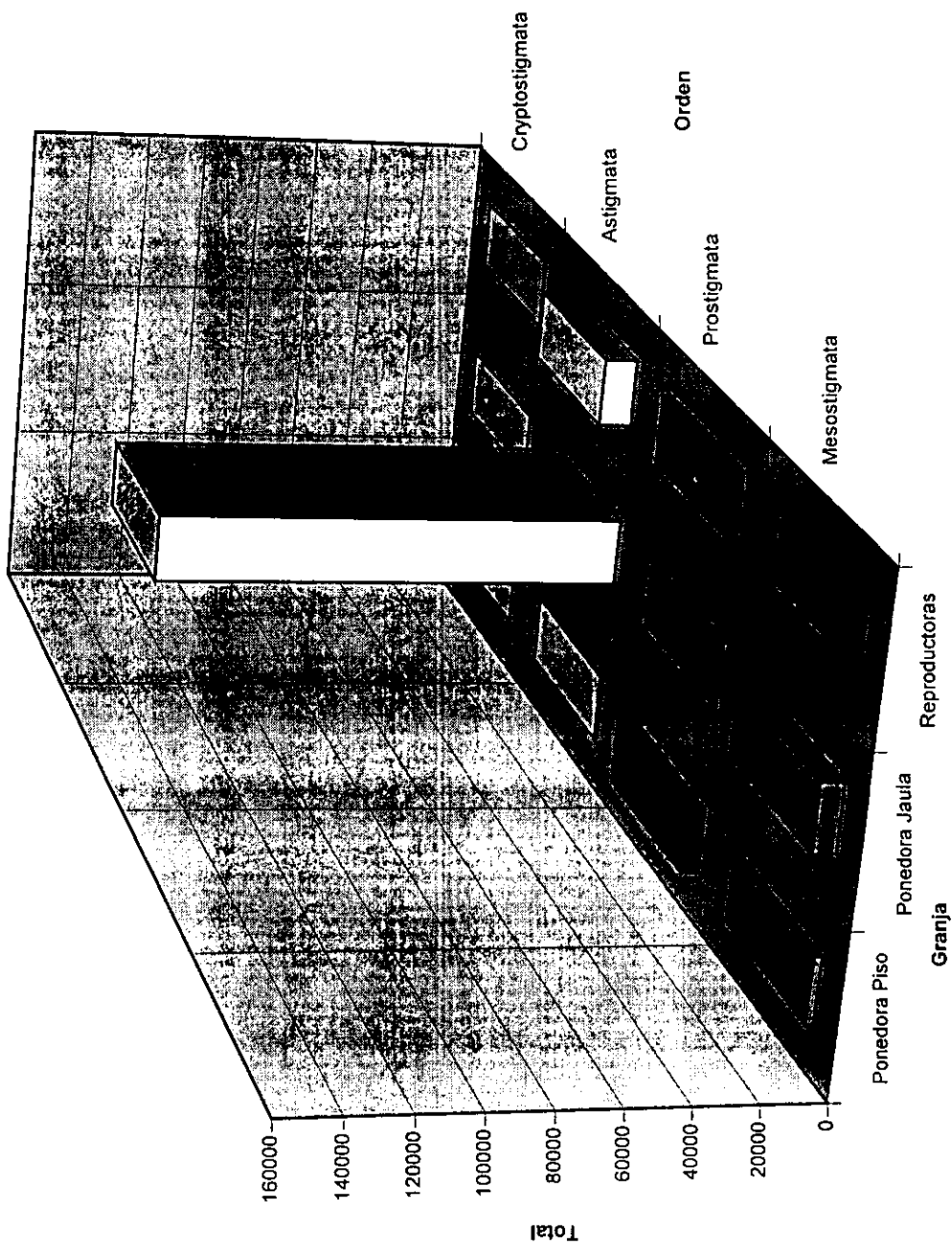
Figura 1. Totales de ácaros por orden, observados en cada tipo de granja. (Rango de ácaros de 0 a 150,634)
