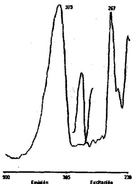
Figura 13. Espectro de emisión y excitación del criseno, obtenido por barrido. Longitudes de onda óptimas.
