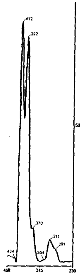
Figura 19. Espectro por síncronos de una mezcla de PAHs.
