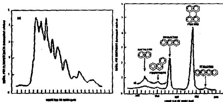
Figura 6. (a) Espectro de fluorescencia de una mezcla de naftaleno, fenantreno, antraceno, pirileno y tetraceno ( \lambda_{exc}=258 nm), (b) Señal por sincronos de la misma muestra ( \Delta\lambda=3 nm). Tomado de Futoma et al, 1981.
