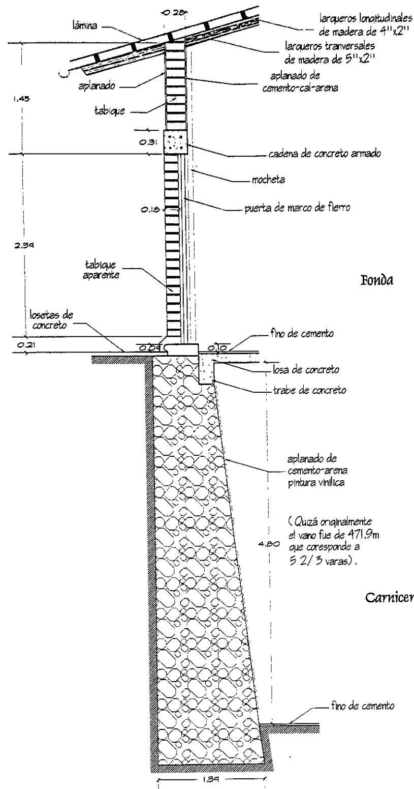
Corte por Fachada bb' Fachada Sur. Antiguas Casas Reales. Levantamiento.
