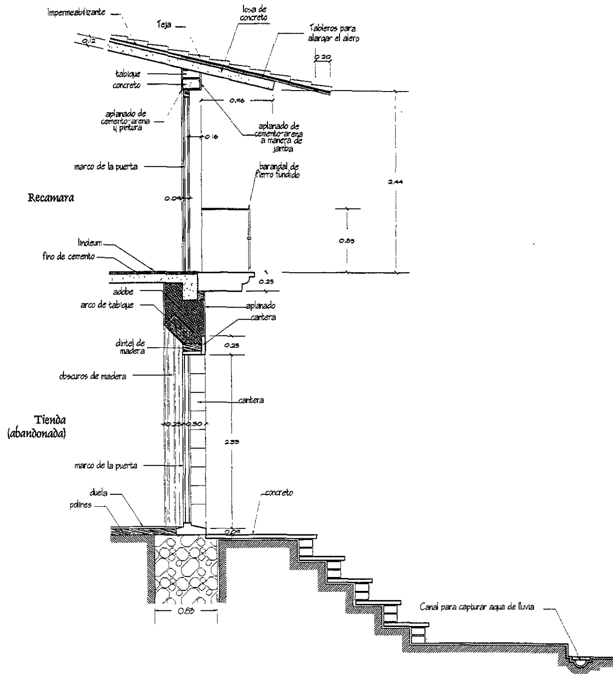
Corte por fachada ee' fachada Nororiente. Ex alcaidia. Casa de la Familia Galindo. Restauración
