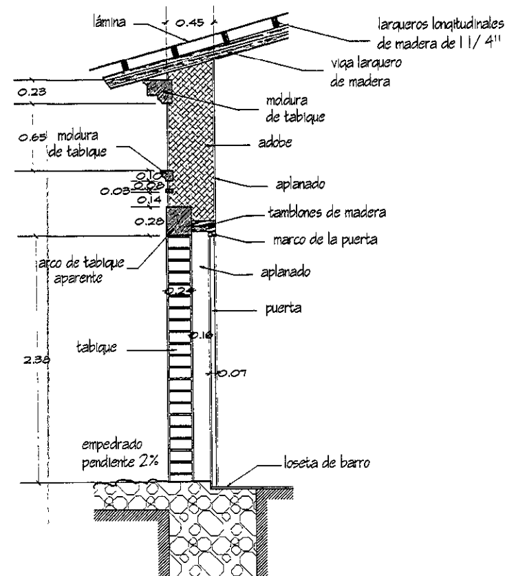
Corte por Fachada aa' Fachada Sur. Levantamiento.
