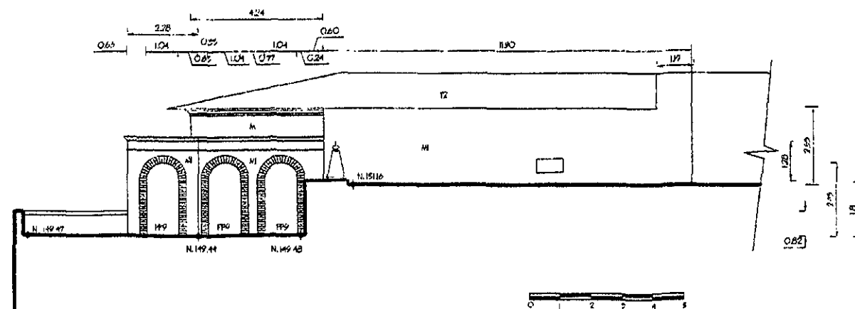
Fachada Sur (Antiguas Cajas Reales) Levantamiento de tipologías y materiales
