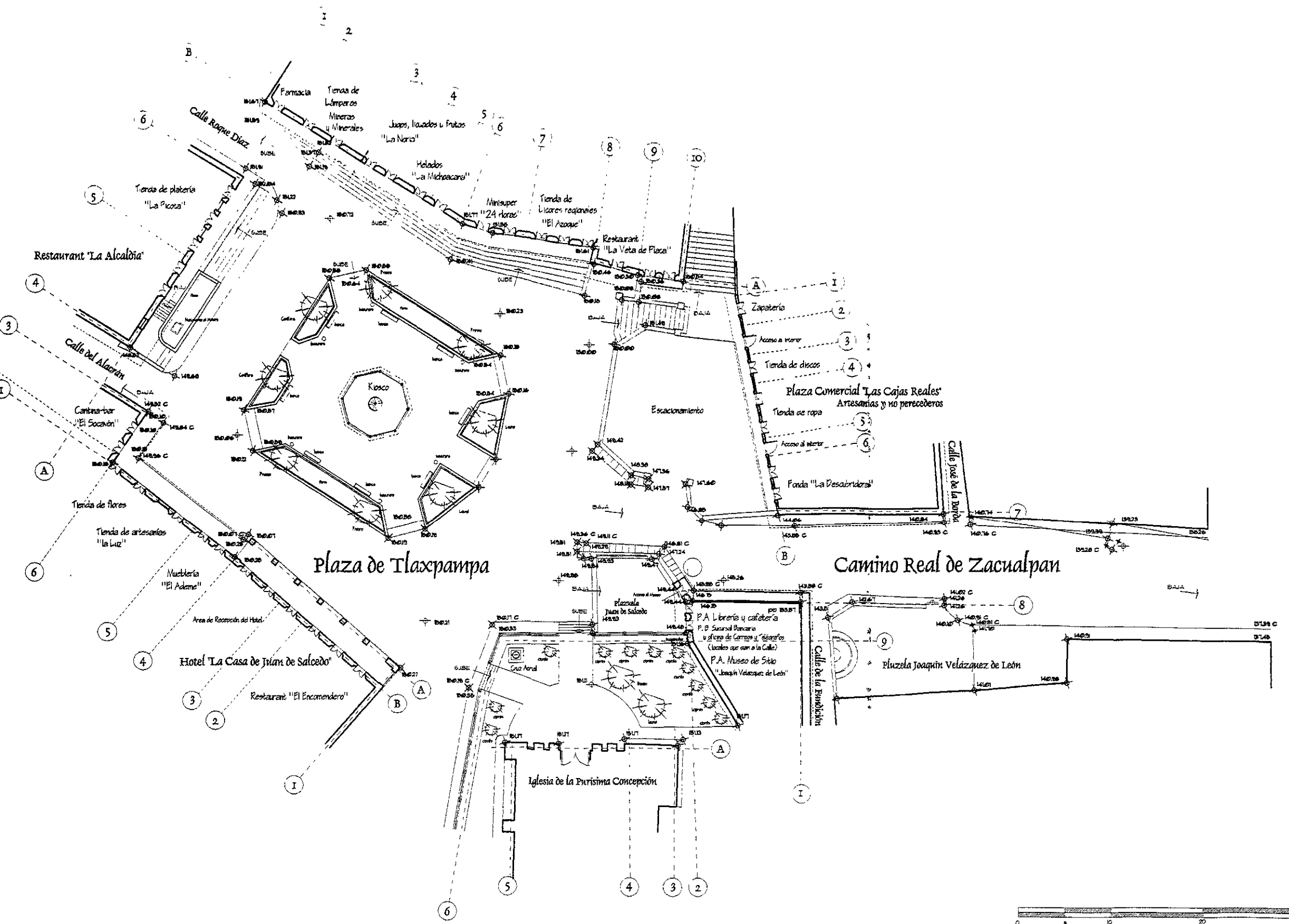
Planta Arquitectónica de Conjunto de la Plaza Proyecto de Restauración
