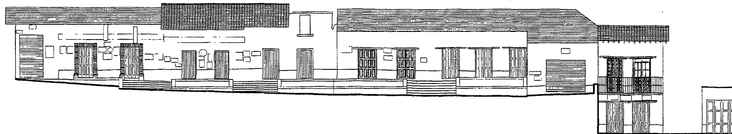
Fachada Oriente Estado actual
