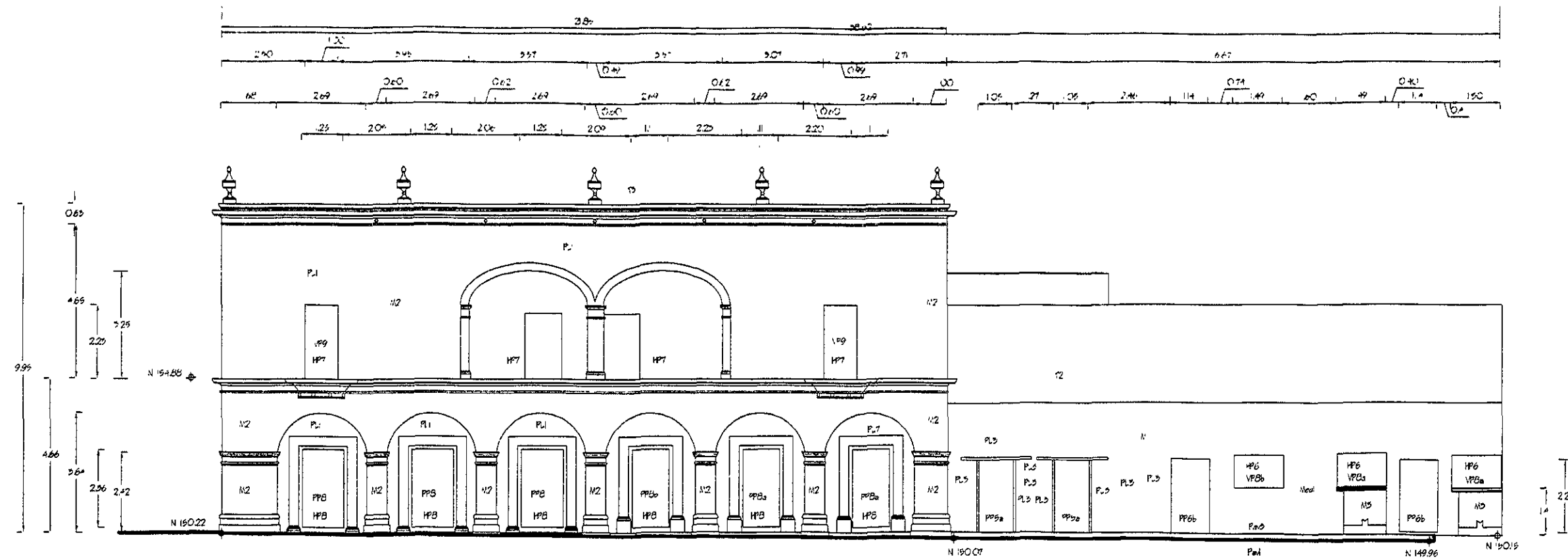
Fachada Norponiente (Casa de Juan de Salcedo) Levantamiento de Tipologías y Materiales
