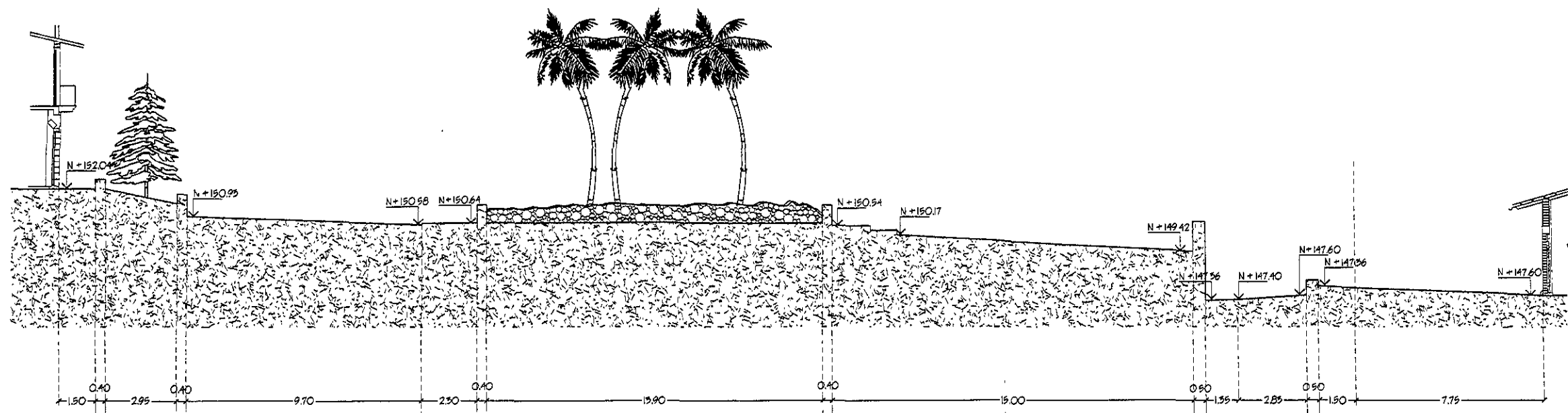
Corte AA' Levantamiento: estado actual
