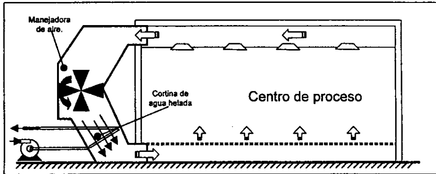
Figura 2.8. Diagrama básico de operación de un sistema de doble ciclo.
