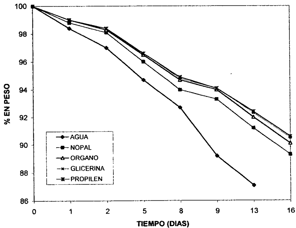
Gráfico 2. Capacidad de captación de agua a 31% de humedad relativa en función del tiempo. Soluciones al 1%, considerando una cantidad inicial de agua de 100%.
