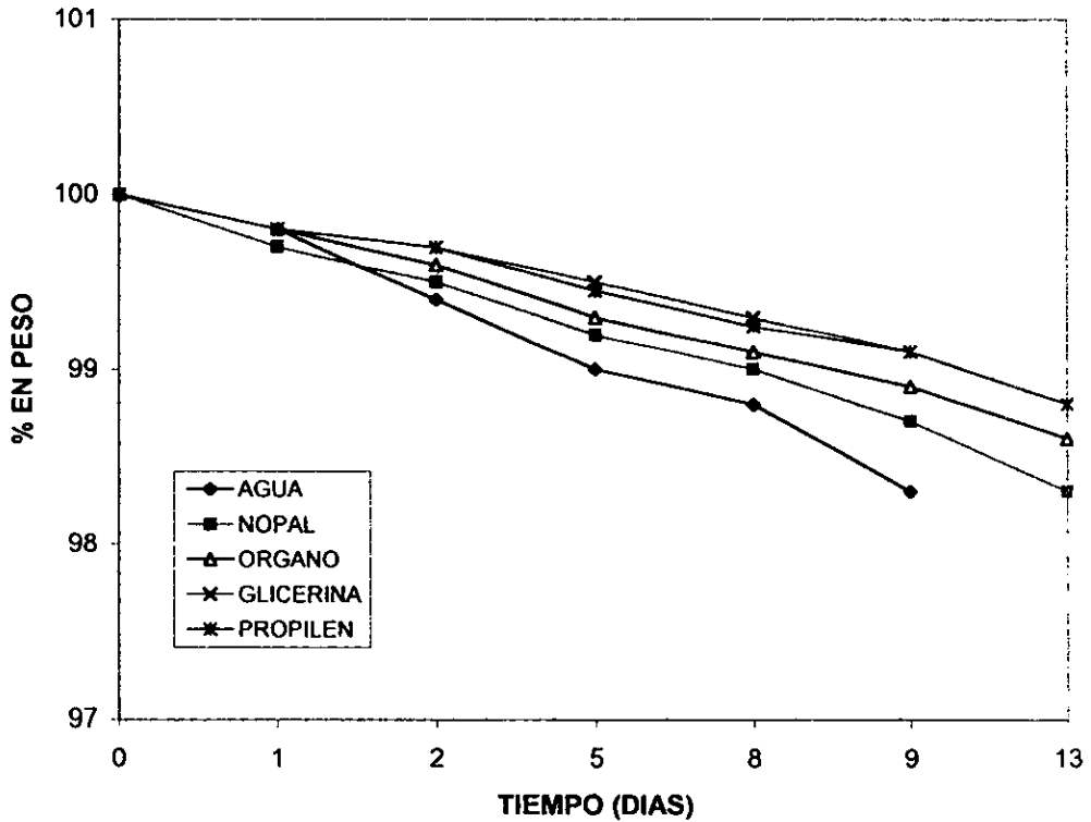
Gráfico 4. Capacidad de captación de agua a 86% de humedad relativa en función del tiempo. Soluciones al 1%, considerando una cantidad inicial de agua de 100%.
